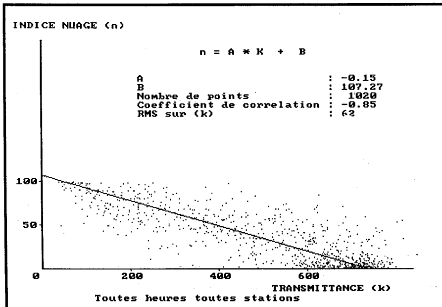
Figure 4.29 : L'indice d'ennuage (n) en fonction de la transmittance globale de l'atmosphère (K) pour les hauteurs du soleil comprises entre 43° et 47° pour l'année 1984.
