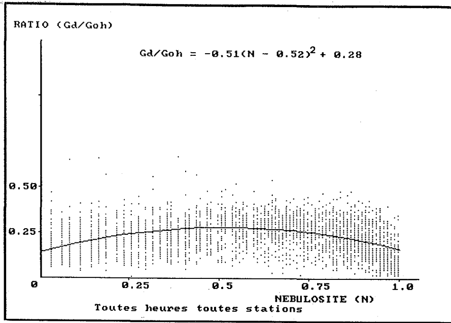
Figure [6.32] : G_d/G_{oh} en fonction de la nébulosité totale ( N ) pour les hauteurs du soleil comprises entre 12^\circ et 65^\circ (année 1985).
