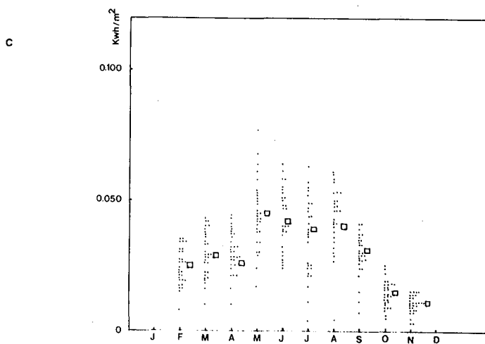
Figure 4.3 : L'erreur quadratique moyenne (rms en kWh/m 2 ) par mois pour l'année 1984. a) 9-10 h TU ; b) 12-13 h TU ; c) 15-16 h TU.
