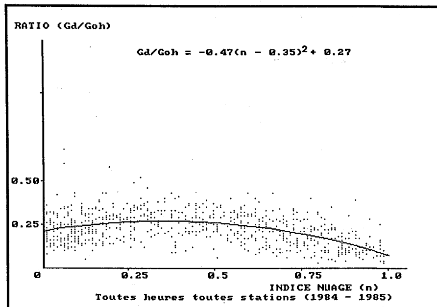
Figure [6.45] : Gd/Goh en fonction de l'indice d'ennuage (n) pour les hauteurs du soleil comprises entre 23° et 27° (années 1984 - 1985).
