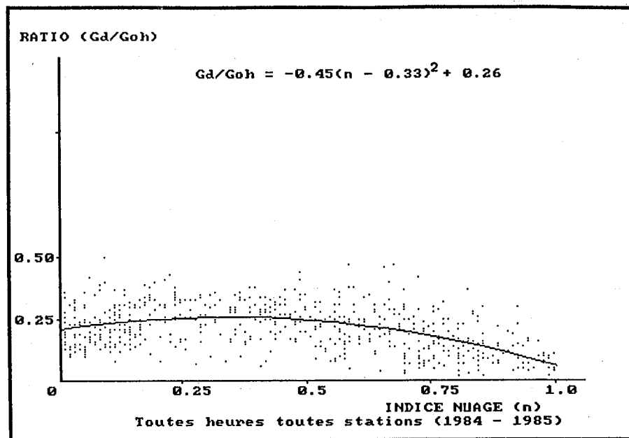
Figure [6.44] : Gd/Goh en fonction de l'indice d'ennuage (n) pour les hauteurs du soleil comprises entre 18° et 22° (années 1984 - 1985).
