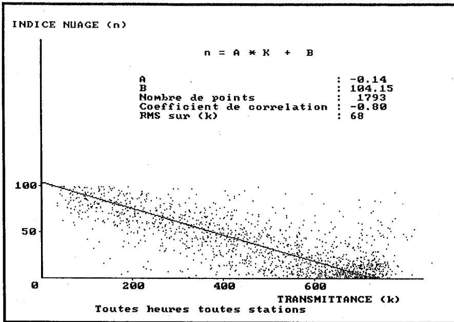
Figure 4.28 : L'indice d'ennuage (n) en fonction de la transmittance globale de l'atmosphère (K) pour les hauteurs du soleil comprises entre 38° et 42° pour l'année 1984.
