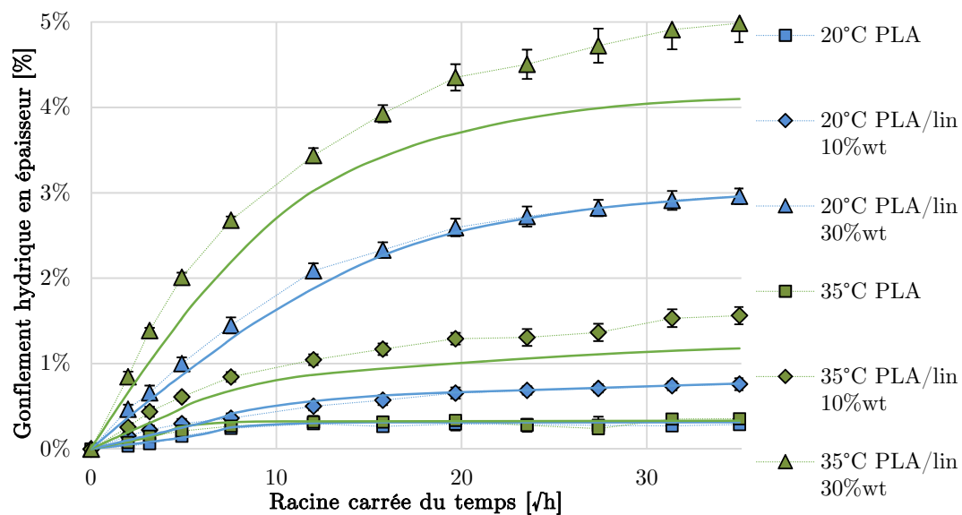
FIGURE 10.8 – Valeurs expérimentales et modélisées de gonflement hydrique du PLA et des composites PLA/lin dans le sens de l'épaisseur ( z ) au cours du vieillissement en immersion dans l'eau à 20 et 35°C
