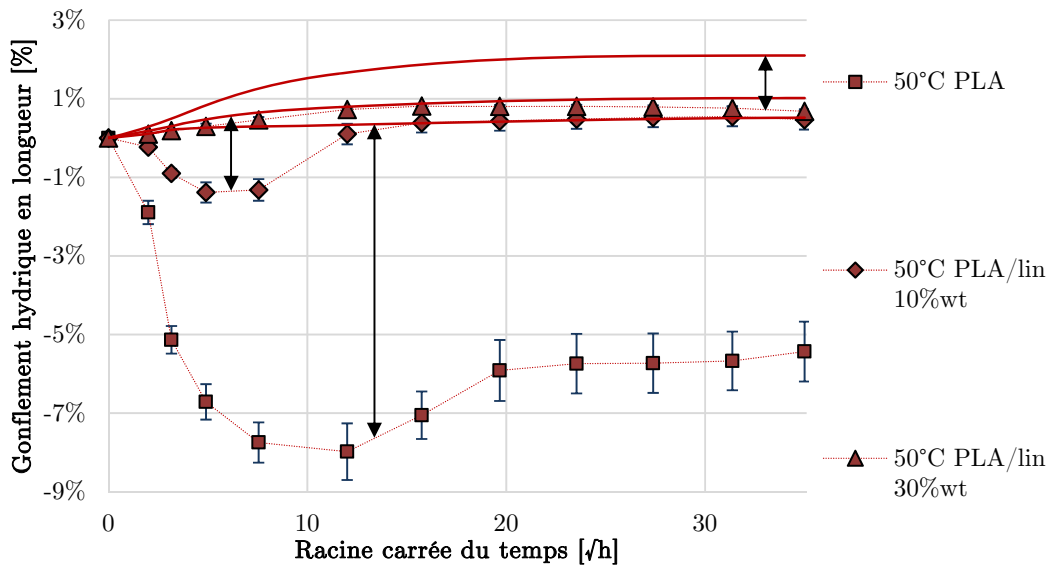
FIGURE 10.13 – Valeurs expérimentales et modélisées de gonflement hydrique du PLA et des composites PLA/lin dans le sens de la longueur ( \bar{x} ) au cours du vieillissement en immersion dans l'eau à 50°C
