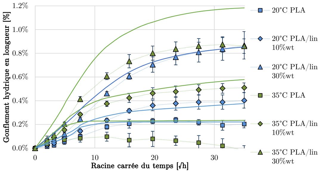
FIGURE 10.10 – Valeurs expérimentales et modélisées de gonflement hydrique du PLA et des composites PLA/lin dans le sens de la longueur ( \bar{x} ) au cours du vieillissement en immersion dans l'eau à 20 et 35°C
