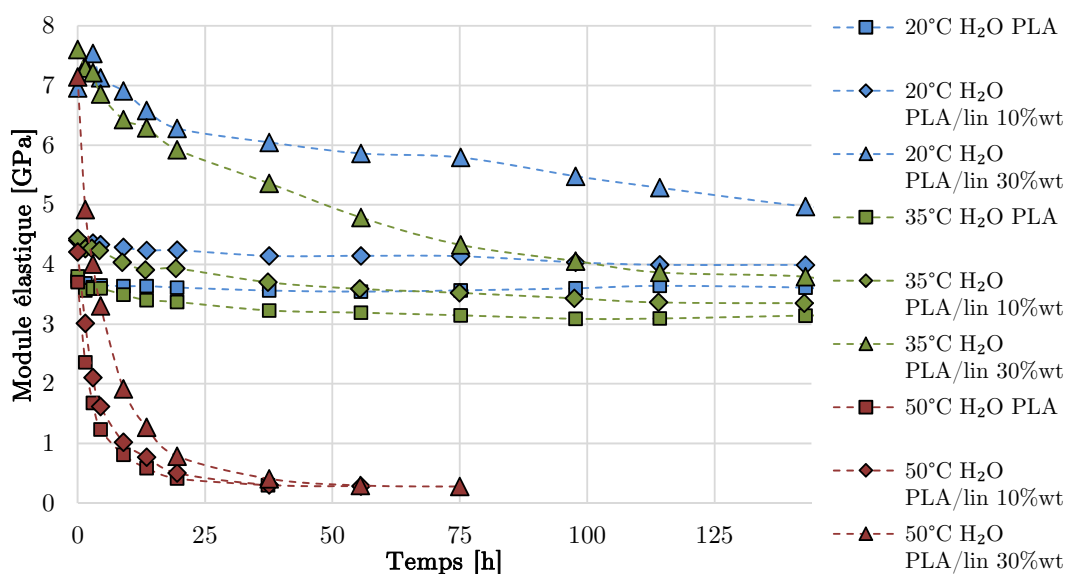
FIGURE 9.5 – Module d'élasticité in situ du PLA et des composites PLA/lin au cours du vieillissement en immersion dans l'eau
