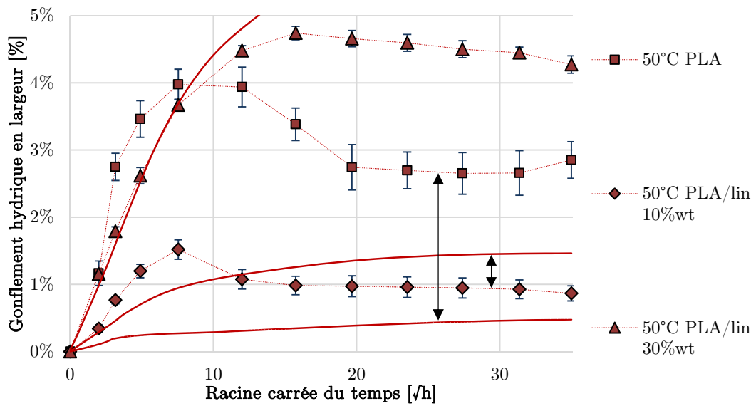
FIGURE 10.12 – Valeurs expérimentales et modélisées de gonflement hydrique du PLA et des composites PLA/lin dans le sens de la largeur ( \bar{y} ) au cours du vieillissement en immersion dans l'eau à 50°C
