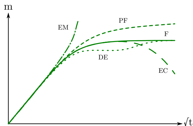
FIGURE 2.5 – Courbes gravimétriques typiques d'absorption d'un fluide [211]; (F) comportement de Fick, (PF) comportement de pseudo-Fick, (DE) diffusion en 2 étapes, (EC) diffusion avec endommagement chimique, (EM) diffusion avec endommagement mécanique
