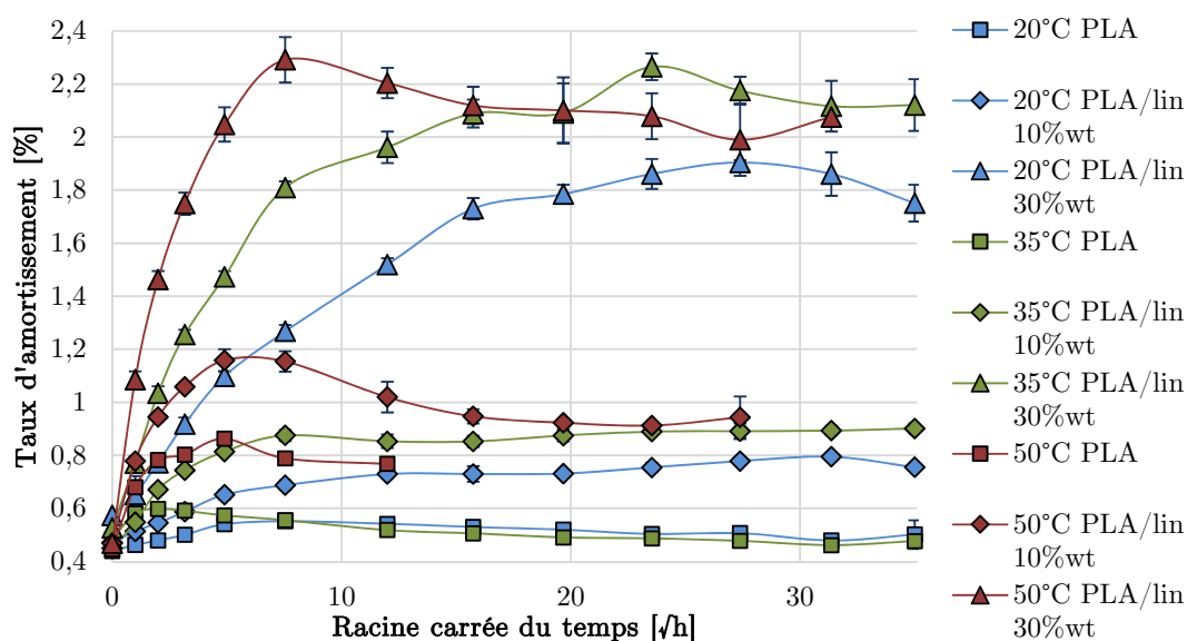
FIGURE 7.23 – Taux d'amortissement ex situ du PLA et des composites PLA/lin au cours du vieillissement en immersion dans l'eau
