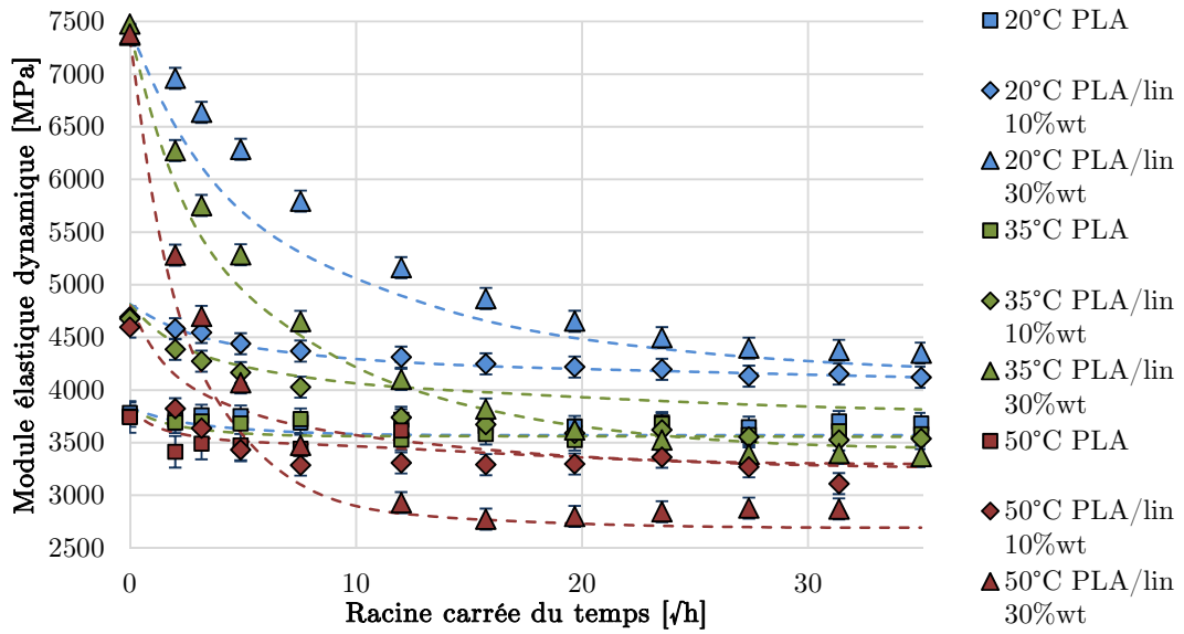
FIGURE 10.16 – Valeurs expérimentales du module d'élasticité et valeurs modélisées du module homogène équivalent en flexion (tirets) du PLA et des composites PLA/lin au cours du vieillissement en immersion dans l'eau
