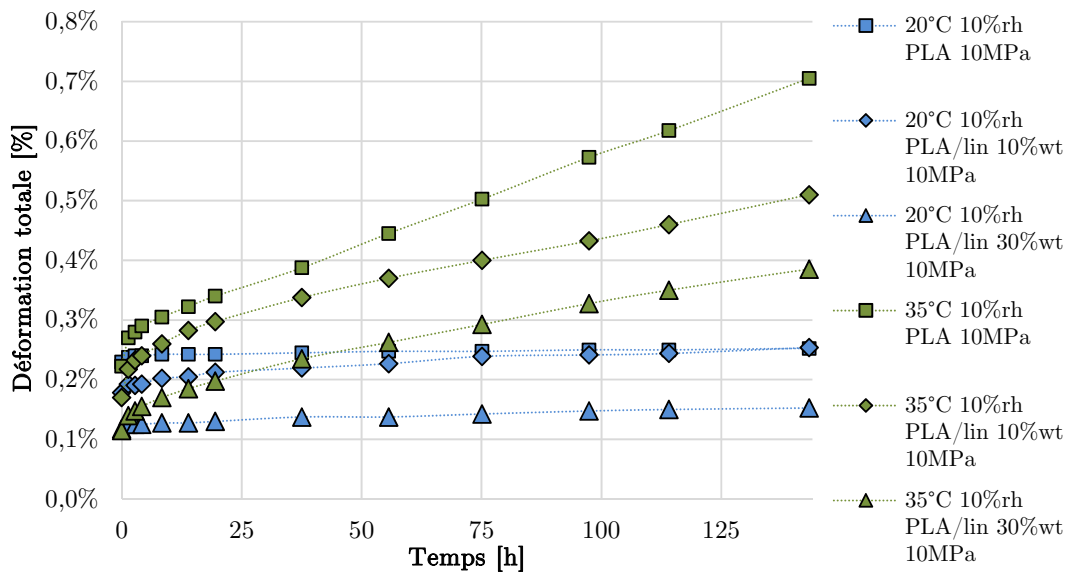
FIGURE 9.3 – Déformation totale du PLA et des composites PLA/lin au cours du fluage à 10 MPa en atmosphère sèche (10%hr)
