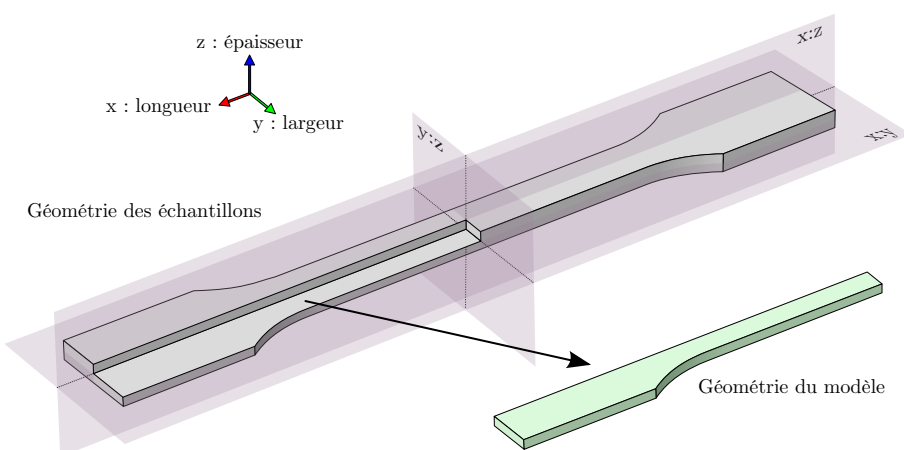
FIGURE 10.2 – Géométrie du modèle utilisé
