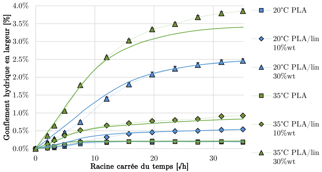
FIGURE 10.9 – Valeurs expérimentales et modélisées de gonflement hydrique du PLA et des composites PLA/lin dans le sens de la largeur ( \bar{y} ) au cours du vieillissement en immersion dans l'eau à 20 et 35°C
