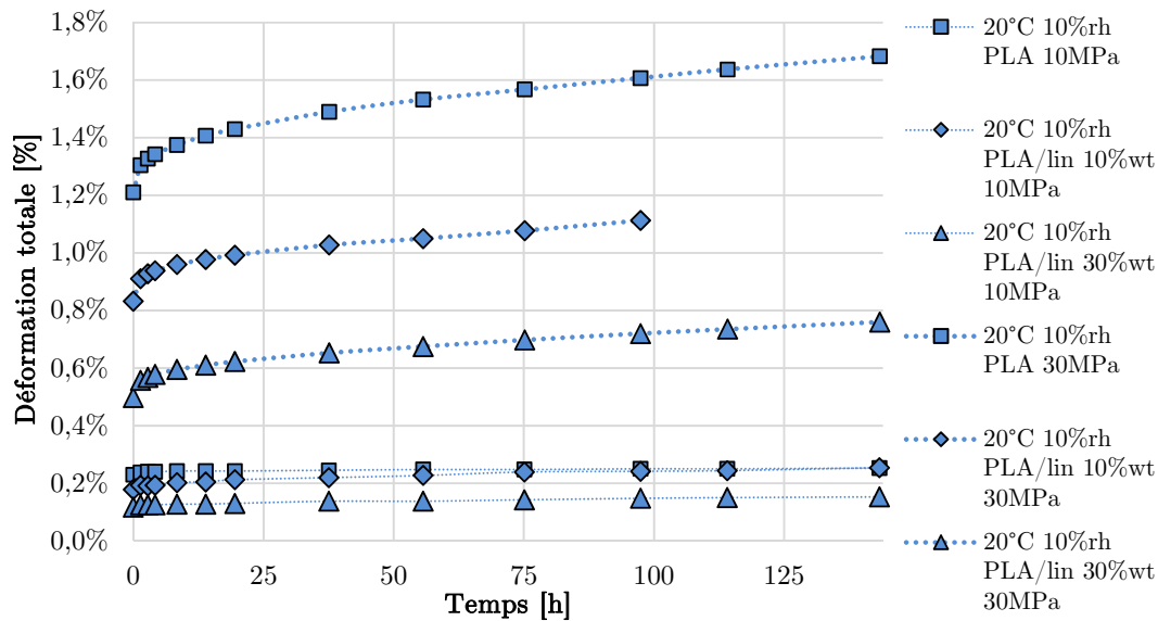
FIGURE 9.1 – Déformation totale du PLA et des composites PLA/lin au cours du fluage en atmosphère sèche à 20°C (10%rh)
