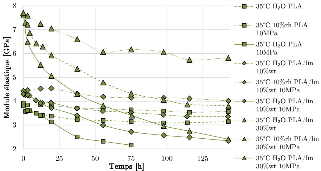
FIGURE 9.11 – Module d'élasticité du PLA et des composites PLA/lin au cours du fluage à 10 MPa en immersion dans l'eau à 35°C
