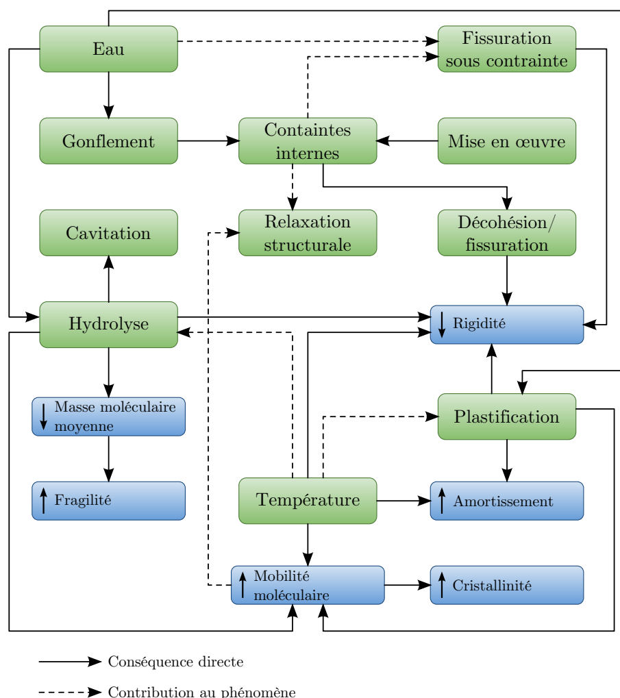
FIGURE 7.27 – Interdépendances des mécanismes de vieillissement impliqués lors de l'exposition des composites PLA/lin à un milieu thermo-hydrigue
