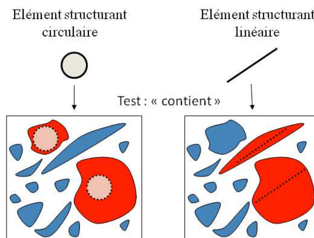
FIGURE D.3 – Éléments structurants : Influence de l'élément structurant choisi (circulaire ou linéaire) sur le résultat d'une transformation morphologique simple (inclusion).
