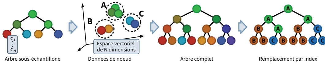
Figure 9 : Vue d'ensemble. A partir d'un sous-échantillonnage de la scène, un arbre PBGI réduit est construit. Les fonctions sphériques des noeuds sont groupées en fonction de leur distance dans l'espace vectoriel de la représentation des fonctions sphériques. Le centre de chaque groupe est le représentant de son groupe. Les représentants forment une table de correspondances avec un index. Pour l'arbre complet, les fonctions sphériques des noeuds sont remplacées par les indices de la table de correspondances, réduisant la consommation de mémoire de l'arbre par un facteur entre 3.7 et 5.
