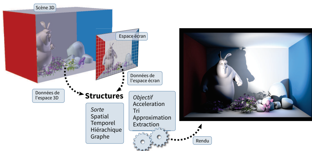
Figure 2 : Les données d'entrée (la scène 3D) sont transformées en structures adaptées à l'algorithme de rendu. Selon cette algorithm, les structures sont de différents types et objectives. L'algorithme se sert des données préparées dans les structures et crée l'image.
