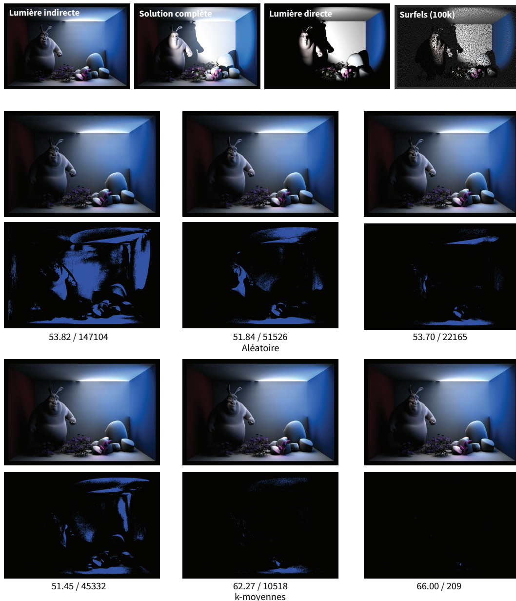
Figure 11 : Résultats et Comparaison. Quelques résultats et la comparaison avec un choix aléatoire de représentants. Nous montrons le nombre de pixels perceptuellement différents (PPD) [Yee04] et le peak signal-to-noise ratio (PSNR) par rapport à la référence (image dénotée "Lumière indirecte") en format <PSNR/PPD> sous chaque résultat. On observe une baisse rapide de PPD et une hausse de PSNR qui sont supérieures à celles du choix aléatoire. En général, les résultats convergent rapidement à un niveau d'erreur peu perceptible.
