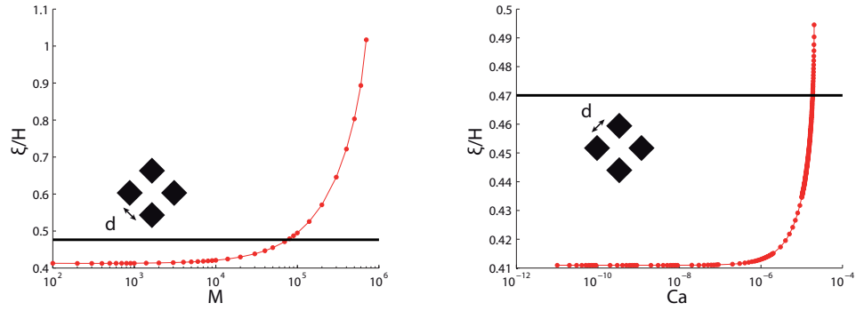
(a) Longueur du ménisque en fonction du rapport de viscosité pour Ca = 10^{-6} .
