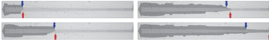
(c) Vue large lors de l'invasion de l'eau en entrée (gauche) et en sortie (droite) montrant une accélération du processus d'invasion dans le poreux. La flèche bleue indique le front d'eau en dehors du poreux et la flèche rouge à l'intérieur du poreux.
