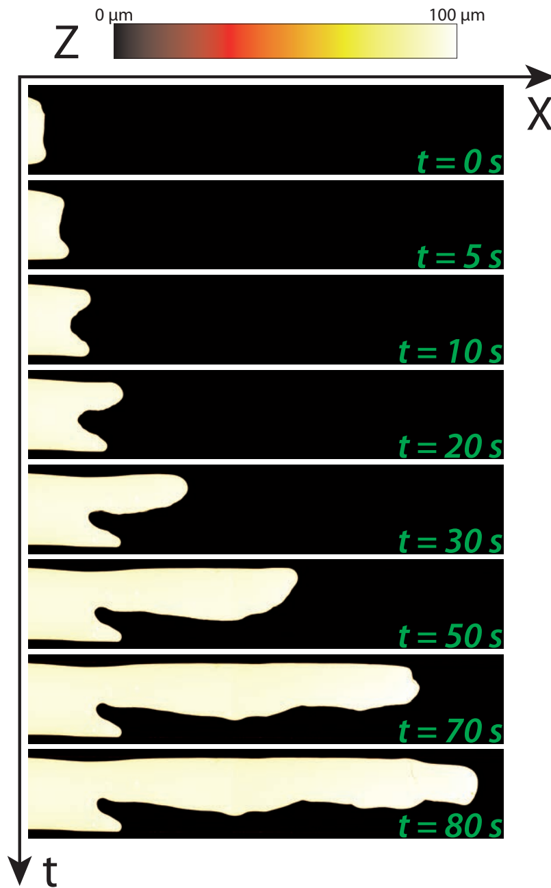
FIGURE 3.2 – Images issues d’une expérience d’invasion en régime de drainage dans une cellule de Hele-Shaw pour Q = 1.5 \mu\text{L}/\text{min} , \theta_e = 120^\circ et M = 1000 . Le niveau de couleur correspond à l’épaisseur d’eau dans le canal. L’eau envahit toute la hauteur du canal.
