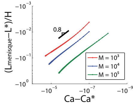
(b) Longueur du ménisque en fonction du nombre capillaire pour différents M . La pente des lois de puissance est identique pour les trois.
