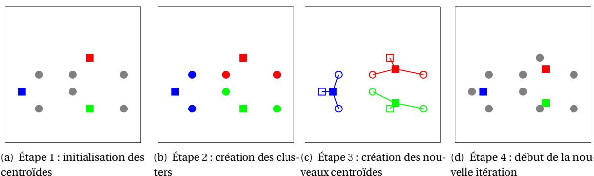
FIGURE 2.1 – Les étapes de l'algorithme du k -means avec k = 3 .
