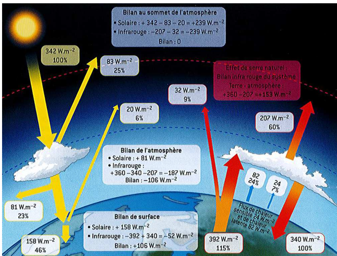
FIGURE 1.1 – Bilan radiatif global de la Terre. Source : Delmas et al. (2007).
