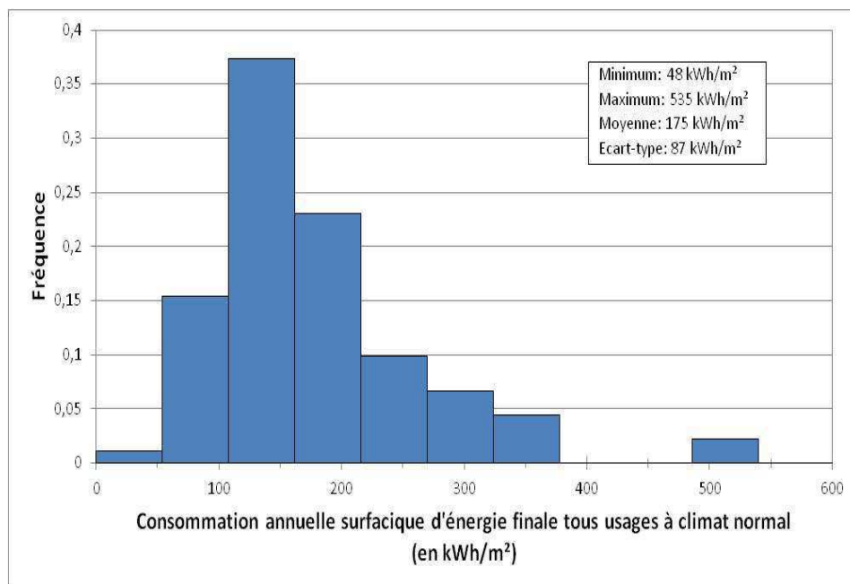
Figure 2.15 Histogramme des consommations annuelles surfaciques d'énergie finale tous usages à climat normal avant travaux de l'échantillon MDE PACA
