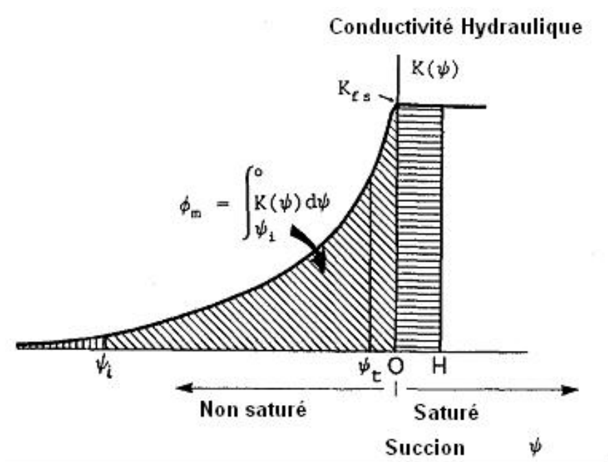
Figure 47. Courbe théorique de la relation entre conductivité hydraulique et succion du sol (Elrick et al. , 1989).
