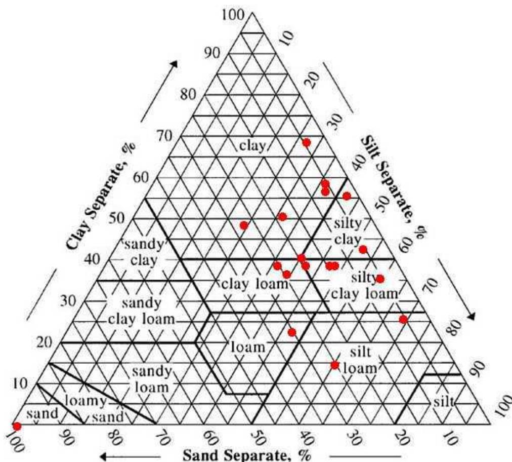
6450 Figure 64. Variations des proportions de l'argile (< 2 µm), du limon (2 à 50 µm), et du sable (> 50 µm) pour les 15 échantillons des sols du territoire d'étude.
