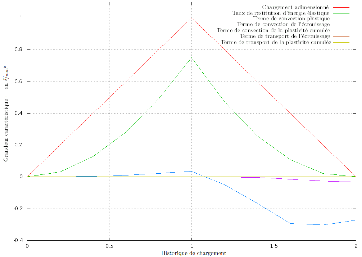
FIGURE 8.2.3: Séparation des différents termes en fonction de l'historique de chargement lors d'un cycle charge-décharge pour une loi isotrope. (En rouge) chargement adimensionné. (En vert) \mathbf{G}_{esh-el} terme d'Eshelby. (En bleu mer) \mathbf{G}_{grad-pl} terme de gradient plastique. (En violet) \mathbf{G}_{grad-ec} terme de gradient d'érouissage. (En bleu clair) \mathbf{G}_{grad-plc} terme indicateur de gradient de plasticité cumulée. (En marron) \mathbf{G}_{tr-ec} terme de transport d'érouissage. (En vert-jaune) \mathbf{G}_{tr-plc} terme indicateur de transport de plasticité cumulée.
