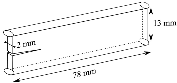
FIGURE 13.2.1: Eprouvette PS (figure tirée de [129]).
