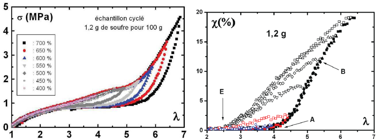
FIGURE 12.1.6: Résultats expérimentaux avec cycles mécaniques à élongations croissantes ( \dot{\lambda} = 2\text{mm}/\text{min} ), allant de 400 à 700% lors d'un test en élongation uniaxiale. (A gauche) Contrainte nominale en fonction de l'élongation. (A droite) Index de cristallinité en fonction de l'élongation (figure tirée de [91]).
