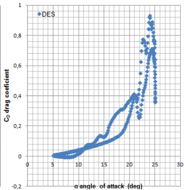
Figure 4.7. Simulations de l'hystérésis de traînée du profil NACA0012
