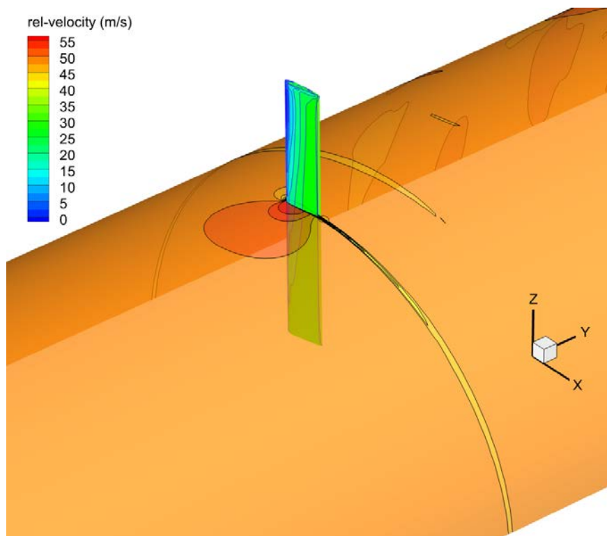
Figure 2.18 Distribution de la vitesse relative et de la pression statique sur la surface de la pale.
