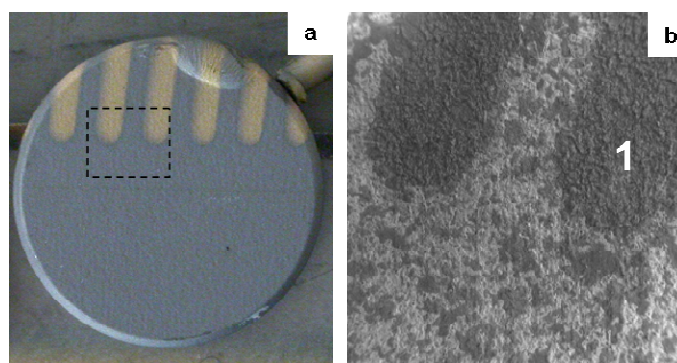
Figure 158 : (a) Photographie de l'échantillon non pré-oxydés après dépôt d'or. (b) Micrographie MEB de surface de l'échantillon non pré-oxydé et vieilli. Le chiffre (1) indique une zone où de l'or a été déposé
