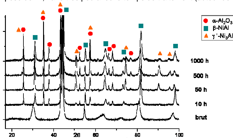
Figure 50 : Diagrammes de diffraction des rayons X des échantillons AM1/NiAlPt. (Pour cause de commodité, l'indexation des raies n'est pas indiquée sur le diagramme.)
