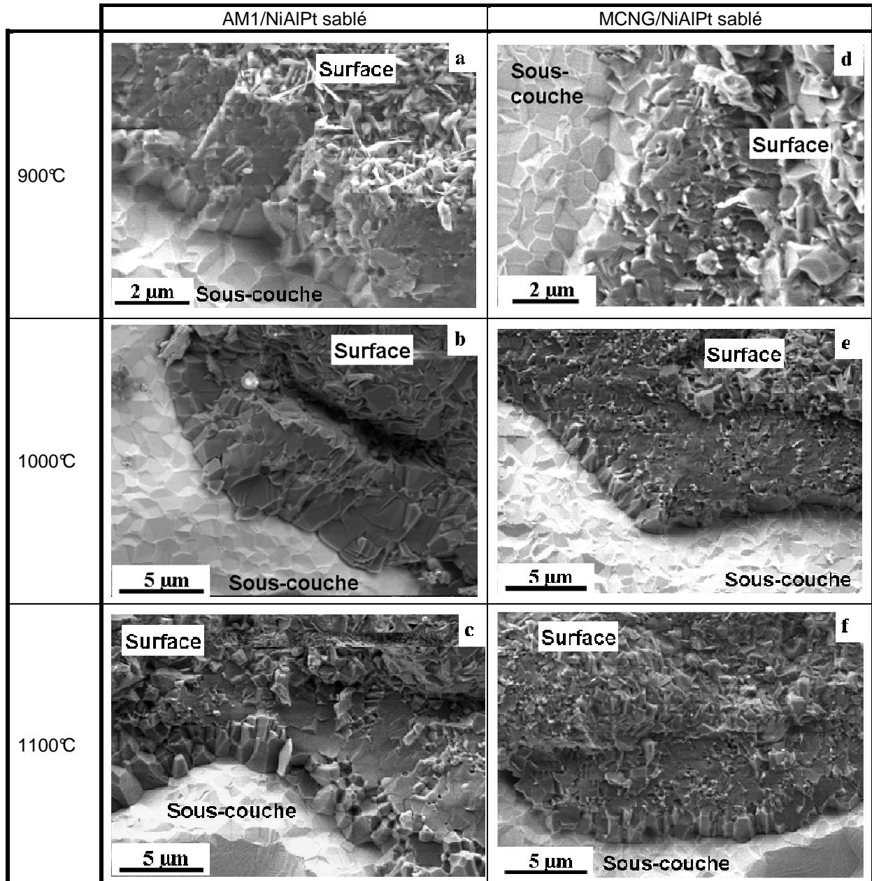
Figure 125 : Micrographies MEB en fractographie de la couche d'oxyde formée sur les systèmes AM1/NiAlPt et MCNG/NiAlPt sablés, pré-oxydés et vieillés.
