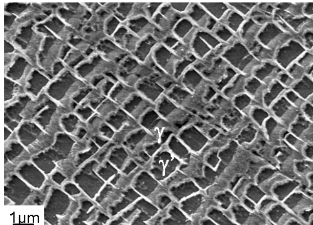
Figure 2 : Micrographie MEB du superalliage MCNG après attaque chimique (Das 2008).
