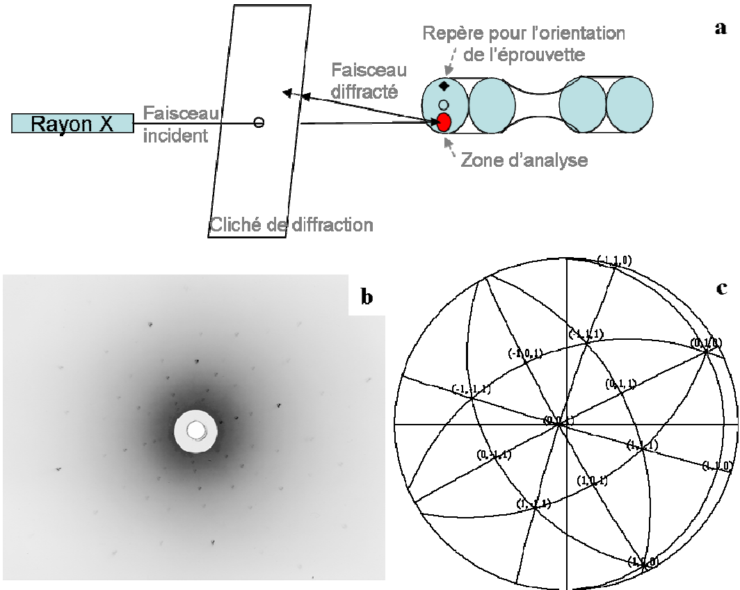
Figure 161 : (a) Principe du LAUE. Un faisceau de rayon X est envoyé sur une face préalablement polie de l'éprouvette. Le faisceau diffracté par le monocristal est renvoyé sur une plaque photosensible. (b) Le cliché ainsi obtenu permet de construire (c) la projection stéréographique du monocristal de superalliage constituant l'éprouvette, et de connaître ainsi son orientation.
