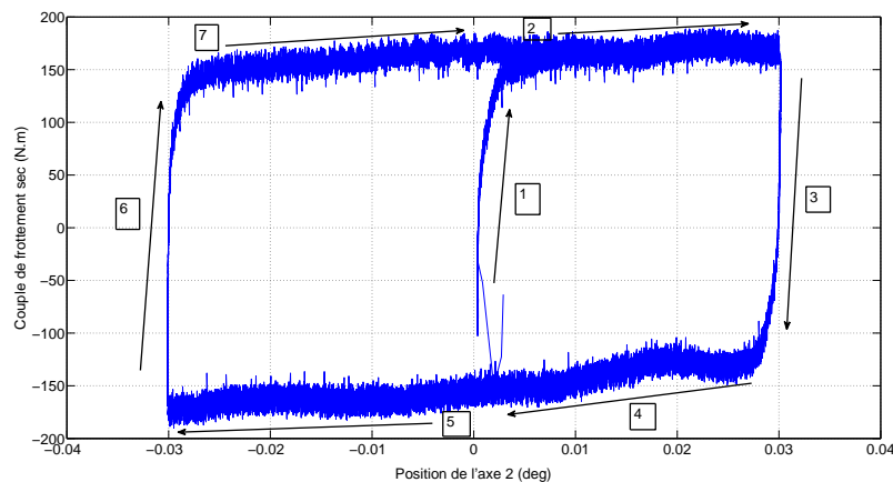
FIGURE 3.20: Couple de frottement en zone de pré-glisement autour de 0 deg
