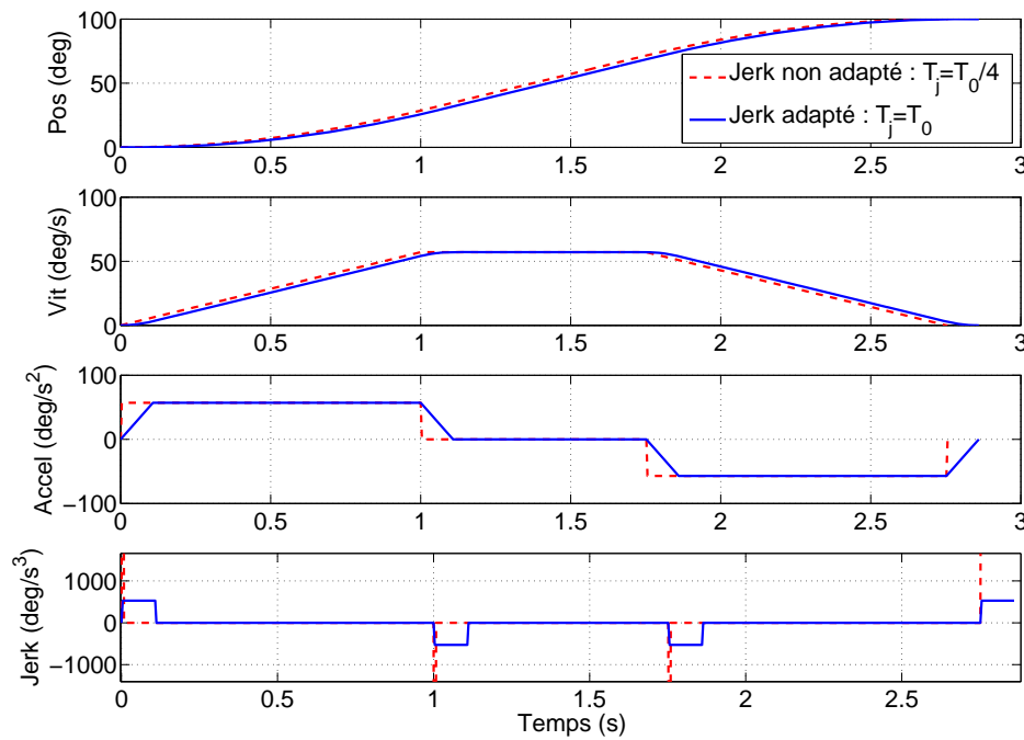
(a) Exemple de profil de référence pour le test avec V_{max} = 57.29 \text{ deg/s} et A_{max} = 57.29 \text{ deg/s}^2
