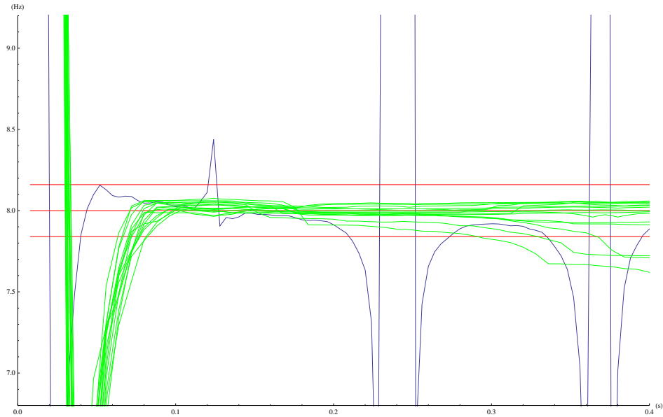
FIGURE 2.14: f_0=8\text{Hz} , \zeta=0 , T_e=4\text{ms} , \text{SNR}=36\text{dB} , A=1 , erreur à 2%
