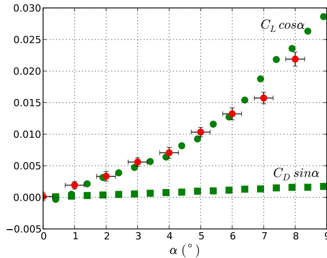
Fig. 2.5 – Composantes de portance C_L \cos \alpha et de traînée C_D \sin \alpha de la force normal F_N tel que C_N = C_L \cos \alpha + C_D \sin \alpha . ( \bullet ) composante de portance mesurée avec la balance bidimensionnelle, ( \bullet ) composante de portance mesurée avec la balance de précision et ( \blacksquare ) composante de traînée mesurée avec la balance bidimensionnelle.
