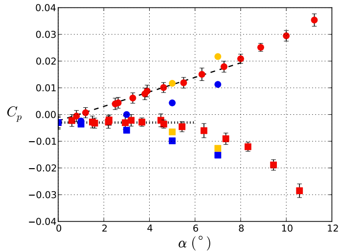
Fig. 4.11 – Coefficients de pression C_p à une distance x = 0.46 m de la pointe amont du cylindre. Pression à l'avant du cylindre ( \theta = 0^\circ ) ( \bullet ) expérimentale, ( \bullet ) numérique sur le cas de référence et ( \bullet ) numérique avec le modèle de turbulence R_{ij} - \epsilon SSG, pression de base ( \theta = 180^\circ ) ( \blacksquare ) expérimentale, ( \blacksquare ) numérique sur le cas de référence et ( \blacksquare ) numérique avec le modèle de turbulence R_{ij} - \epsilon SSG, ( \dots ) valeur de la pression pour le cylindre à l'horizontale C_p = C_p(\alpha = 0^\circ) , ( - - ) régression linéaire C_p = 0.16\alpha(\text{rad}) .
