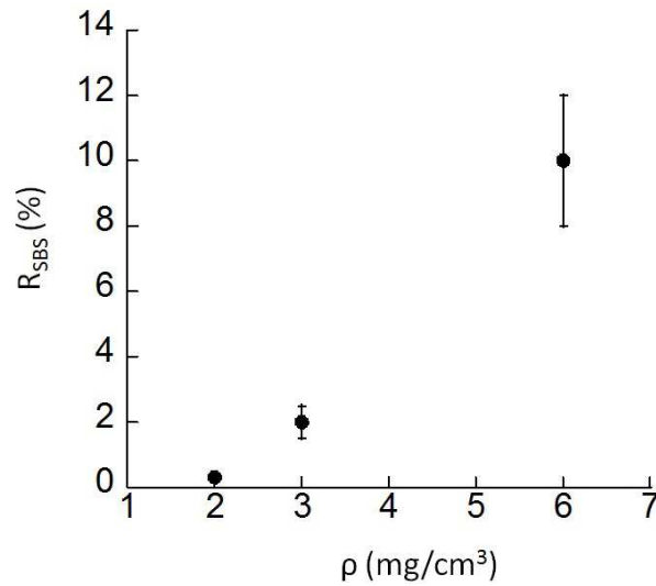
FIGURE 3.27 – Réflectivités instantanées obtenues pour une série de mousses de densité croissante : 2 \text{ mg}/\text{cm}^3 , 3 \text{ mg}/\text{cm}^3 et 6 \text{ mg}/\text{cm}^3 .
