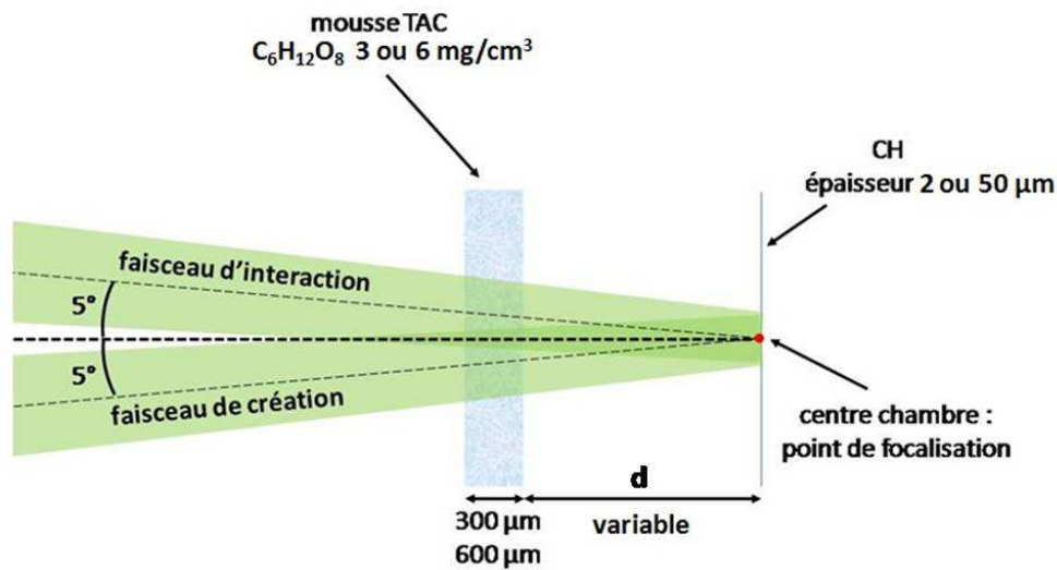
FIGURE 2.10 – Représentation détaillée de la géométrie d'irradiation dans le cas d'une cible composée.
