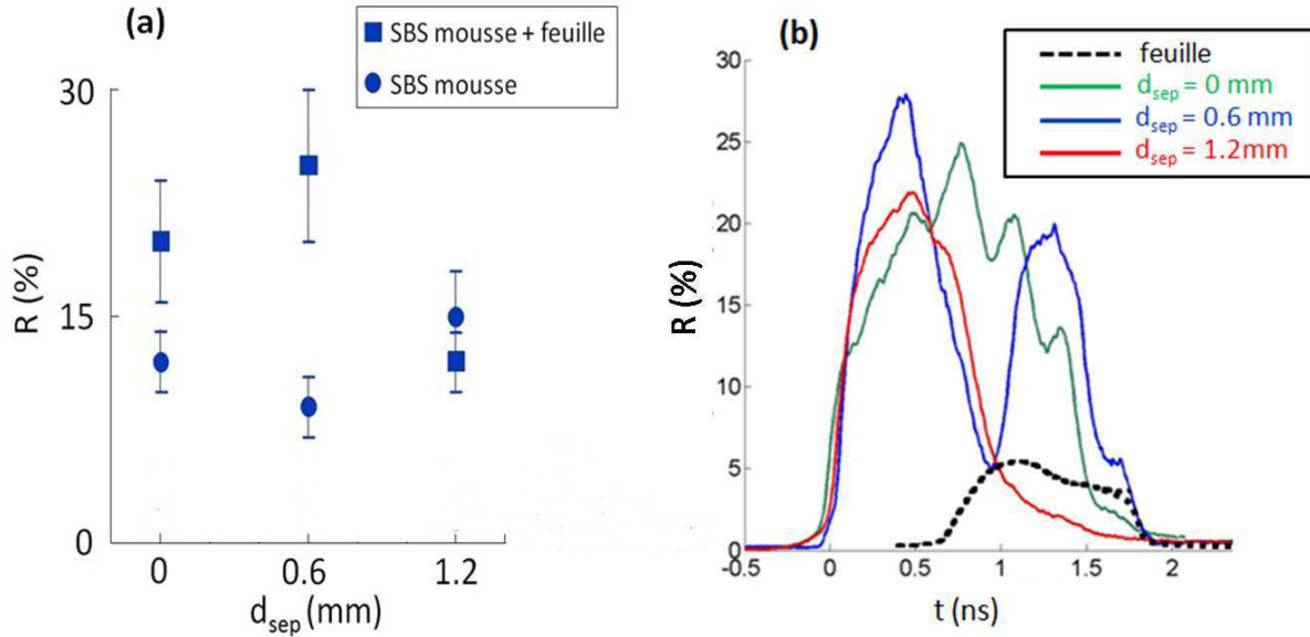
FIGURE 4.5 – (a) Réflectivités Brillouin en fonction de d_{\text{sep}} . Pour les tirs sur cible simple, les trois points correspondent à trois tirs dans les mêmes conditions. (b) Réflectivités Brillouin instantanées pour les trois valeurs de d_{\text{sep}} .
