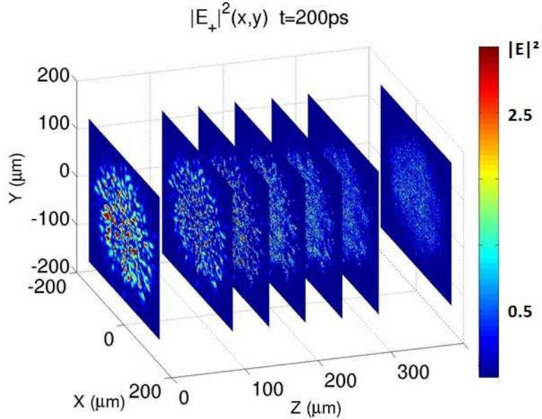
FIGURE 5.15 – Distribution d'intensité laser en fin d'impulsion ( t = 200 ps) dans différents plans transverses le long de l'axe de propagation du laser.
