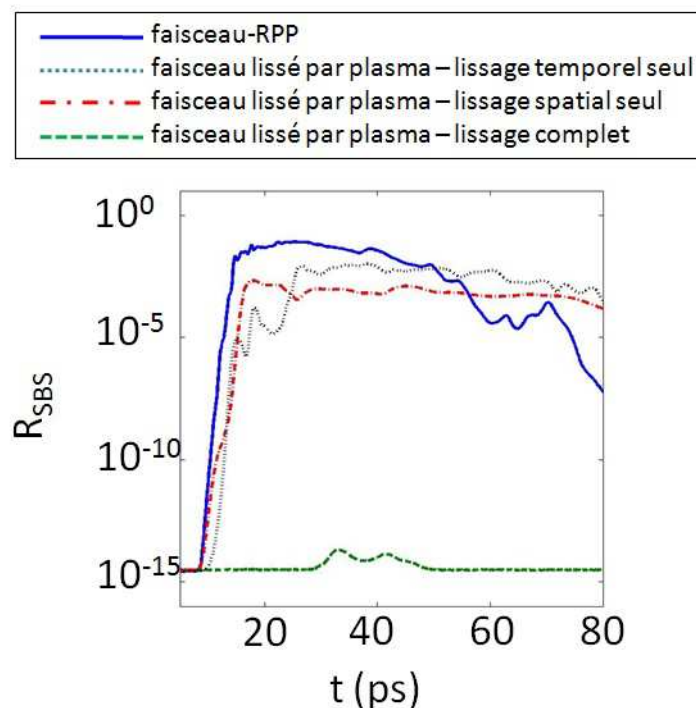
FIGURE 5.19 – Simulation de la réflectivité Brillouin d'une cible solide irradiée par un faisceau d'intensité 2.5 \times 10^{14} W/cm 2 pour différentes conditions de lissage de l'impulsion.
