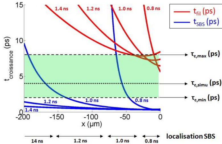
FIGURE 5.21 – Temps caractéristiques de croissance des instabilités de rétrodiffusion Brillouin (bleu) et de filamentation (rouge) comparés au temps de cohérence estimé du faisceau lissé à travers la mousse (zone verte).
