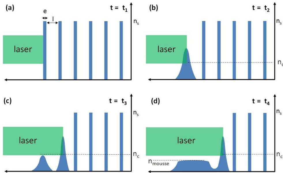
FIGURE 3.7 – Représentation schématique du processus d'ionisation dans les mousses. La progression de l'impulsion laser est présentée à quatre instants t_1 < t_2 < t_3 < t_4 .
