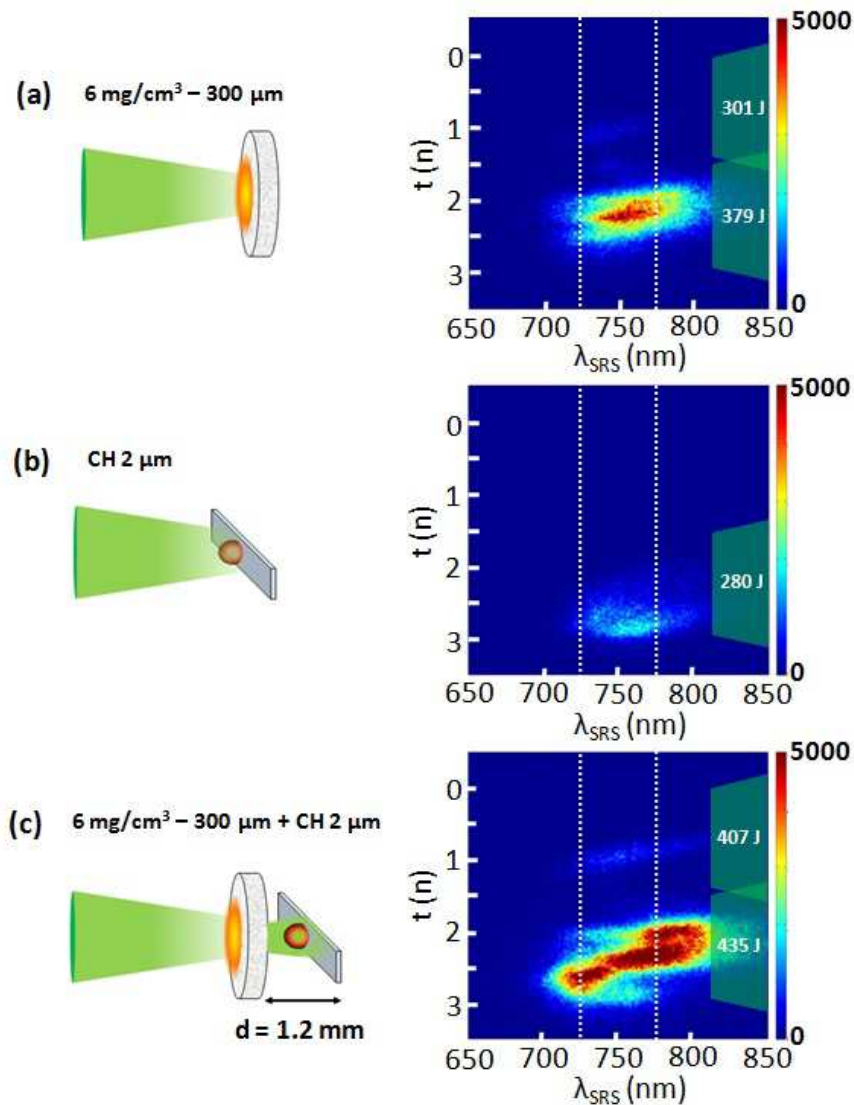
FIGURE 6.8 – Spectres de rétrodiffusion Raman résolus en temps mesurés pour (a) une mousse de 6 \text{ mg/cm}^3 - 300 \mu\text{m} , (b) une cible de CH 2 \mu\text{m} et (c) une cible composée.
