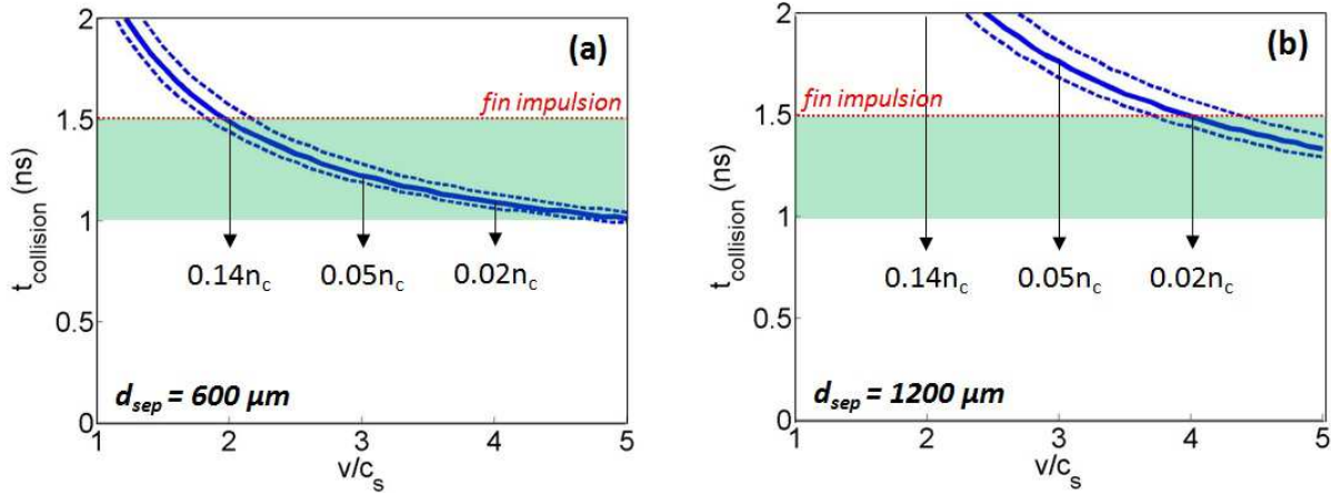
FIGURE 4.7 – Temps de collision des deux plasmas en fonction de la vitesse de détente dans le cadre d’un modèle d’écoulement auto-semblable avec T_e = 1 \text{ keV} pour la mousse et T_e = (0.5 \pm 0.2) \text{ keV} pour la feuille pour (a) une séparation de 0.6 mm et (b) une séparation de 1.2 mm. Les lignes pointillées correspondent aux barres d’erreur sur la température : +0.2 \text{ keV} pour la ligne inférieure et -0.2 \text{ keV} pour la ligne supérieure.
