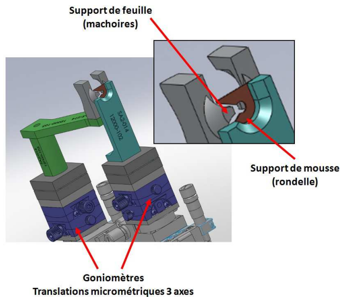
FIGURE 2.6 – Dessin technique de porte-cible pour cible composée avec un support type rondelle pour la mousse et un support type mâchoire pour la feuille.
