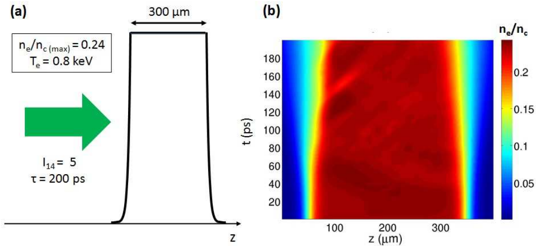
FIGURE 5.14 – (a) Représentation schématique du profil de densité électronique utilisé pour simuler le lissage plasma induit par une mousse de 3 \text{ mg/cm}^3 - 300 \mu\text{m} . (b) Évolution temporelle simulée du profil de densité électronique.
