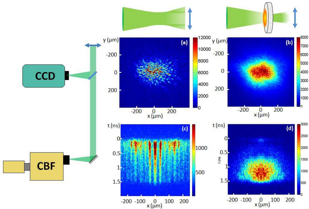
FIGURE 5.3 – Images en transmission obtenues dans le cas d'un tir à vide (images (a) et (c)) et après propagation à travers une mousse de 3 \text{ mg/cm}^3 - 300 \mu\text{m} (images (b) et (d)). La ligne supérieure correspond aux images 2D intégrées temporellement et la ligne du bas aux images 1D résolues en temps.
