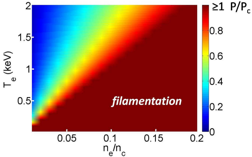
FIGURE 3.3 – Paramètre P/P_c évalué en fonction de la température électronique et de la densité électronique pour un speckle typique de nos conditions laser expérimentales ( P = 329 \text{ MW} ).
