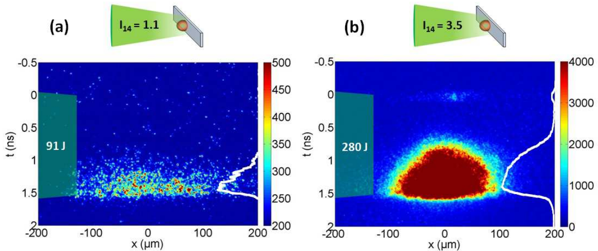
FIGURE 6.5 – Transmission résolue en temps pour une feuille de CH 2 \mu\text{m} en plasma non préformé pour une énergie laser de 91 J (a) et 280 J (b). A droite en blanc sur chaque image, la puissance transmise intégrée spatialement, en unités arbitraires.
