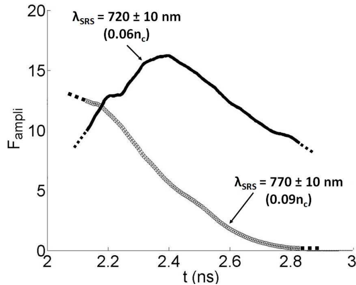
FIGURE 6.14 – Facteur d'amplification tel que défini par la relation 6.17 en fonction du temps pour \lambda_{\text{SRS}} = (720 \pm 10) nm et \lambda_{\text{SRS}} = (770 \pm 10) nm.
