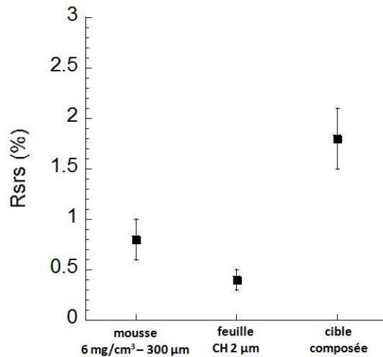
FIGURE 6.9 – Réflectivités Raman intégrées en temps mesurées en fonction de la cible : mousse de 6 mg/cm 3 - 300 μm, feuille de CH 2 μm ou cible composée mousse 6 mg/cm 3 - 300 μm + feuille de CH 2 μm.
