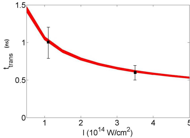
FIGURE 6.6 – Temps à partir duquel une cible de CH 2 \mu\text{m} transmet la lumière en fonction de l'intensité incidente. Les valeurs expérimentales mesurées pour I = 1.1 \times 10^{14} W/cm ^2 et pour I = 3.5 \times 10^{14} W/cm ^2 ont également été reportées.
