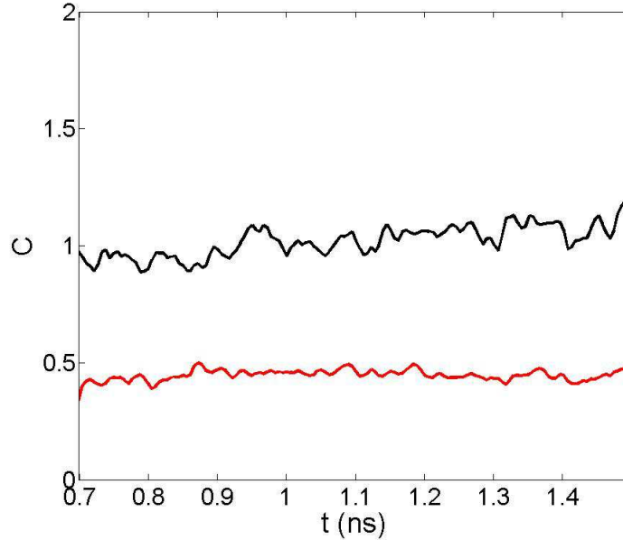
FIGURE 5.5 – Evolution temporelle du contraste spatial dans le cas d'un tir à vide (noir) et après propagation à travers une mousse de 3 \text{ mg/cm}^3 - 300 \mu\text{m} .
