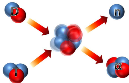
FIGURE 1.1 – Représentation schématique de la réaction de fusion du deutérium et du tritium
