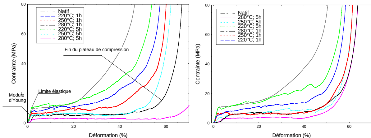
Figure A-6. Compression radiale du bois de pin maritime, traité ou non, soumis à différents taux de déformation: A) 1mm/min; B) 10mm/min.
