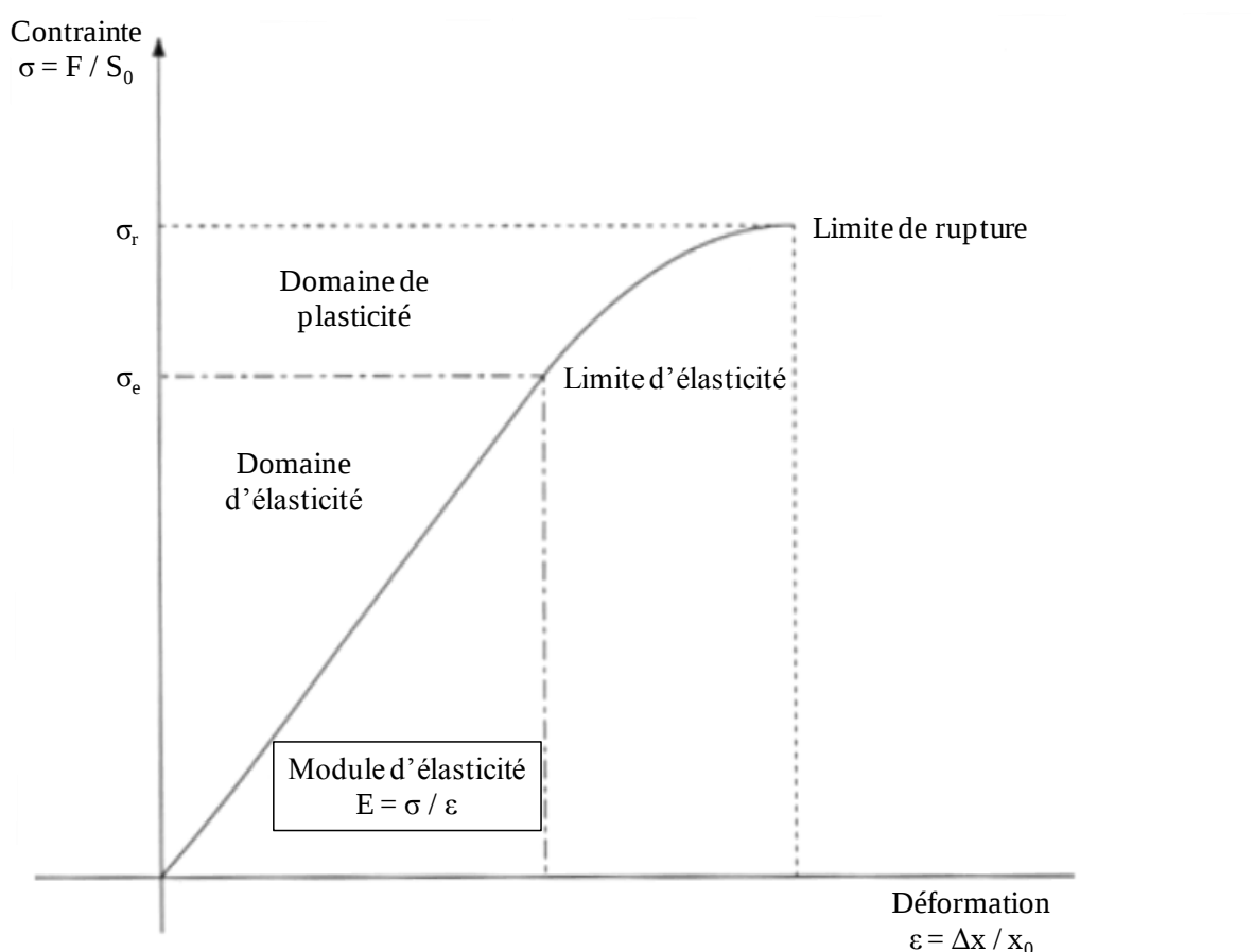
Figure I-14. Comportement des matériaux soumis à des efforts de traction, de compression ou autre : évolution de la contrainte en fonction de la déformation relative.
