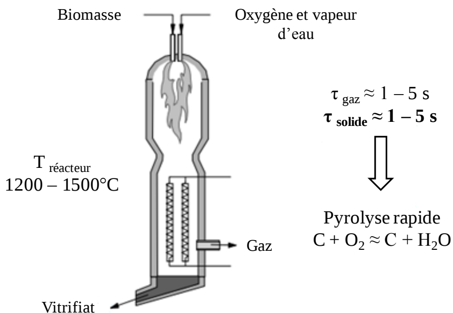
Figure I-2. Schéma de principe d'un gazéifieur à lit entraîné (Mauviel et al., 2009).
