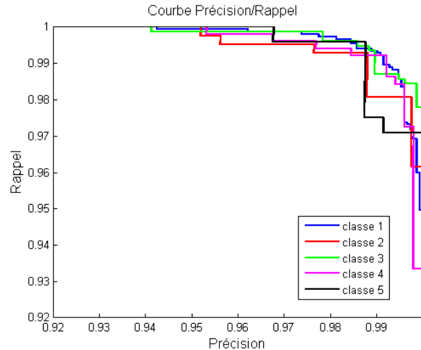
FIGURE 4.26 – Courbe Précision-Rappel obtenue pour SVM 1vs1 avec descripteur HOG 7 \times 3 pour chacune des classes.
