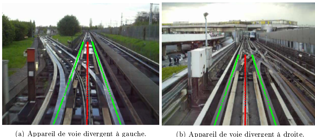
FIGURE 4.1 – Ambigüités de détection des rails à l'approche des appareils de voie divergents.
