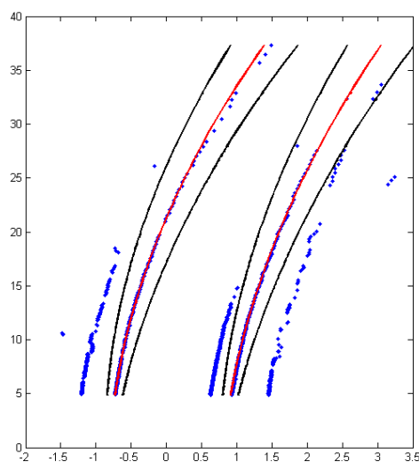
FIGURE 3.28 – Filtrage temporel pour les nuages des points.
