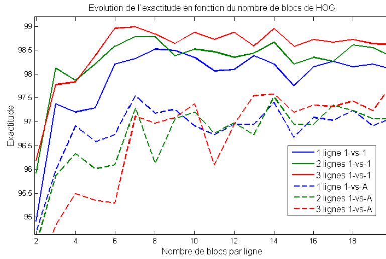
FIGURE 4.25 – Élection du nombre de lignes et de colonnes pour le descripteur de HOG. Nous pouvons voir comment varie l'exactitude pour les deux classifieurs SVS 1vs1 et SVM 1vsA en fonction du nombre de colonnes de lignes du descripteur HOG. SVM 1vs1 se présente plus efficace que 1vsA pour tout les cas. La meilleure exactitude est obtenue pour 7 colonnes et 2 lignes. La taille finale du meilleur descripteur est de 7 \times 3 \times 10 = 210 . L'exactitude est de 98.98%
