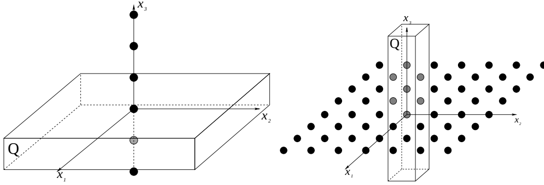
FIG. 2 – L'ensemble \Lambda et la cellule unité Q = Q(\ell) dans le cas des polymères (à gauche) et des films minces (à droite).
