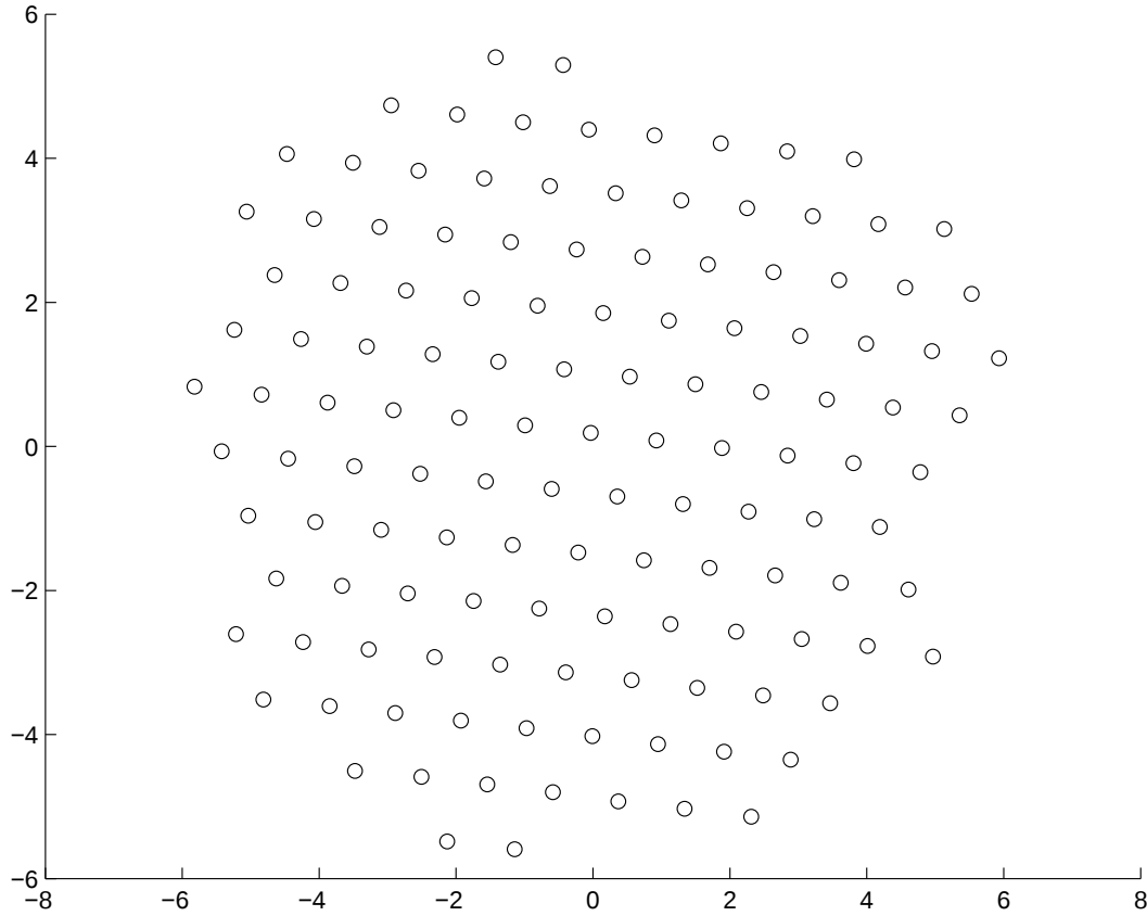
FIG. 4 – Le résultat d'un calcul de gradient conjugué sur le cas du potentiel de Morse (le point de départ est une configuration aléatoire).
