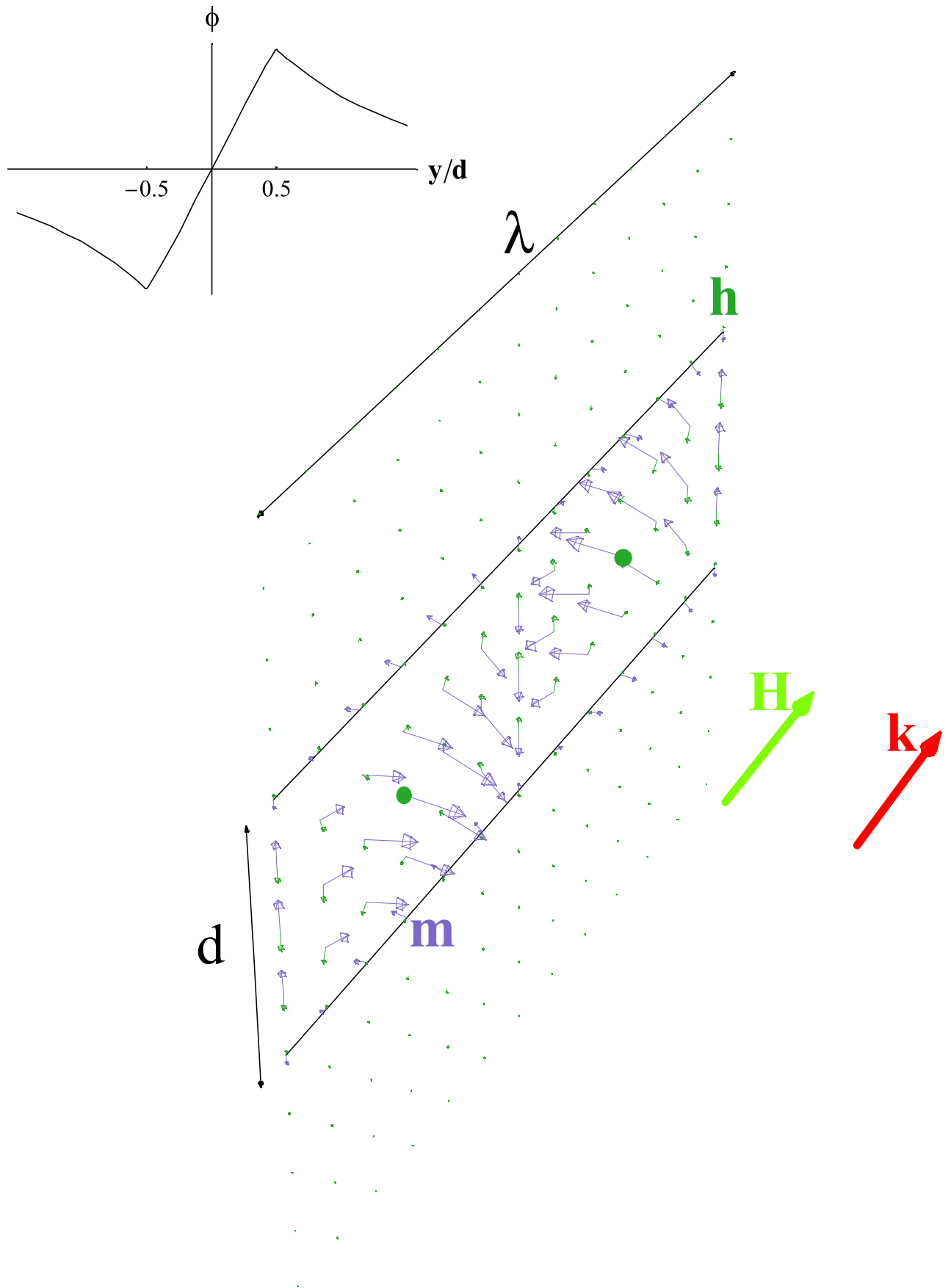
FIG. 2.8 – Structure de l'onde MSBVW. En haut figure le profil du potentiel et en bas une représentation en perspective des vecteurs champ dipolaire dynamique ( h ) et aimantation
