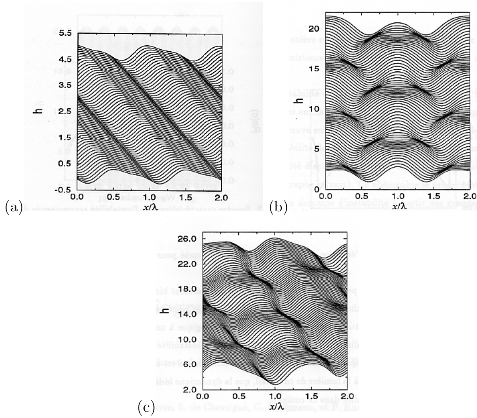
FIG. 5.12 – Quelques états dynamiques obtenus par A.Valance et C. Misbah [24] par simulation de l'équation KSA (a) Mode de parité brisée (PB): état dérivant. (b) Mode de vascillation-respiration (VB): état oscillant. (c) Mode mixte PB+VB: état oscillodérivant.
