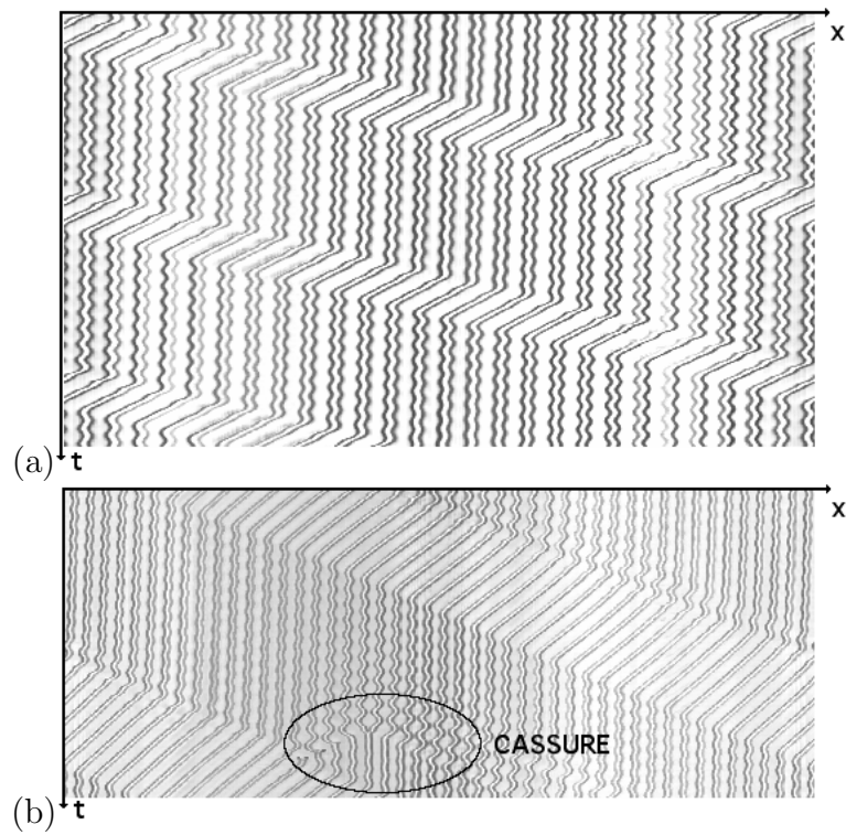
FIG. 5.5 – Sillage oscillant derrière un domaine dérivant. (a) \eta=200 cP, d=10 cm, \Gamma=0.34 cm 2 /s, 25 cols. Durée=17.6 s. (b) \eta=100 cP, d=16.7 cm, \Gamma=0.33 cm 2 /s, 41 cols. Durée= 12.5 s.
