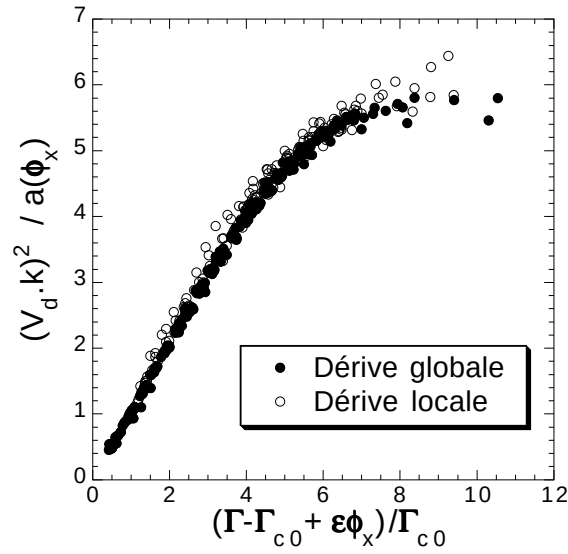
FIG. 3.23 – Rassemblement des mesures de vitesse de dérive sur une seule courbe.
