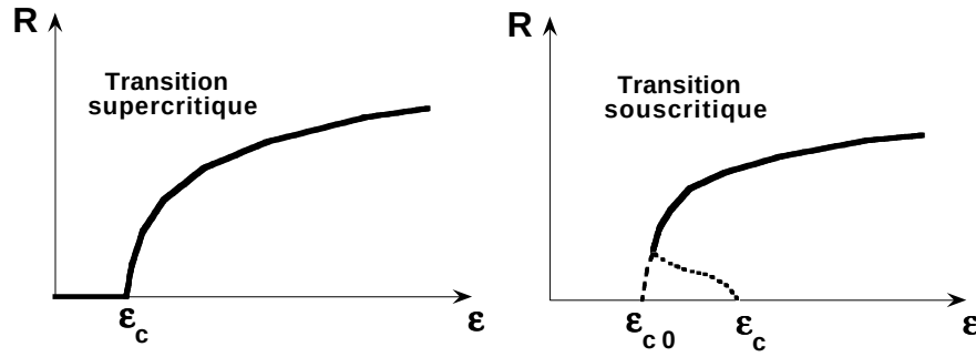
FIG. 1.1 – Représentation schématique des deux types de transition (supercritique et sous critique). R représente la fraction turbulente dans le système, une quantité dont des définitions possibles seront données ultérieurement.
