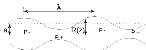
FIG. 2.1 – Instabilité de Rayleigh dans un jet liquide.
