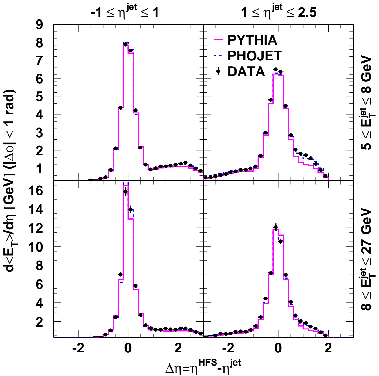
FIG. 5.12 – Flux d'énergie transverse, en fonction de \eta , autour de l'axe des jets dans différents domaines de pseudo-rapidité et d'énergie transverse.
