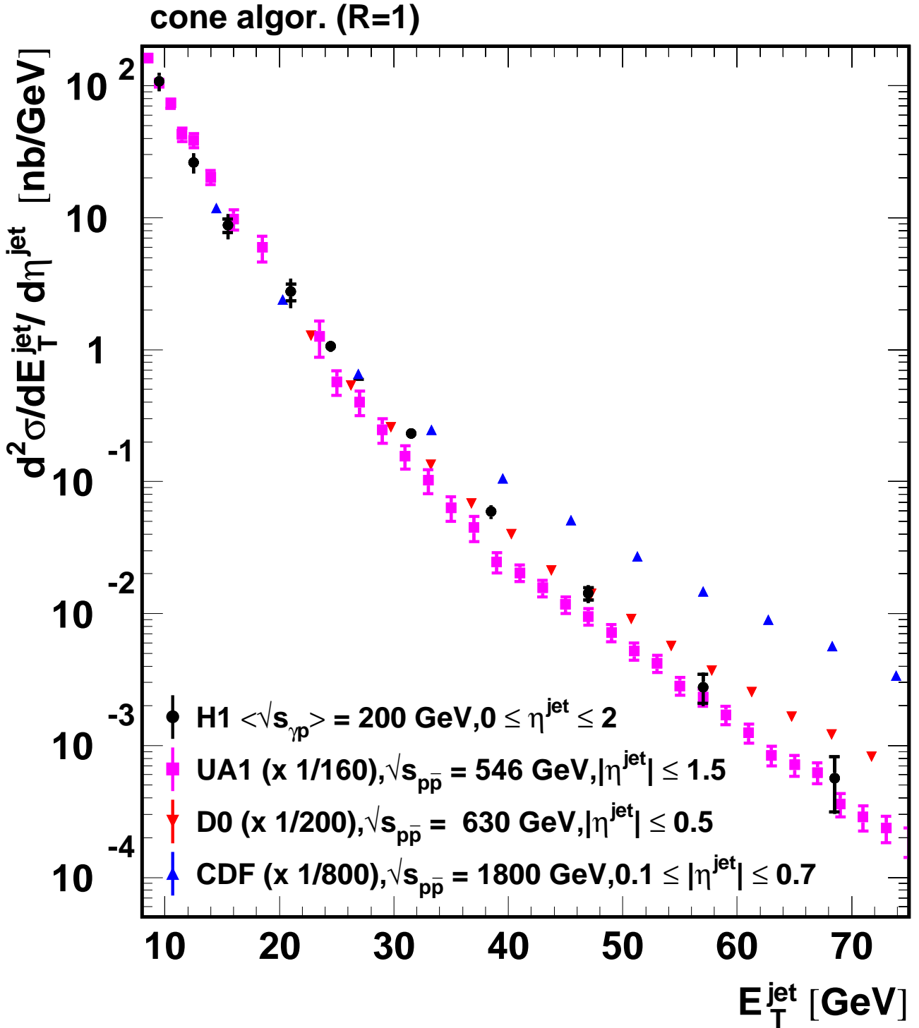
FIG. 7.21 – La section efficace inclusive pour les jet en photoproduction (points noirs) mesurée dans le domaine cinématique 0 \leq \eta^{\text{jet}} \leq 2 , 165 \leq W_{\gamma p} \leq 242 \text{ GeV} . Les barres d'erreurs internes représentent les erreurs statistiques, les barres d'erreurs externe la somme quadratique des erreurs statistique et systématique. Les mesures de CDF [162], D0 [161] et UA1 [160] pour la production inclusive de jets dans les collision p\bar{p} à différente énergie dans le centre de masse sont représentées avec une normalisation ajustée de façon à reproduire celle des données \gamma p .
