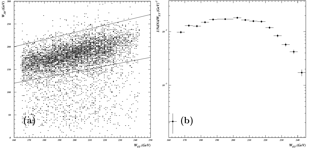
FIG. 5.7 – Corrélation entre W_{JB} et W_{ET} (a), et distribution, normalisée à l'unité, de W_{ET} (b) observées avec le lot Coll.
