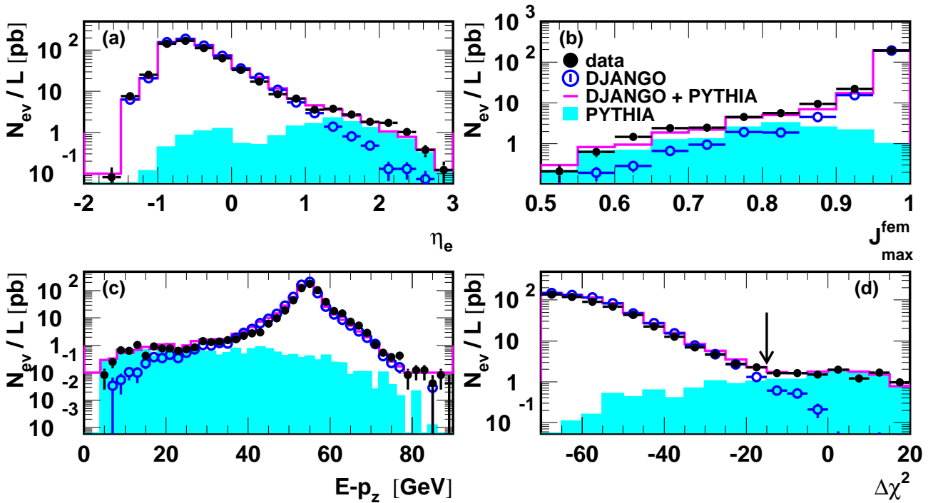
FIG. 6.6 – Distributions, normalisées à la luminosité, de la pseudo-rapidité du candidat positron (a), de J_{max}^{fem} (b), de (E - p_z) (c) et de la « distance » \Delta\chi^2 (d) obtenues avec les événements possédant un candidat positron identifié dans le LAr. Les points noirs représentent la contribution des données, les points blancs celle prédite par DJANGO. L'histogramme grisé représente la contribution des événements de photoproduction donnée par PYTHIA. La somme des distributions obtenues avec PYTHIA et DJANGO est indiquée par l'histogramme en trait plein. Pour obtenir ces distributions la coupure 0.1 \leq y \leq 0.9 a été relâchée.
