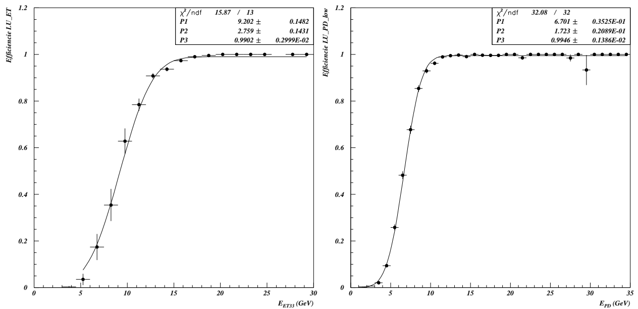
FIG. 5.2 – Efficacité de déclenchement des conditions LU_ET et LU_PD_low en fonction de l'énergie déposée dans les calorimètres ET et PD.
