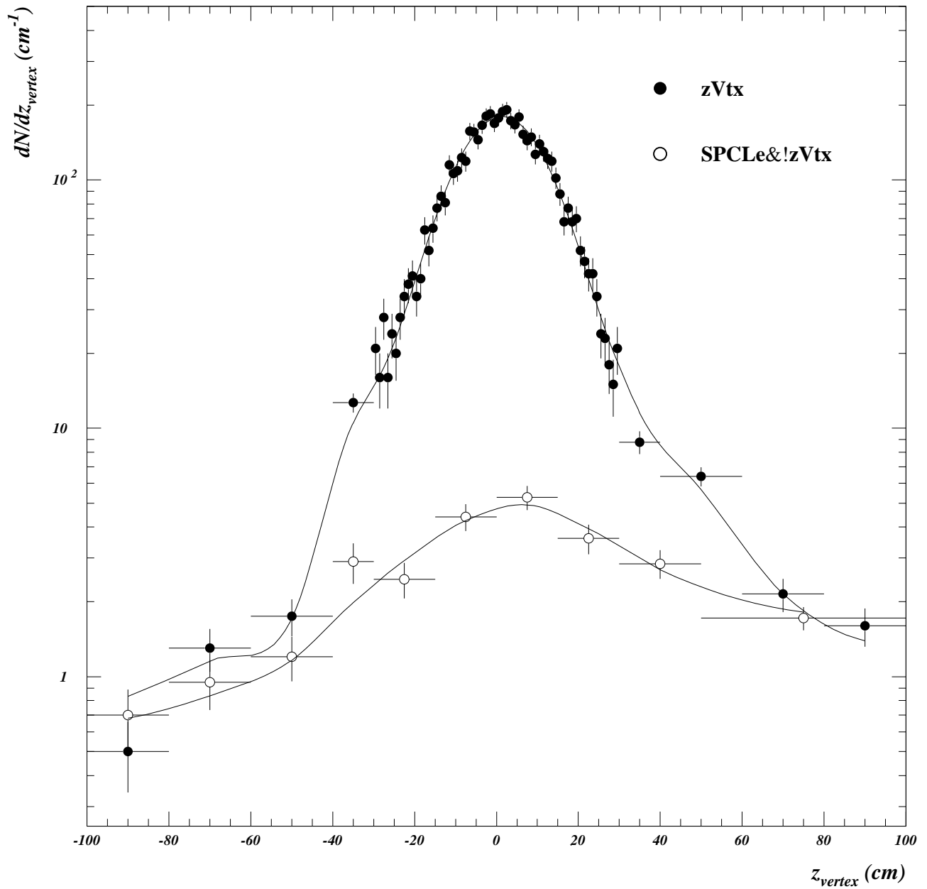
FIG. 5.5 – Ajustements des distributions en z_v pour les deux conditions de déclenchement zVtx (points noirs) et SPCLe\&!zVtx (points blancs).
