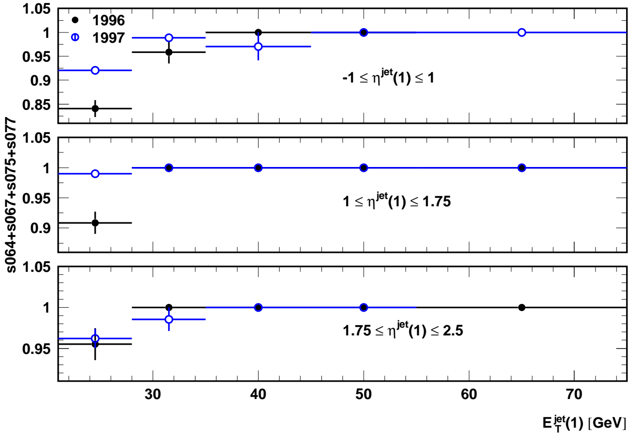
FIG. 6.9 – Efficacité de déclenchement de la condition s064/s067/s075/s077 en fonction de E_T^{jet}(1) dans trois domaines en \eta^{jet}(1) pour les deux années 1996 et 1997. Les jets sont définis avec l'algorithme k_T .
