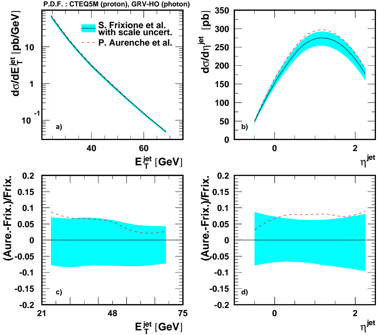
FIG. 2.12 – Sections efficaces différentielles de production inclusive de jets 21 \leq E_T^{\text{jet}} \leq 75 GeV, -1 \leq \eta^{\text{jet}} \leq 2.5 dans les collision ep à Q^2 \leq 1 GeV 2 et 0.1 \leq y \leq 0.9 calculées avec l'algorithme k_T en fonction de E_T^{\text{jet}} (a) et \eta^{\text{jet}} (b) avec la méthode de soustraction [116] et la méthode du découpage de l'espace de phase [124].
