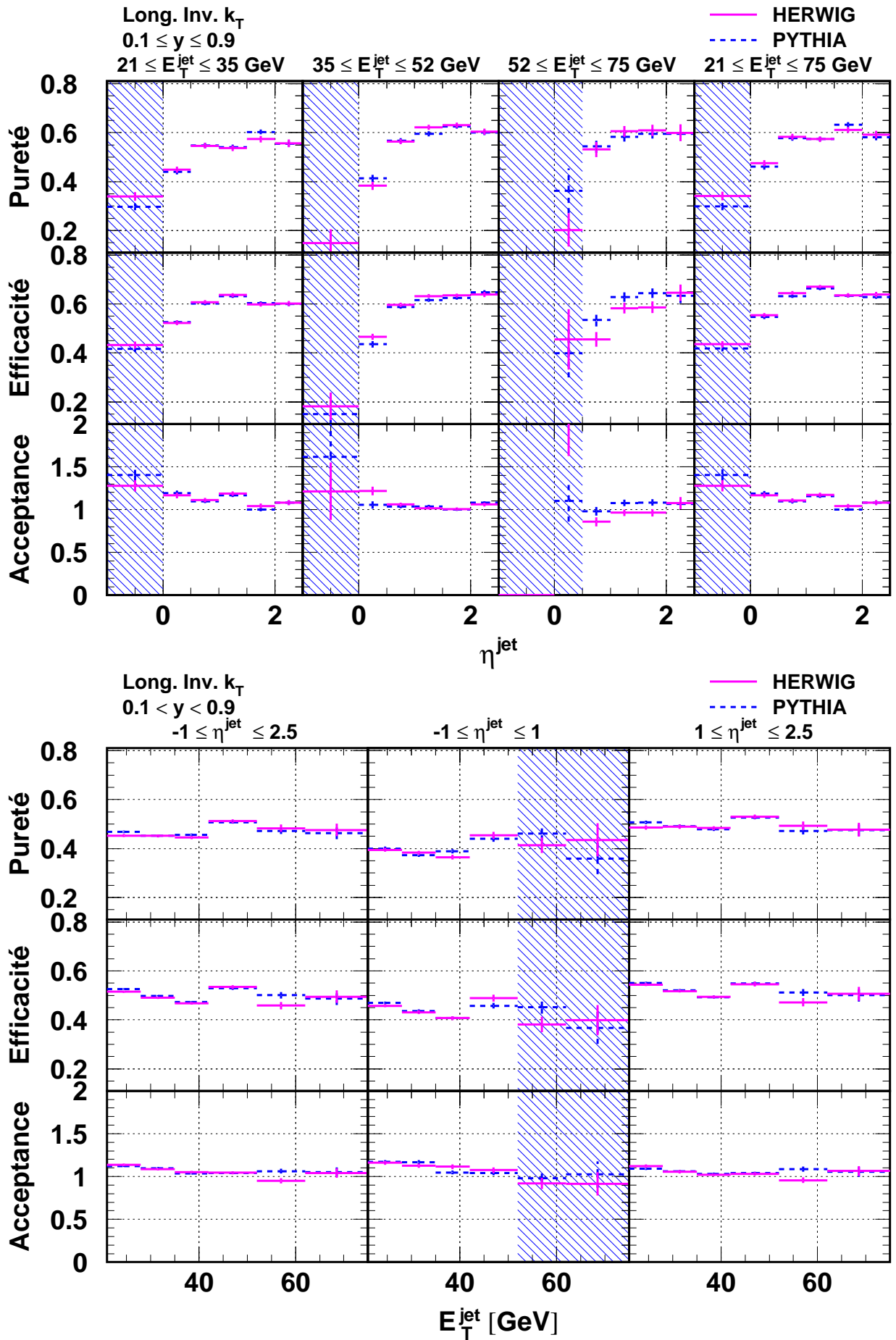
FIG. 6.22 – Pureté, efficacité et acceptance des intervalles en \eta^{jet} et E_T^{jet} pour 0.1 \leq y \leq 0.9 . Les zones hachurées ne sont pas retenues pour la mesure finale.
