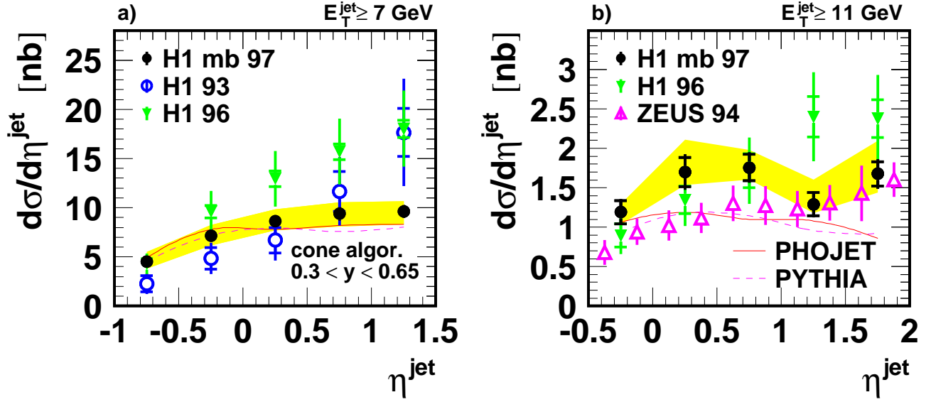
FIG. 7.17 – Sections efficaces différentielles pour la production inclusive de jets en photoproduction ( Q^2 \leq 0.01 \text{ GeV}^2 , 0.3 \leq y \leq 0.65 ) mesurées avec l’algorithme de cône en fonction de la pseudo-rapidité des jets d’énergie transverse supérieures à 7 GeV (a) et 11 GeV (b). L’erreur systématique due à l’échelle d’énergie hadronique des jets est représentée par la bande grisée. Les données (« H1 97 mb ») sont comparées aux mesures précédentes. La normalisation des Monte-Carlos est ajustée aux données.
