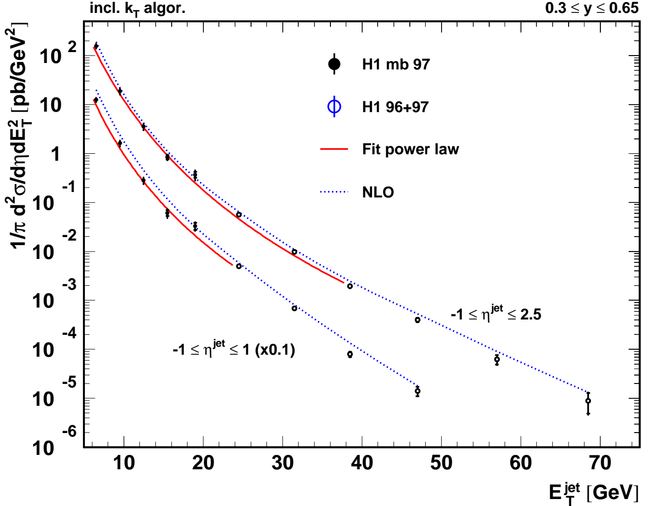
FIG. 7.14 – Sections efficaces pour la production inclusive de jets en photoproduction mesurées pour 164 \leq W_{\gamma p} \leq 242\ GeV . Les jets sont reconstruits avec l’algorithme k_T dans les intervalles -1 \leq \eta^{jet} \leq 2.5 et -1 \leq \eta^{jet} \leq 1 . Les barres d’erreur internes représentent l’erreur statistique des données, les barres d’erreur externes, la somme quadratique des erreurs statistique et systématique. Les données issues des analyses à petit et grand E_T^{jet} sont indiquées par des points noirs et blancs respectivement. Les courbes en traits pleins représentent les résultats d’ajustement par une loi de puissance (équation 7.3). Les données sont comparées aux prédictions au NLO de QCD utilisant les paramétrisations CTEQ5M et GRV des densités de partons dans le proton et les photon.
