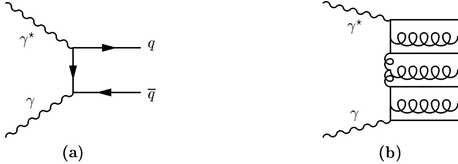
FIG. 1.12 – Exemples de diagrammes contribuant aux fonctions de structures du photon, en QED (a) et en QCD (b).
