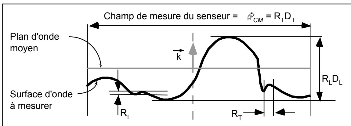
Figure II32a : Dynamiques et résolutions transverses et longitudinales requises pour caractériser une surface d'onde (courbe en gras ). Le vecteur d'onde moyen \vec{k} qui lui est associé est parallèle à l'axe optique du senseur (en pointillés).
