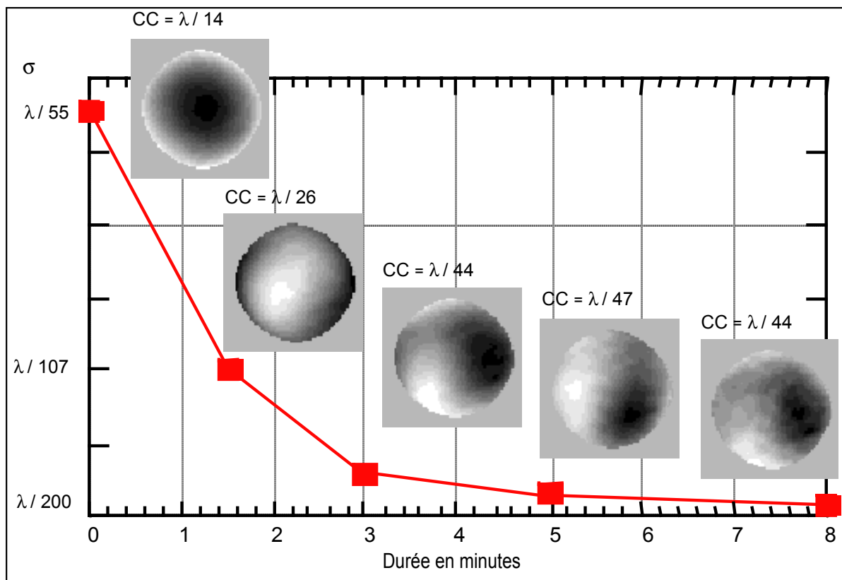
Figure II35g : Evolution des distorsions de phase générées par un barreau de verre phosphate dopé au néodyme de 45 mm de diamètre pompé par lampes flashes à t=0 . La courbe représente la décroissance de l'écart type (avec \lambda = 1 micron). Pour chaque point de mesure sont représentées une carte de \Delta OPD ainsi que la valeur crête à crête associée.
