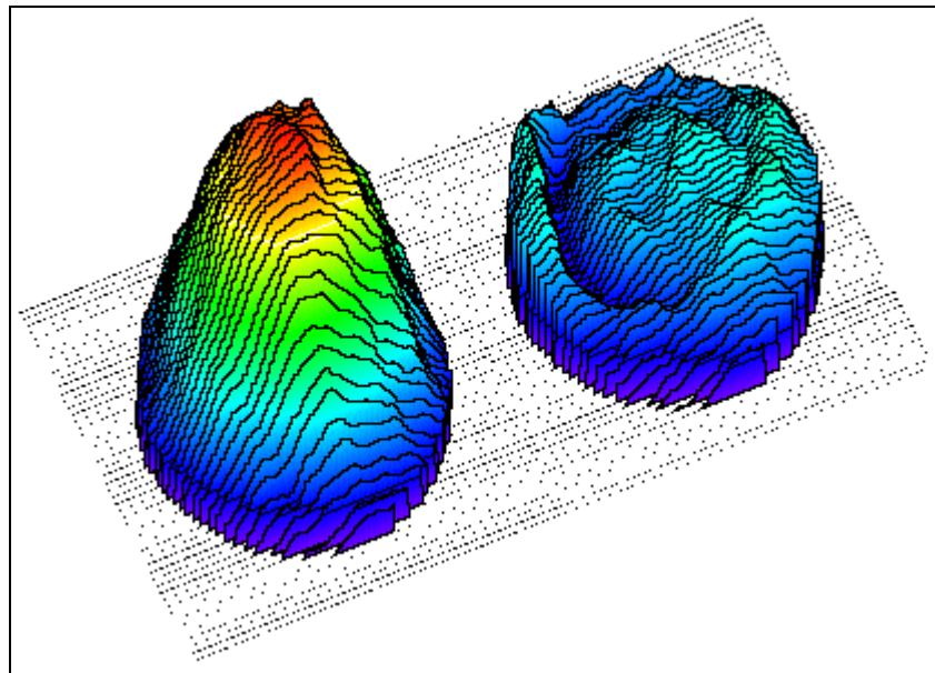
Figure II5p : Vues en trois dimensions des surfaces d'onde obtenues avant correction (à gauche) et après correction (à droite). La valeur de CC passe de 0,48\lambda à 0,20\lambda tandis que celle de \sigma passe de 0,13\lambda à 0,04\lambda .
