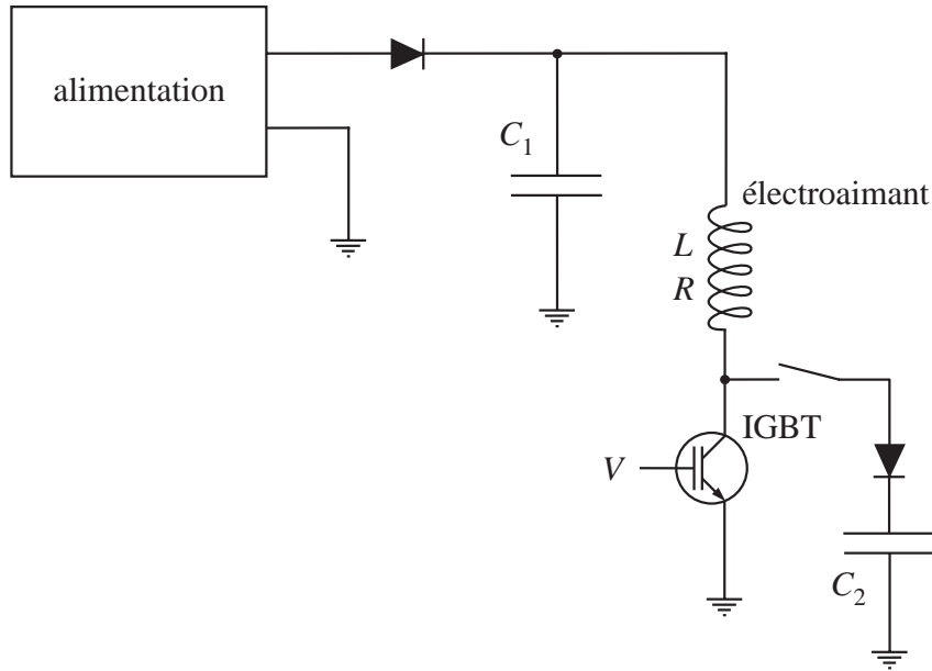
FIG. III.12 – Circuit d'alimentation de l'électroaimant. Il existe en deux exemplaires, un pour les bobines du dipôle, et un pour celles du quadropôle. Les capacités C_1 et C_2 servent respectivement à la montée et à la coupure du courant. L'ouverture et la fermeture du circuit se fait grâce au transistor IGBT, piloté par la tension de commande V . La séquence expérimentale est la suivante. On charge la capacité C_1 (avec un dispositif non représenté) jusqu'à ce qu'elle contienne l'énergie \frac{1}{2}LI^2 , I étant le courant d'alimentation réalisant l'adaptation durant le transfert (§ III.3.2). Puis on ferme l'IGBT au moment du transfert. En 1/4 d'oscillation LC_1 , la capacité se décharge dans la bobine L jusqu'à ce que le courant atteigne la valeur I . L'alimentation prend alors le relais. Pour couper le courant, on commute la capacité C_2 sur le circuit, puis on ouvre l'IGBT. Le courant chute en 1/4 d'oscillation LC_2 , et la diode l'empêche de s'inverser. Puis la capacité est déchargée dans un circuit annexe non représenté.
