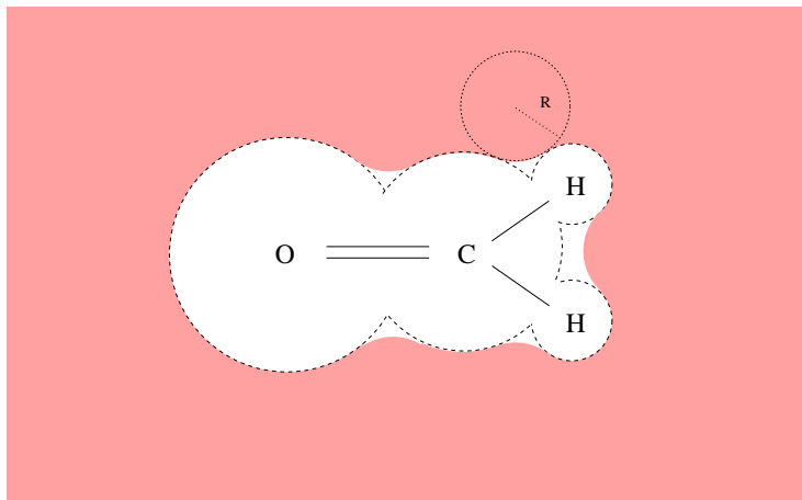
FIG. 3: Cavité \Omega^{sc} pour une molécule de formaldéhyde.
