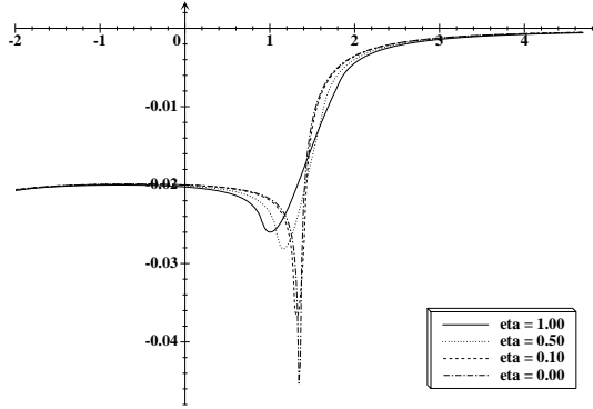
FIG. 8: Profil de la densité de charge \sigma_1 pour \eta = 1.00 , \eta = 0.50 , \eta = 0.10 et \eta = 0.00
