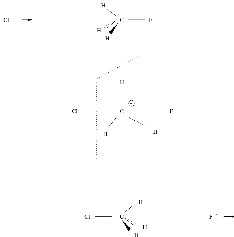
FIG. 6: Réaction de substitution \text{Cl}^- + \text{CH}_3\text{F} \rightarrow \text{ClCH}_3 + \text{F}^- .
