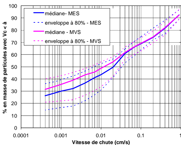
Figure 40: comparaison des vitesses de chute des MES et des MVS dans les eaux de nettoyage de voirie
