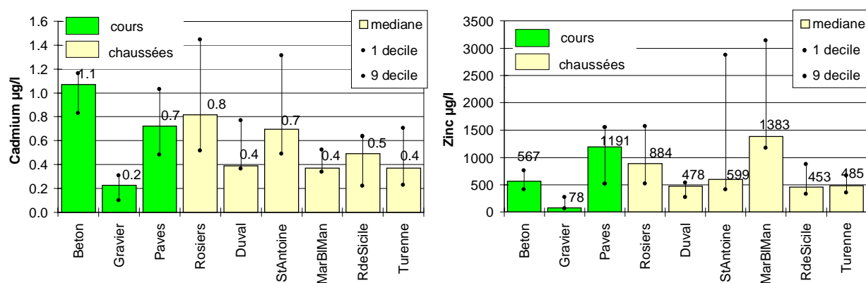
Figure 79: ordre de grandeur des concentrations en cadmium et en zinc des eaux de ruissellement pour les différents sites de cours et de chaussées
