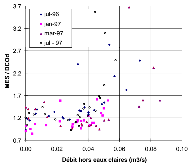
Figure 64: relation entre le rapport MES/DCOd et le débit moyen horaires (moyenne sur chaque campagne)
