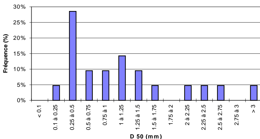
Figure 9 : granulométrie des dépôts dans le collecteur Vieille du Temple
