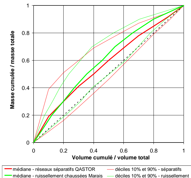
Figure 106 : comparaison du fuseau de courbes M(V) obtenu pour les eaux de ruissellement du Marais, avec le fuseau de courbe M(V) établi par [Saget; 94] pour les eaux pluviales à l'exutoire de réseaux séparatifs
