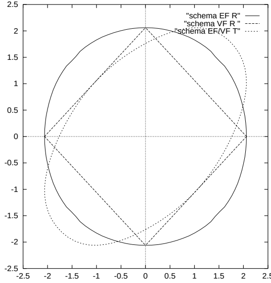
FIG. II.8 – Domaines de stabilité des trois schémas “sans diffusion numérique” avec \beta = \frac{1}{3} en RK4.
