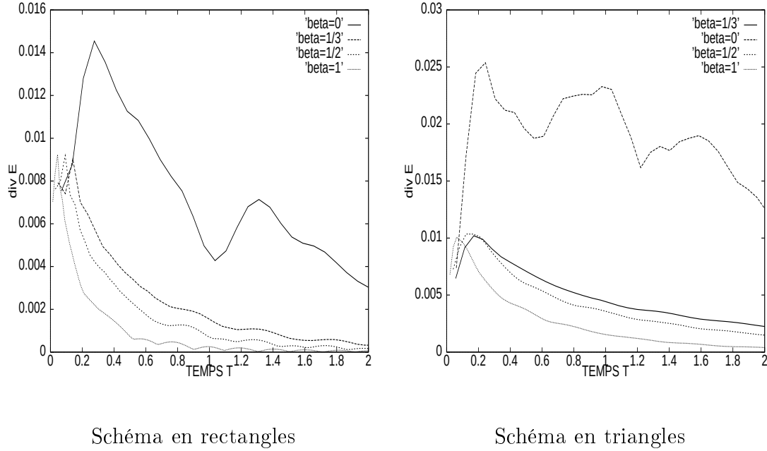
FIG. IV.11 – Influence du paramètre de décentrage \beta .
