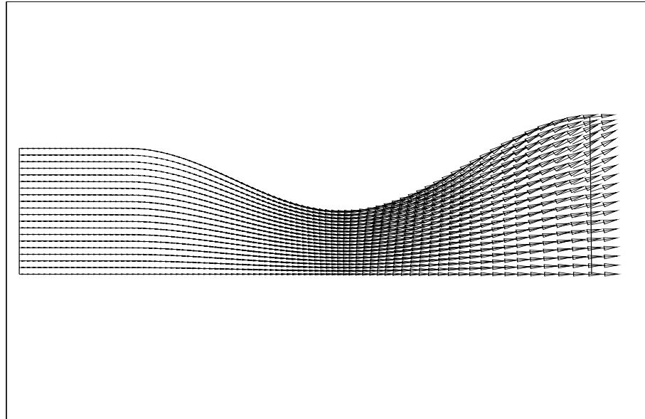
FIG. VIII.43 – Champ de vitesse du gaz pour r = 50.10^{-6} m avec la “méthode de splitting”.
