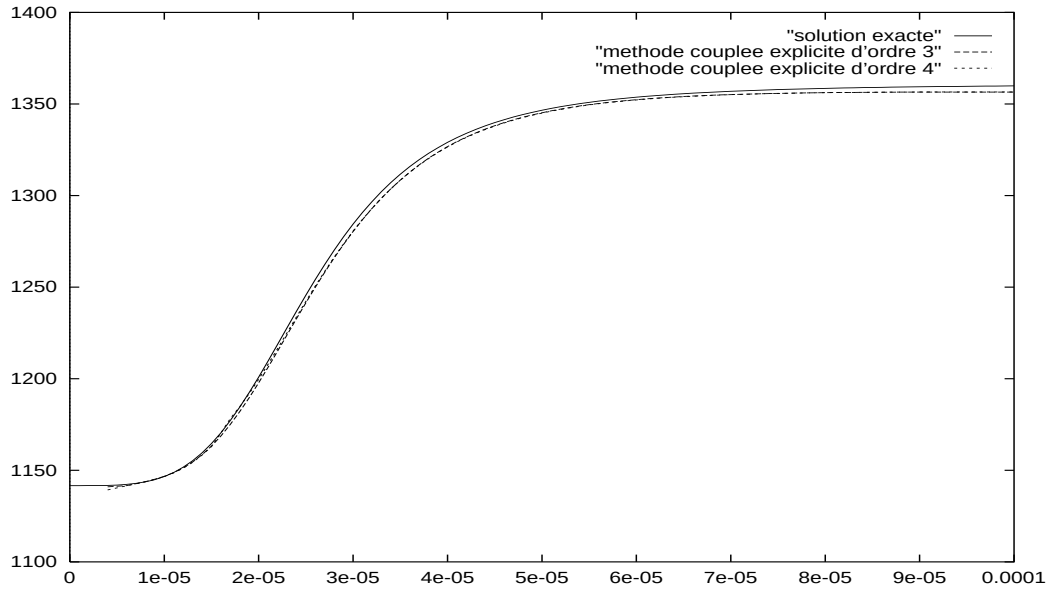
FIG. VIII.6 – Vitesse du son pour les “méthodes couplées” d’ordre trois et quatre.
