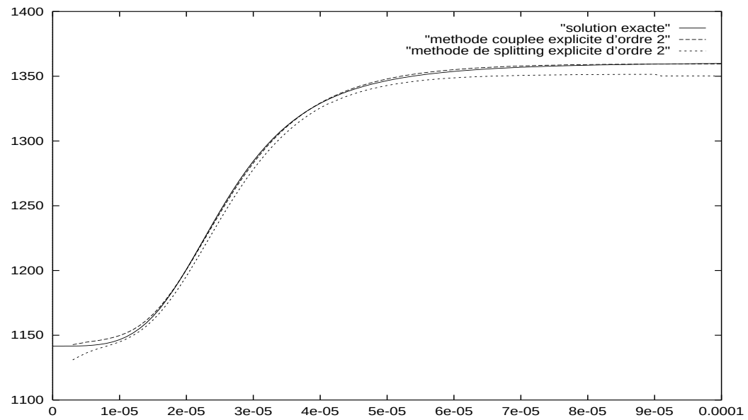
FIG. VIII.4 – Vitesse du son pour les méthodes d'ordre deux.
