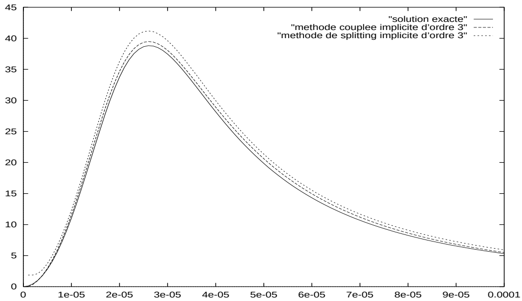
FIG. VIII.8 – Amortissement pour les schémas de Crank-Nicolson appliqués aux deux méthodes.
