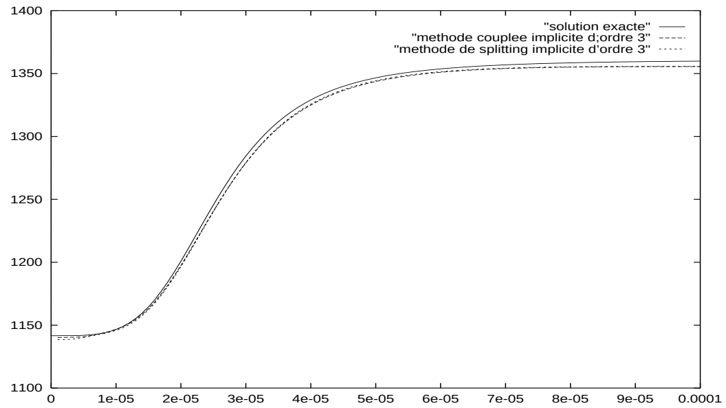
FIG. VIII.9 – Vitesse du son pour les schémas de Cranck-Nicolson appliqués aux deux méthodes.
