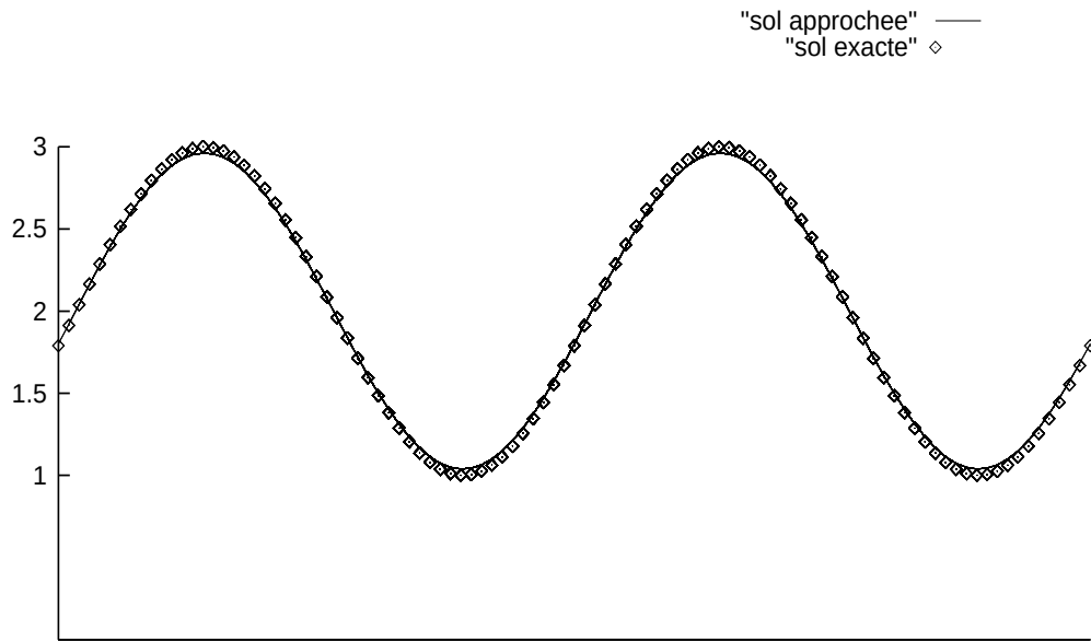
FIG. II.10 – Solution obtenue avec le schéma VF R, sans masse, \beta = \frac{1}{3} .
