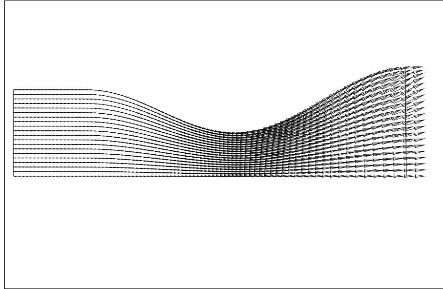
FIG. VIII.42 – Champ de vitesse du gaz pour r = 50.10^{-6} m avec la “méthode couplée”.
