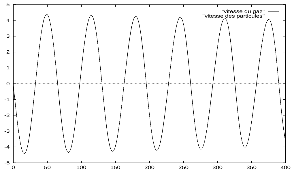
FIG. VIII.11 – Vitesse du gaz et des particules pour r = 3 \cdot 10^{-6} \text{ m} avec la “méthode couplée”.
