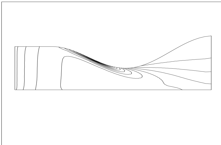
FIG. VIII.41 – Densité des gouttes pour r = 50.10^{-6} m avec la “méthode de splitting”.
