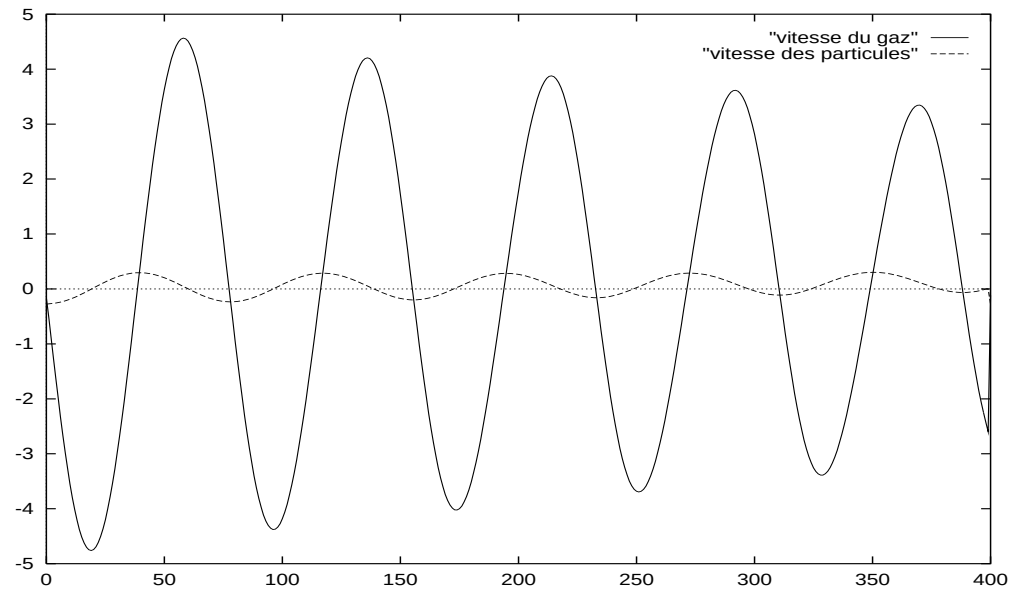
FIG. VIII.12 – Vitesse du gaz et des particules pour r = 1 \cdot 10^{-4} \text{ m} avec la “méthode couplée”.
