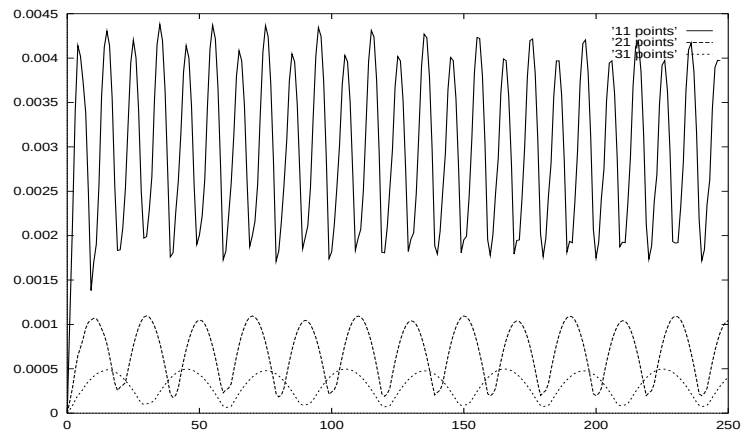
FIG. III.17 – Influence du pas de maillage sur la divergence pour les schémas modifiés d'ordre quatre.
