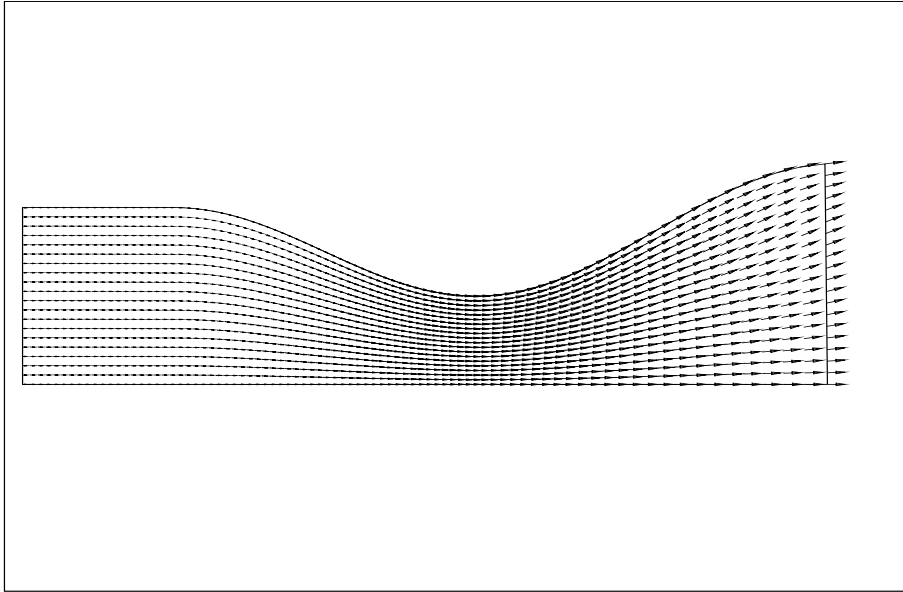
FIG. VIII.36 – Champ de vitesse des gouttes pour r = 1.10^{-6} m avec la “méthode couplée”.
