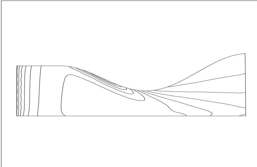
FIG. VIII.33 – Densité des gouttes pour r = 1.10^{-6} m avec la “méthode de splitting”.
