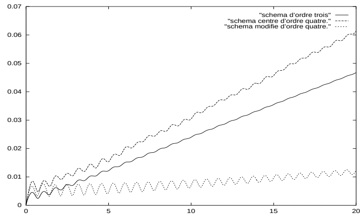
FIG. III.12 – Comparaison des schémas pour un maillage en triangles.
