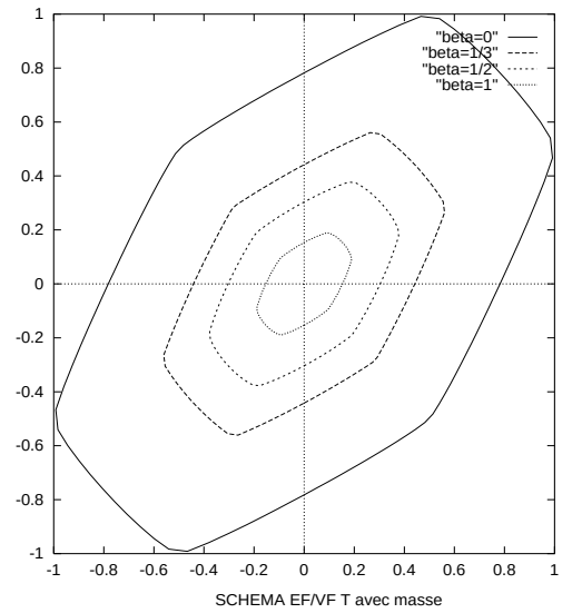
FIG. II.5 – Domaines de stabilité des schémas précis à l'ordre trois en temps
