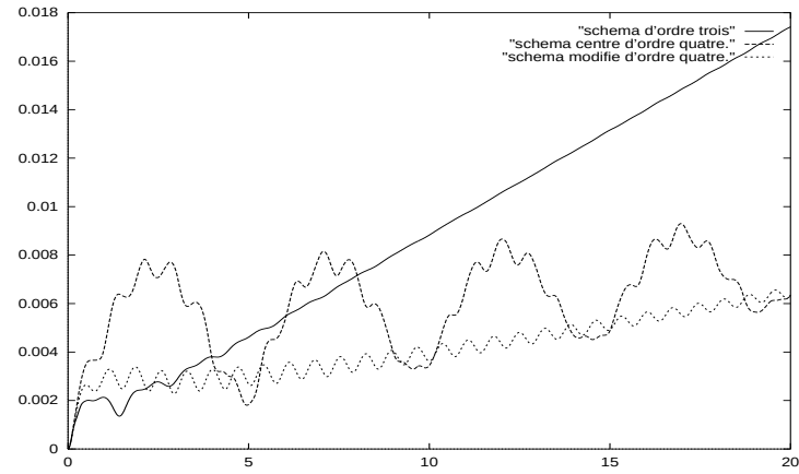
FIG. III.11 – Comparaison des schémas pour un maillage en rectangles.
