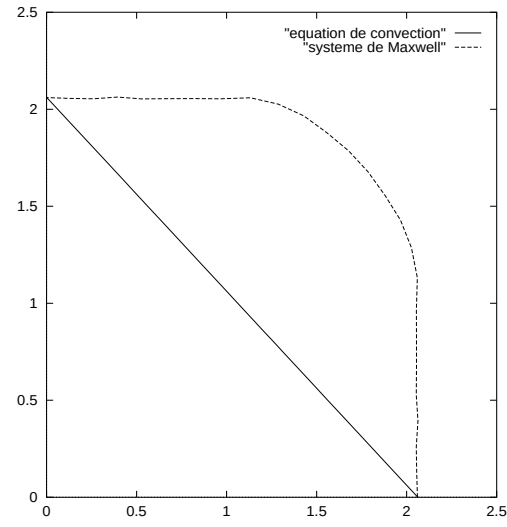
FIG. III.9 – Domaines de stabilité pour un maillage rectangulaire.
