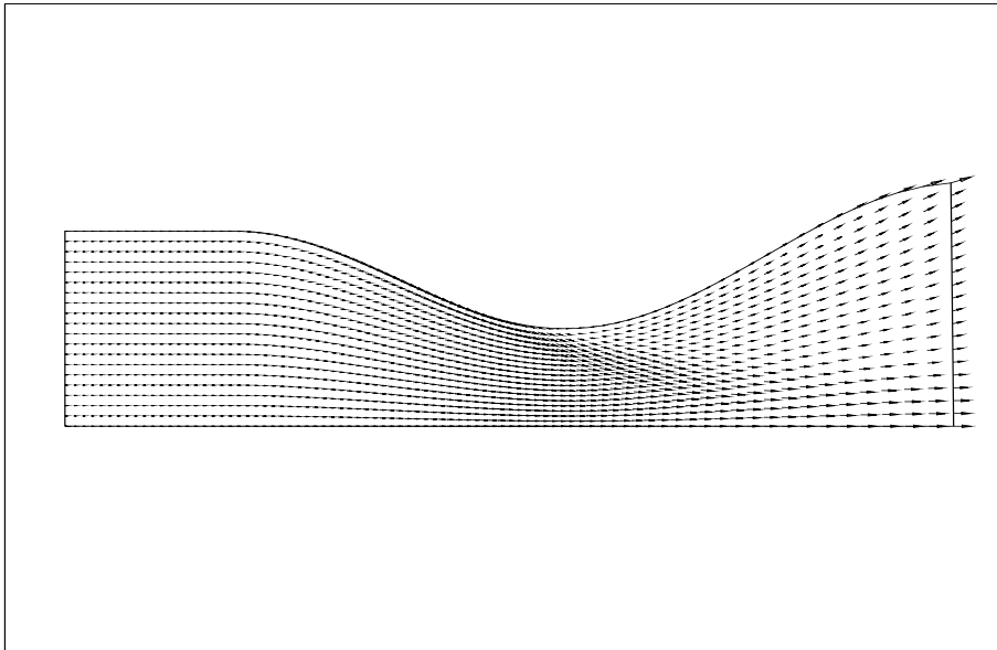
FIG. VIII.45 – Champ de vitesse des gouttes pour r = 50.10^{-6} m avec la “méthode de splitting”.
