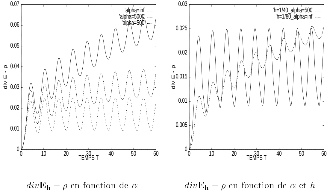
FIG. IV.15 – Influence de \alpha et de h sur la divergence.
