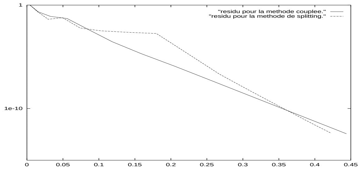
FIG. VIII.46 – Residus obtenus pour r = 1.10^{-6} m avec les deux méthodes.
