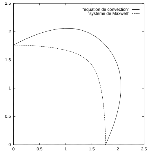
FIG. III.10 – Domaines de stabilité pour un maillage triangulaire.
