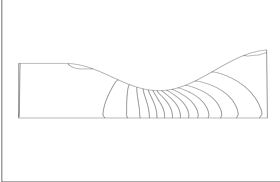
FIG. VIII.30 – Masse volumique du gaz pour r = 1.10^{-6} \text{ m} avec la “méthode couplée”.
