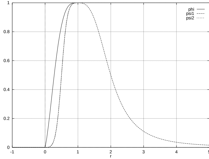
FIG. VII.4 – Limiter fonctions \varphi , \psi_1 et \psi_2 for \beta = 1/3 (VII.28).
