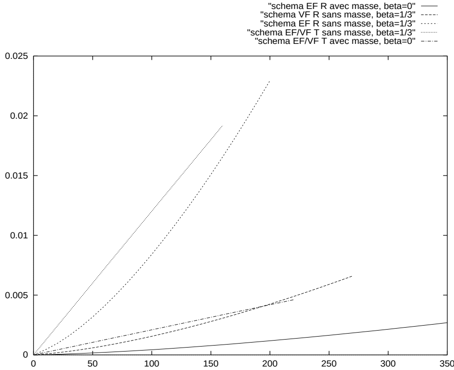
FIG. II.12 – Evolution de l'erreur E_{l_2} en fonction du nombre d'itérations pour les schémas d'ordre quatre.
