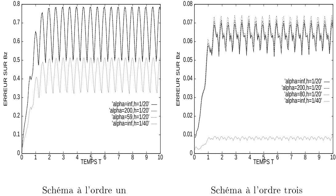
FIG. IV.12 – Erreur sur le champ magnétique pour un maillage triangulaire.
