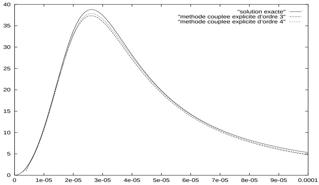
FIG. VIII.5 – Amortissement pour les “méthodes couplées” d’ordre trois et quatre.
