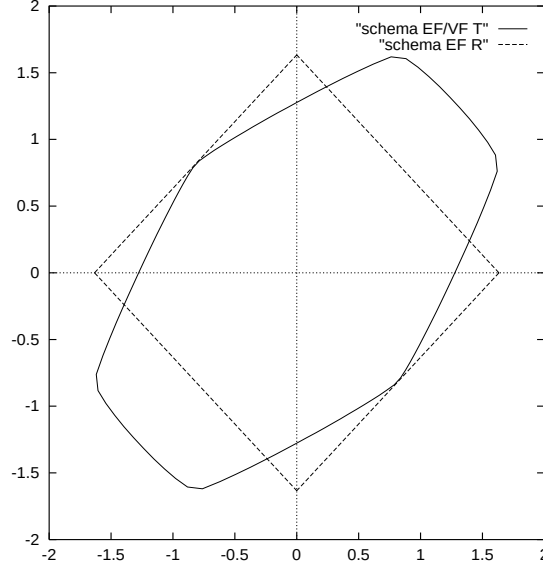
FIG. II.7 – Schémas EF R et EF/VF T avec \beta = 0 et matrice de masse en RK4.
