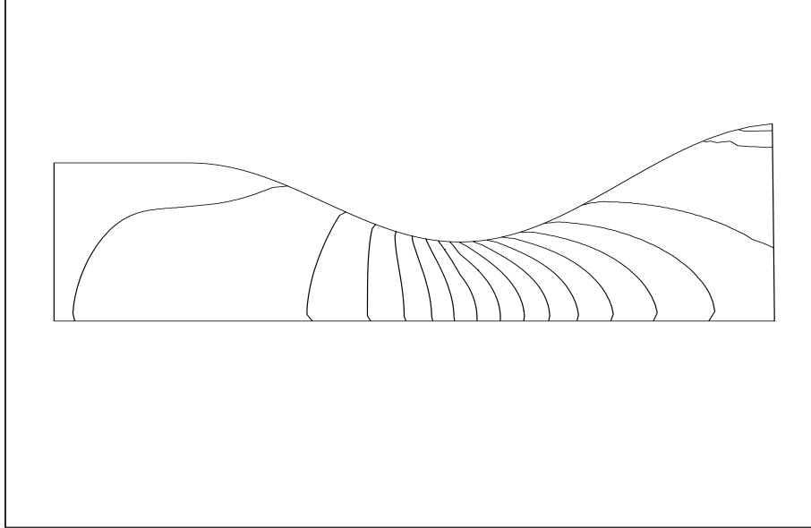
FIG. VIII.38 – Masse volumique du gaz pour r = 50 \cdot 10^{-6} \text{ m} avec la “méthode couplée”.
