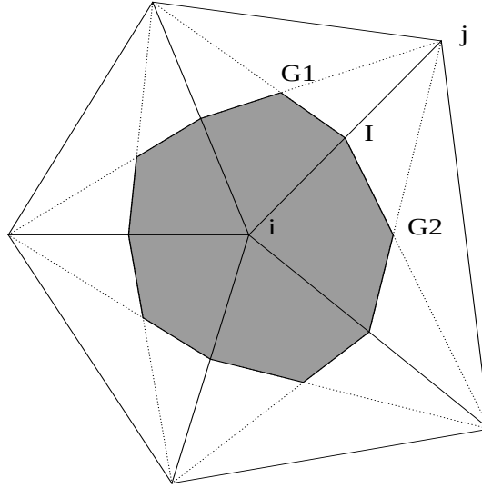
FIG. VI.1 – Construction d'une cellule pour un maillage triangulaire.
