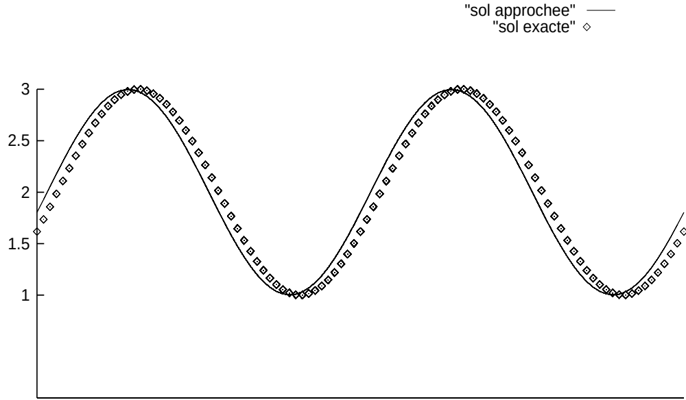
FIG. II.9 – Solution obtenue avec le schéma VF R, sans masse, \beta = 0 .
