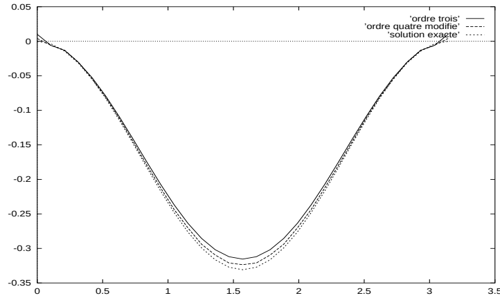
FIG. III.15 – Comparaison entre l'ordre trois et l'ordre quatre pour E_z .
