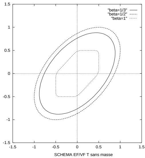
FIG. II.4 – Domaines de stabilité des schémas précis à l'ordre deux en temps
