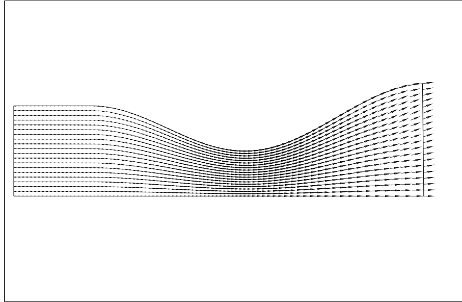
FIG. VIII.34 – Champ de vitesse du gaz pour r = 1.10^{-6} m avec la “méthode couplée”.
