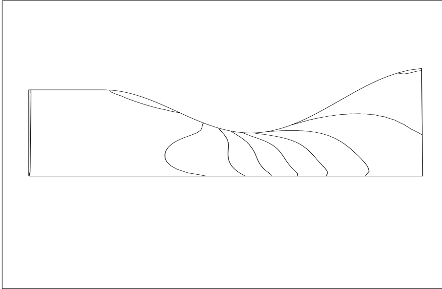
FIG. VIII.32 – Densité des gouttes pour r = 1.10^{-6} m avec la “méthode couplée”.
