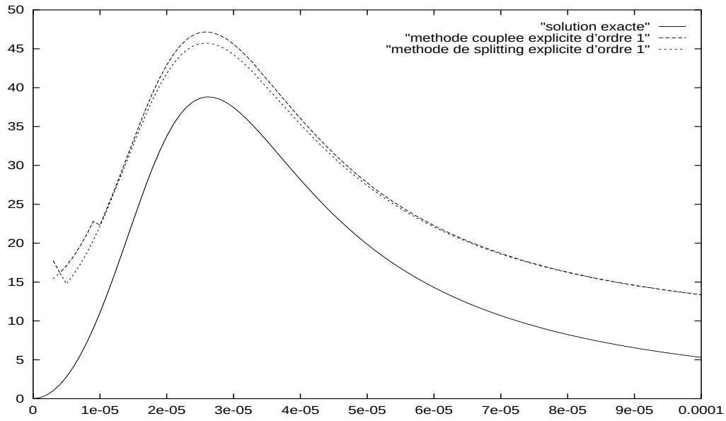
FIG. VIII.1 – Amortissement pour les méthodes d'ordre un.
