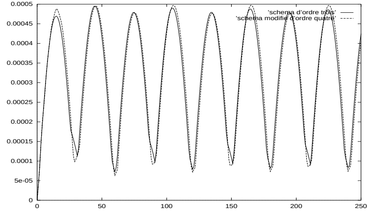
FIG. III.18 – Comparaison entre l'ordre trois et l'ordre quatre pour la divergence.
