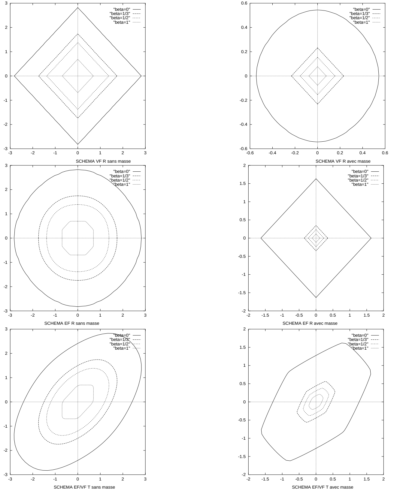
FIG. II.6 – Domaines de stabilité des schémas précis à l'ordre quatre en temps
