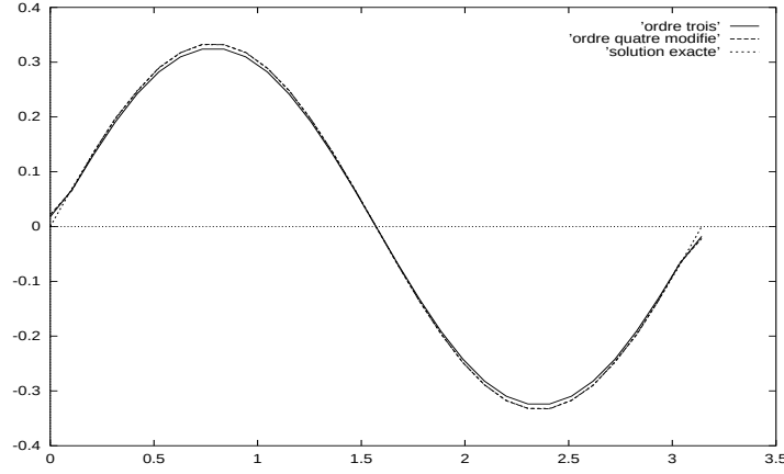
FIG. III.14 – Comparaison entre l'ordre trois et l'ordre quatre pour B_x .
