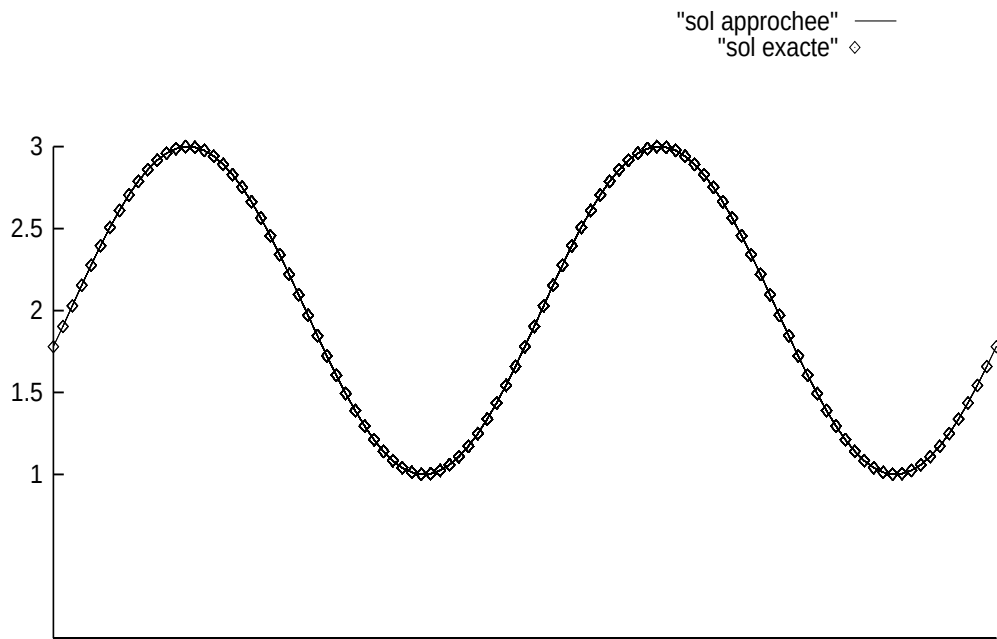
FIG. II.11 – Solution obtenue avec le schéma EF R, avec masse, \beta = 0 .
