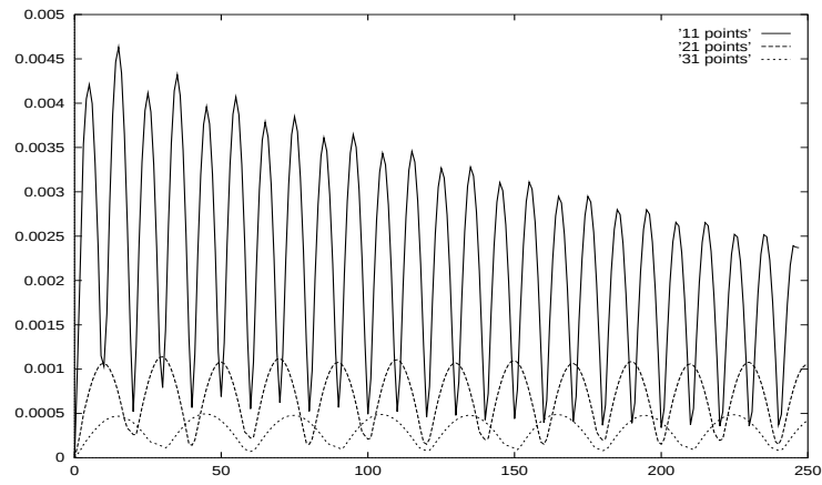
FIG. III.16 – Influence du pas de maillage sur la divergence pour les schémas d'ordre trois.
