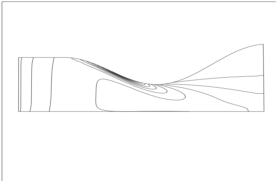
FIG. VIII.40 – Densité des gouttes pour r = 50.10^{-6} m avec la “méthode couplée”.
