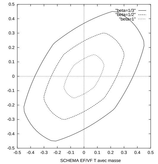
FIG. II.4 – Domaines de stabilité des schémas précis à l'ordre deux en temps
