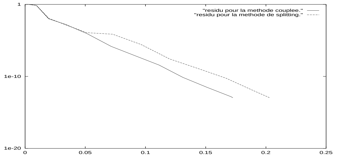
FIG. VIII.47 – Residus obtenus pour r = 50.10^{-6} m avec les deux méthodes.
