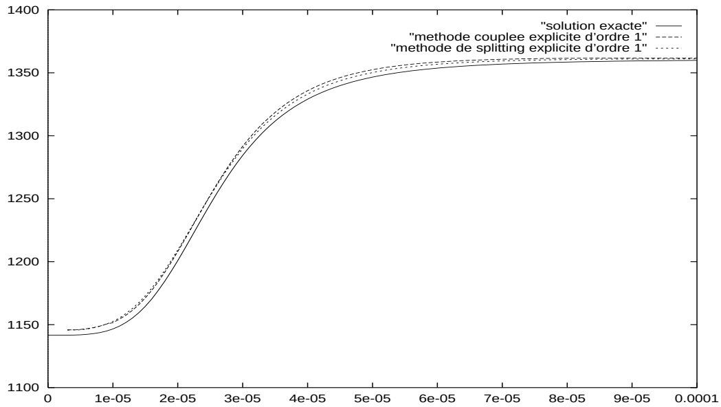
FIG. VIII.2 – Vitesse du son pour les méthodes d'ordre un.
