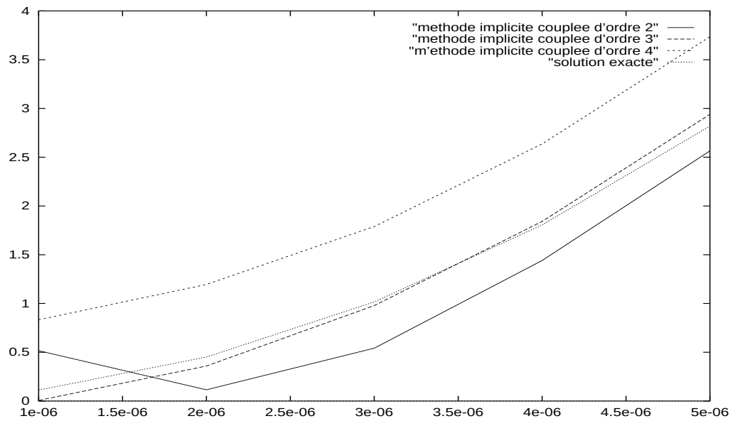
FIG. VIII.10 – Amortissement pour les schémas de Cranck-Nicolson d'ordre deux, trois, quatre en espace appliqués à la "méthode couplée".
