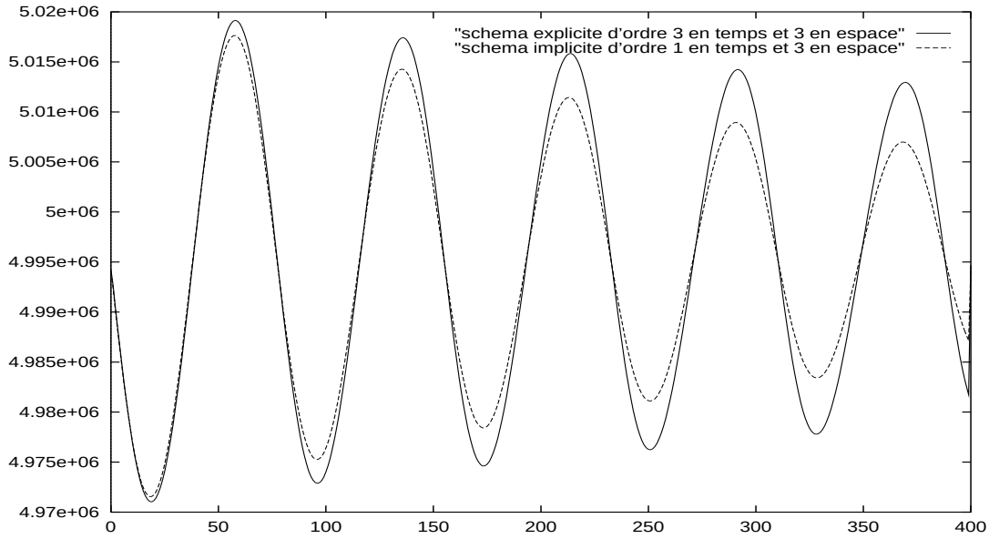
FIG. VIII.7 – Comparaison entre le schéma implicite d'ordre un en temps et le schéma explicite d'ordre trois en temps avec la “méthode couplée” pour r = 1.10^{-4} m .
