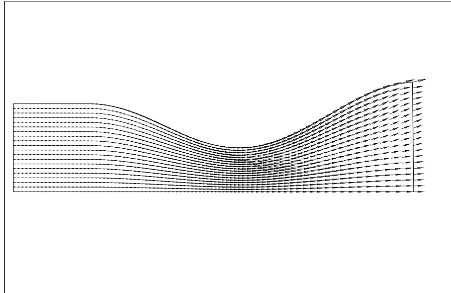
FIG. VIII.35 – Champ de vitesse du gaz pour r = 1.10^{-6} m avec la “méthode de splitting”.
