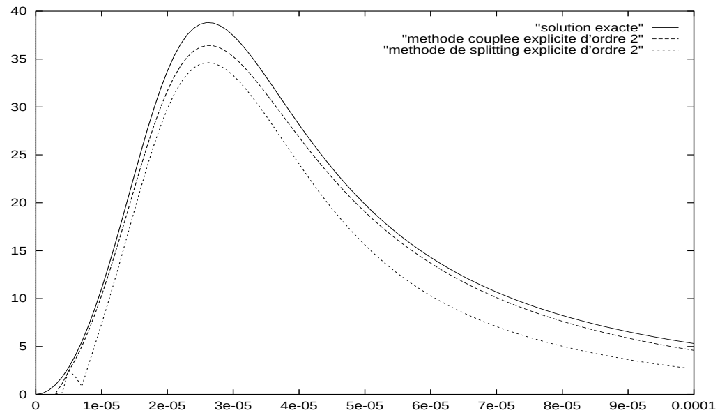
FIG. VIII.3 – Amortissement pour les méthodes d'ordre deux.
