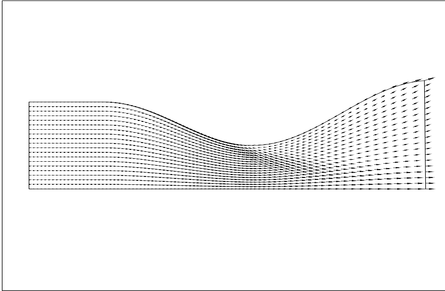
FIG. VIII.44 – Champ de vitesse des gouttes pour r = 50.10^{-6} m avec la “méthode couplée”.
