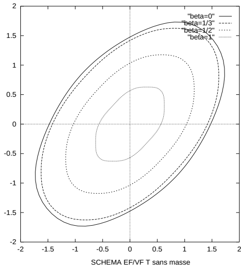
FIG. II.5 – Domaines de stabilité des schémas précis à l'ordre trois en temps
