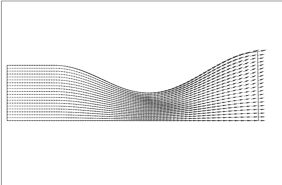
FIG. VIII.37 – Champ de vitesse des gouttes pour r = 1.10^{-6} m avec la “méthode de splitting”.
