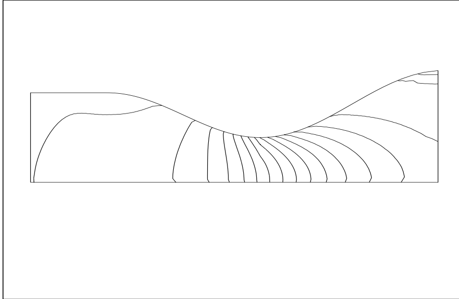
FIG. VIII.39 – Masse volumique du gaz pour r = 50 \cdot 10^{-6} \text{ m} avec la “méthode de splitting”.
