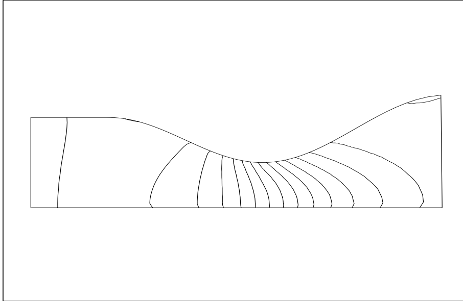
FIG. VIII.31 – Masse volumique du gaz pour r = 1.10^{-6} \text{ m} avec la “méthode de splitting”.
