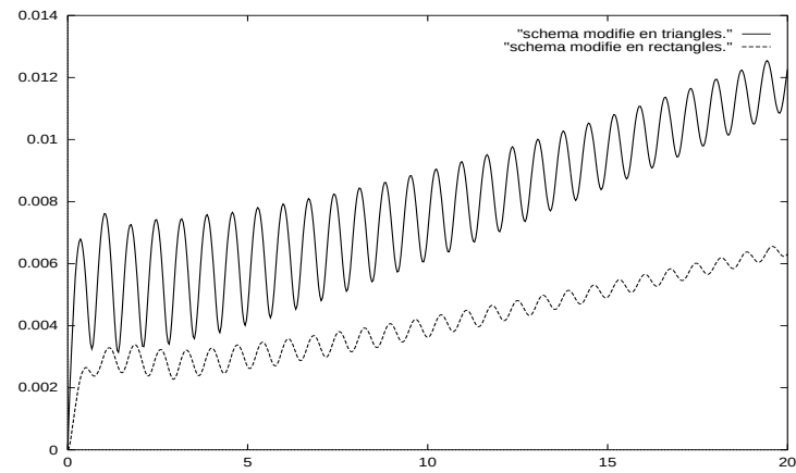
FIG. III.13 – Comparaison entre le maillage en rectangles et celui en triangles .
