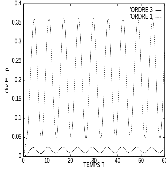
FIG. IV.16 – Comparaison entre les schémas d'ordre un et trois.
