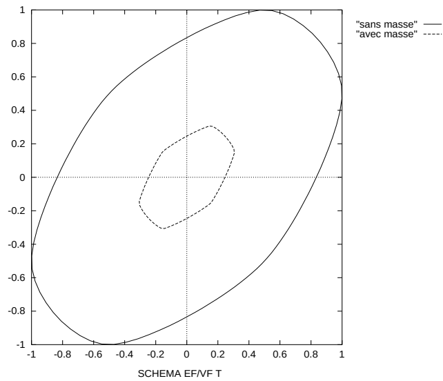
FIG. II.3 – Domaines de stabilité des schémas avec et sans matrice de masse.
