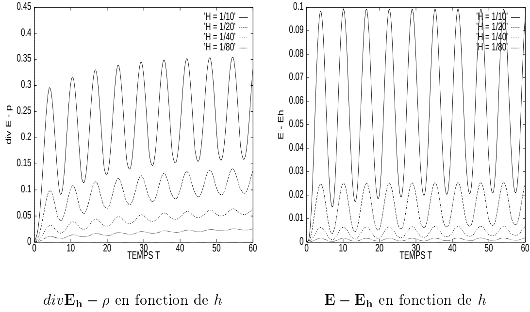
FIG. IV.14 – Influence du pas de maillage h .
