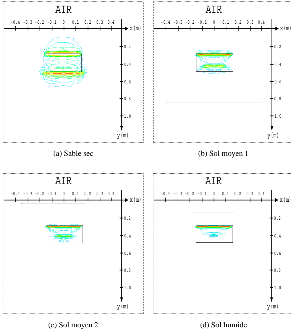
FIG. 3.7 – Reconstructions d'un diélectrique pur enterré dans différents sols
