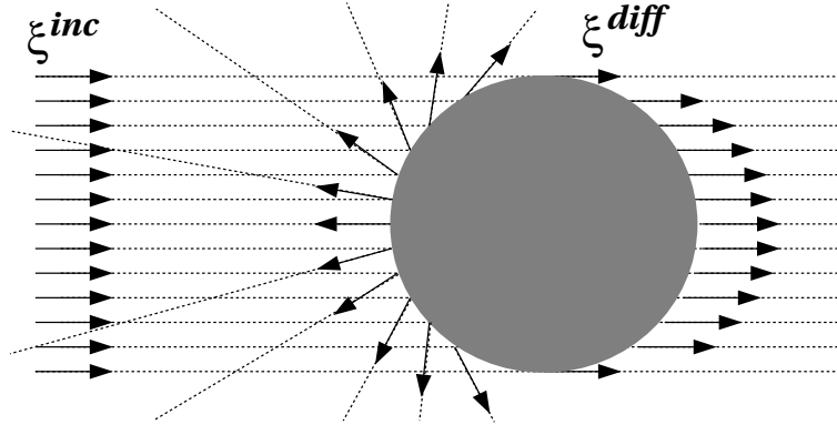
FIG. 5.6: Représentation des vecteurs diffractés \xi^{diff} résultants du vecteur d'onde \xi^{inc}
