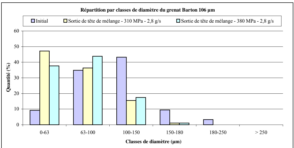
Graph 10 : Evolution granulométrique du grenat Barton 106 µm en fonction de la pression d'eau
