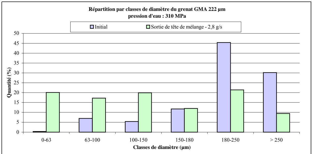
Graph 18 : Evolution granulométrique du grenat GMA 222 μm pour une pression d'eau de 310 MPa
