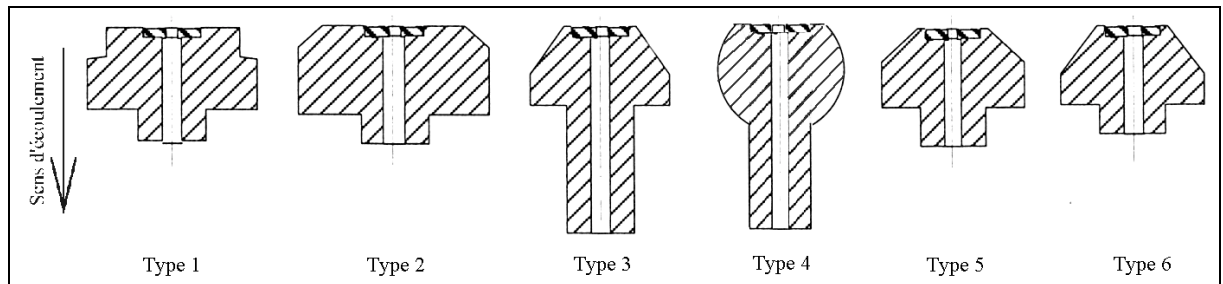
Figure 2 : Buses de découpe
