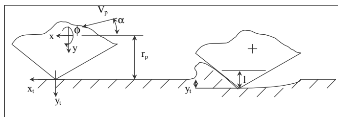
Figure 8 : Enlèvement de matière par une particule
