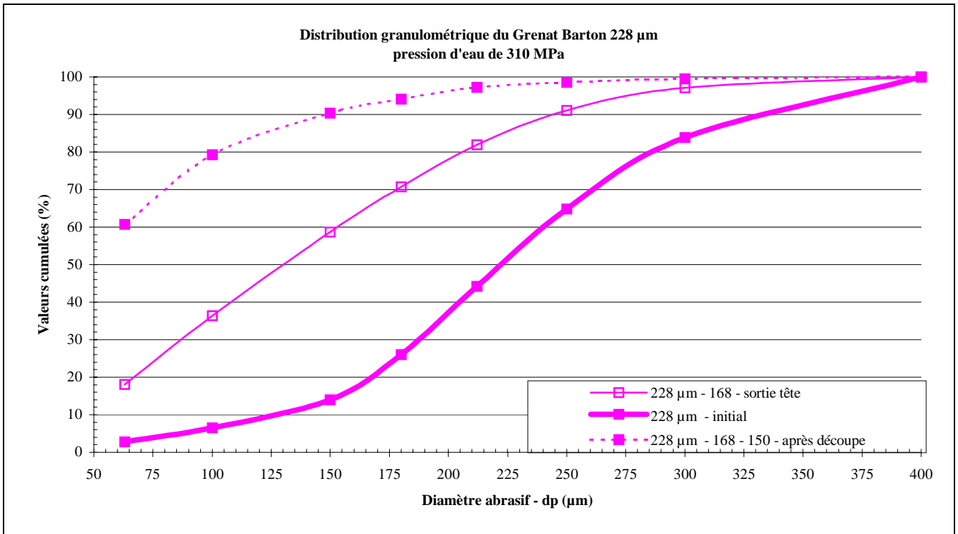
Grphe A . 6 : Evolution granulométrique d'un grenat Barton 228 μm pour une pression d'eau de 310 MPa
