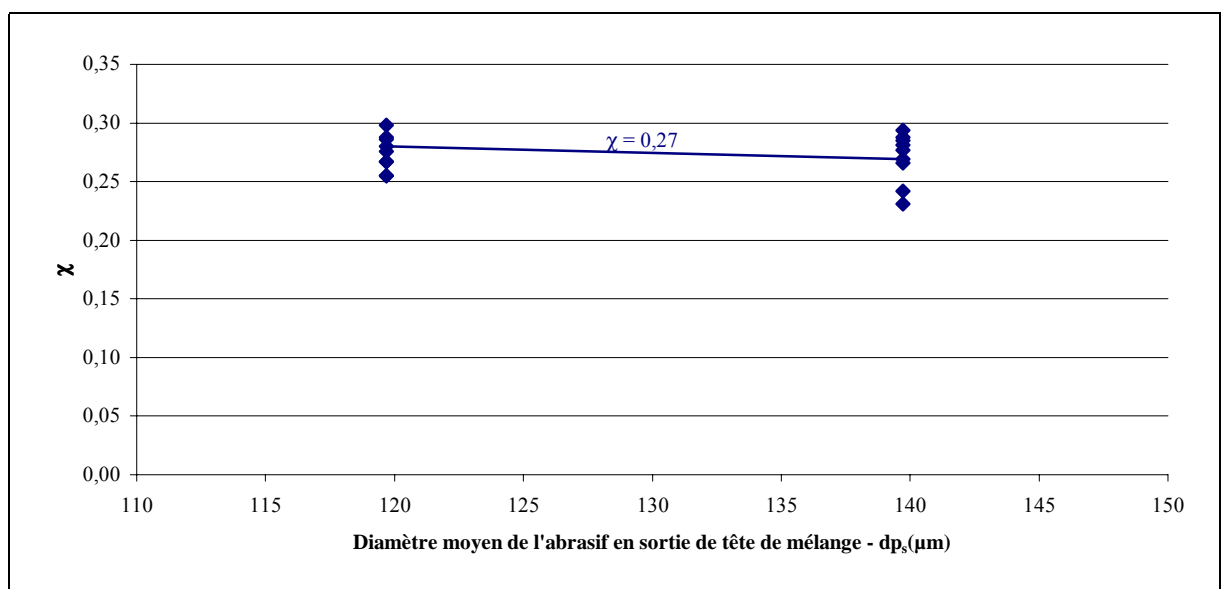
Graph 23 : Evolution de \chi en fonction du diamètre de l'abrasif en sortie de tête de mélange
