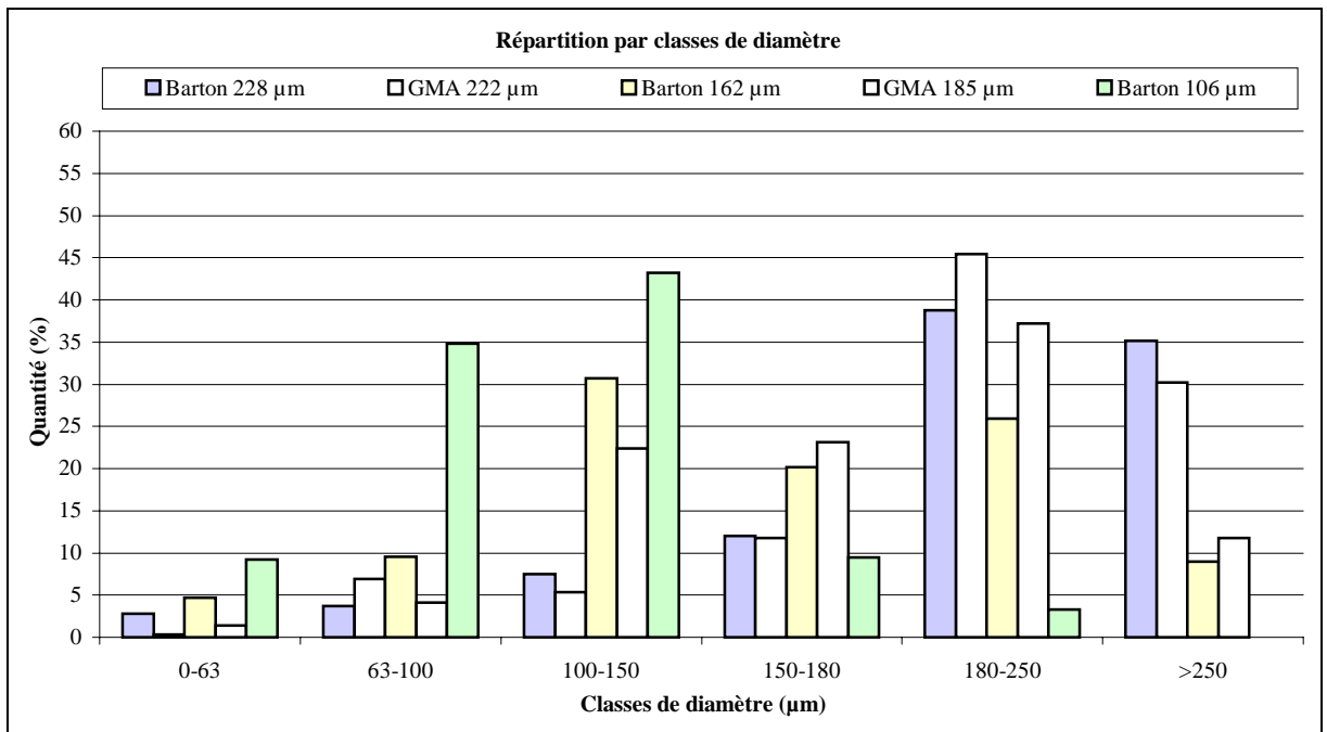
Graph A . 1 : Répartition granulométrique initiale des particules abrasives
