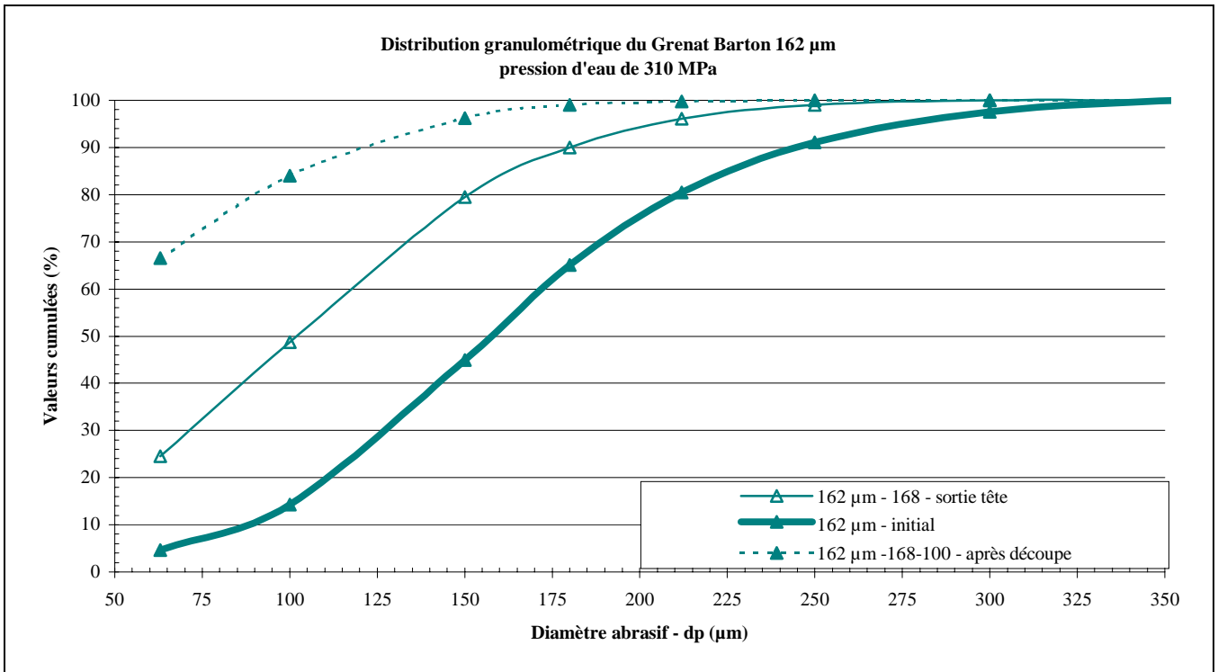
Graphe A . 7 : Evolution granulométrique d'un grenat Barton 162 μm pour une pression d'eau de 310 MPa
