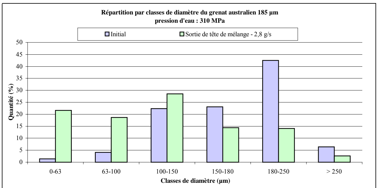
Graph 19 : Evolution granulométrique du grenat GMA 185 μm pour une pression d'eau de 310 MPa
