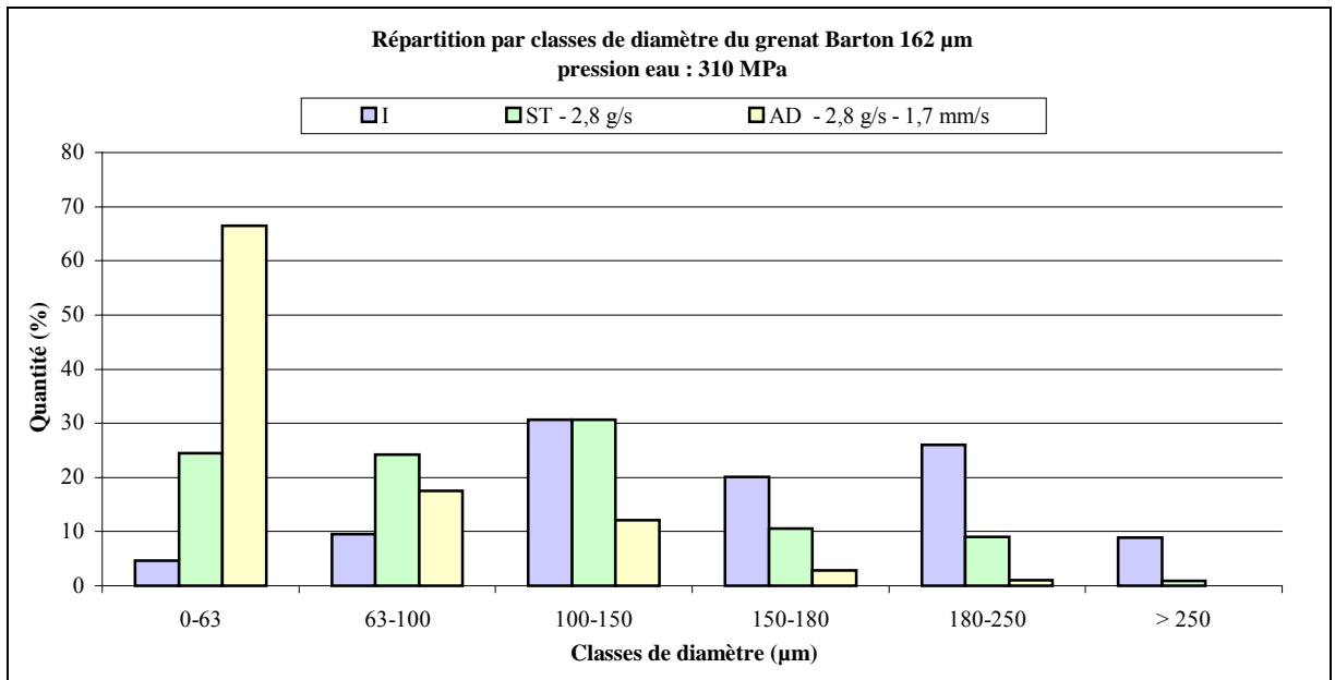
Graphe 5 : Evolution granulométrique du grenat Barton 162 \mu\text{m} - pression d'eau : 310 MPa
