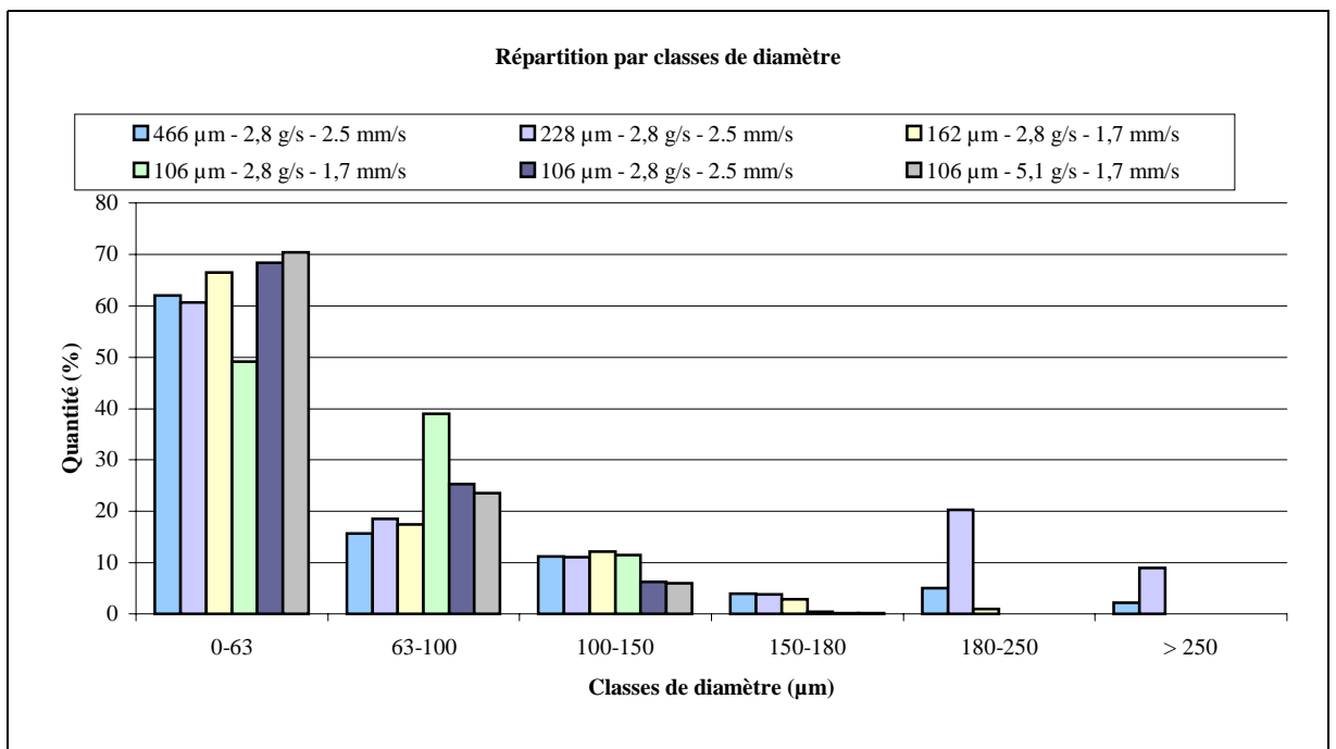
Graph A . 3 : Répartition granulométrique des particules abrasives après découpe
