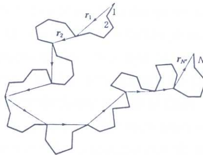
Figure I.10 Chaîne polymère de N segments rigides (—) et chaîne équivalente de Kuhn (→) (Doi, 1996)
