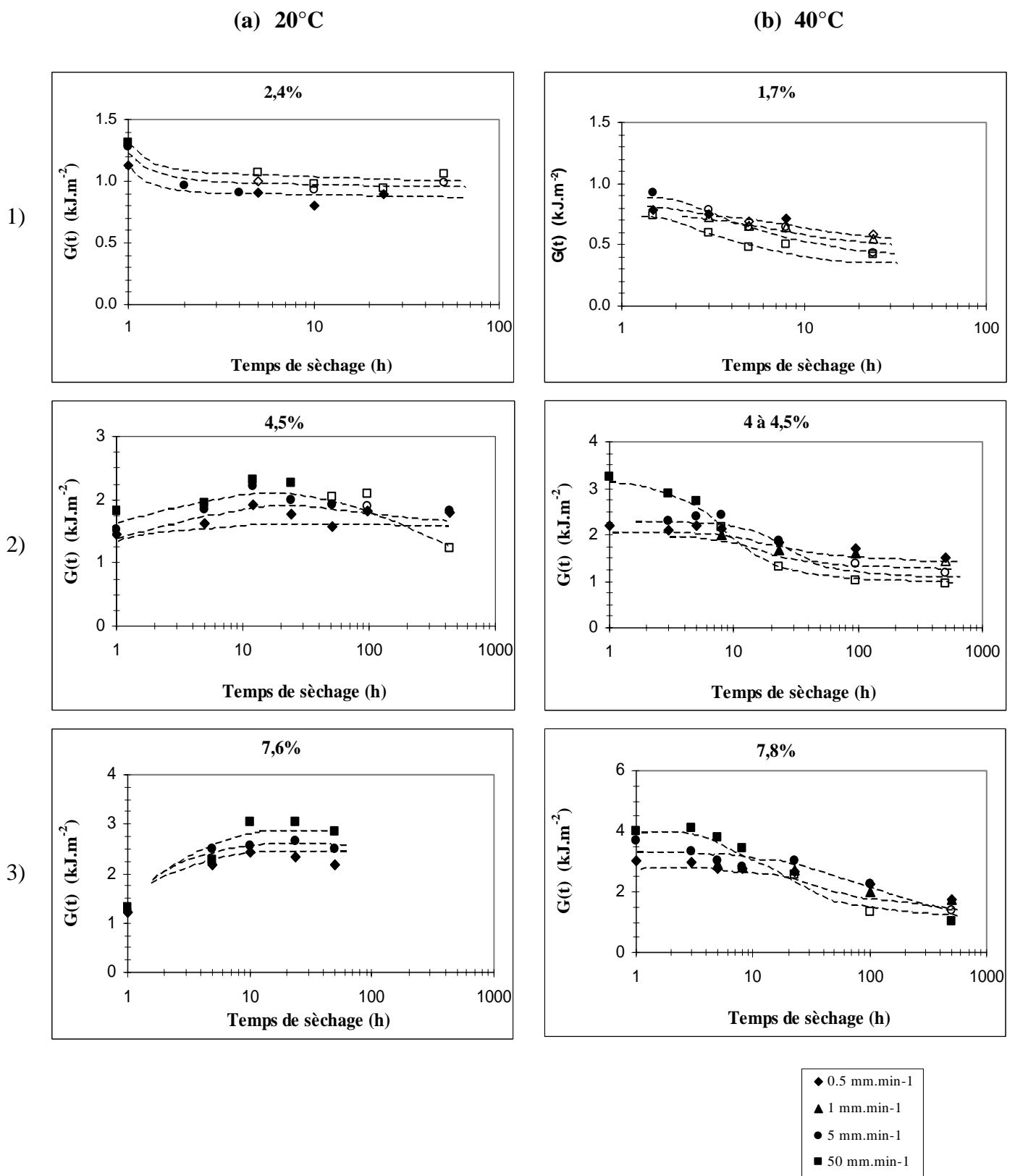
Figure III.29 Energie à rupture en fonction du temps de séchage a) à 20°C pour 4 vitesses de pelage b) à 40°C pour 4 vitesses de pelage
