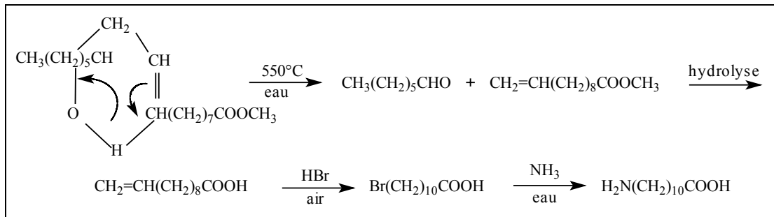
Figure I.1 Synthèse de l'acide \omega -amino undécanoïque (Kohan, 1973)
