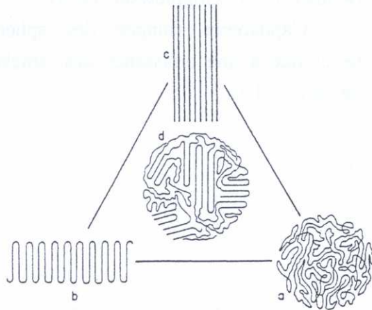
Figure I.3 Conformations possibles d'une macromolécule linéaire (Van Krevelen, 1990)
