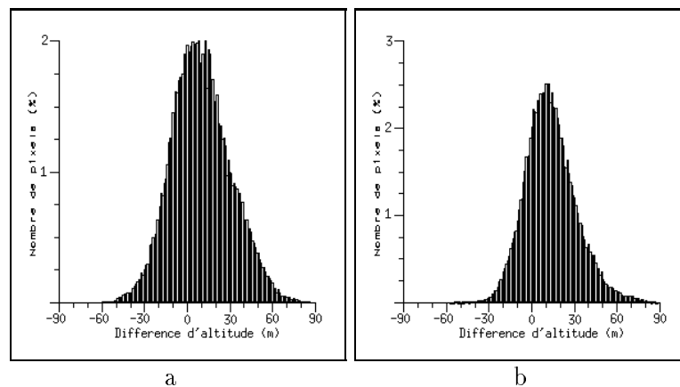
FIG. 6.5 – Exemples d'histogramme de différence entre deux cartes d'altitude restituées par radarcinométrie à partir d'images radar différentes (en a : ERS-1 (22°) - RADARSAT (25°), et en b : JERS-1 (36°) - RADARSAT (32°)).
