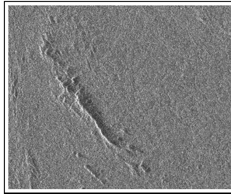
FIG. B.15 – Images radar ERS-1 d'une région sud du Cameroun. Le couvert végétal y apparaît très homogène ce qui remplit une des conditions d'utilisation de notre procédé de restitution.
