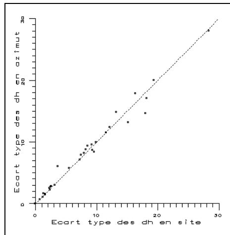
FIG. 4.4 – Ecart type des différences d'altitude estimées pour divers modèles numériques de terrain et suivant deux directions perpendiculaires entre elles (site/azimut).
