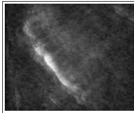
FIG. B.17 – Relief final obtenu à partir de l'image radar (Fig B.15), et résultant du processus markovien initialisé par la carte d'altitude figurant en (Fig B.16).
