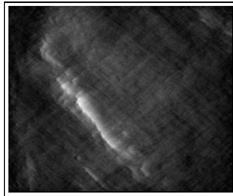
FIG. B.16 – Relief obtenu à partir de l'image radar (Fig B.15), et par une simple intégration en ligne suivant diverses directions de part et d'autre de l'axe en site. Cette carte relativement proche de la réalité permet l'initialisation du procédé markovien.
