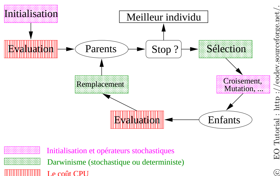
FIG. 1.8 – Schéma général d'un algorithme évolutionnaire.
