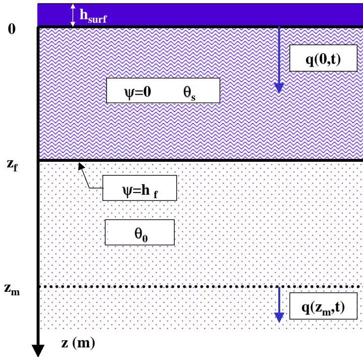
FIG. D.1: Schéma de l'infiltration dans un sol selon Green et Ampt (1911)
