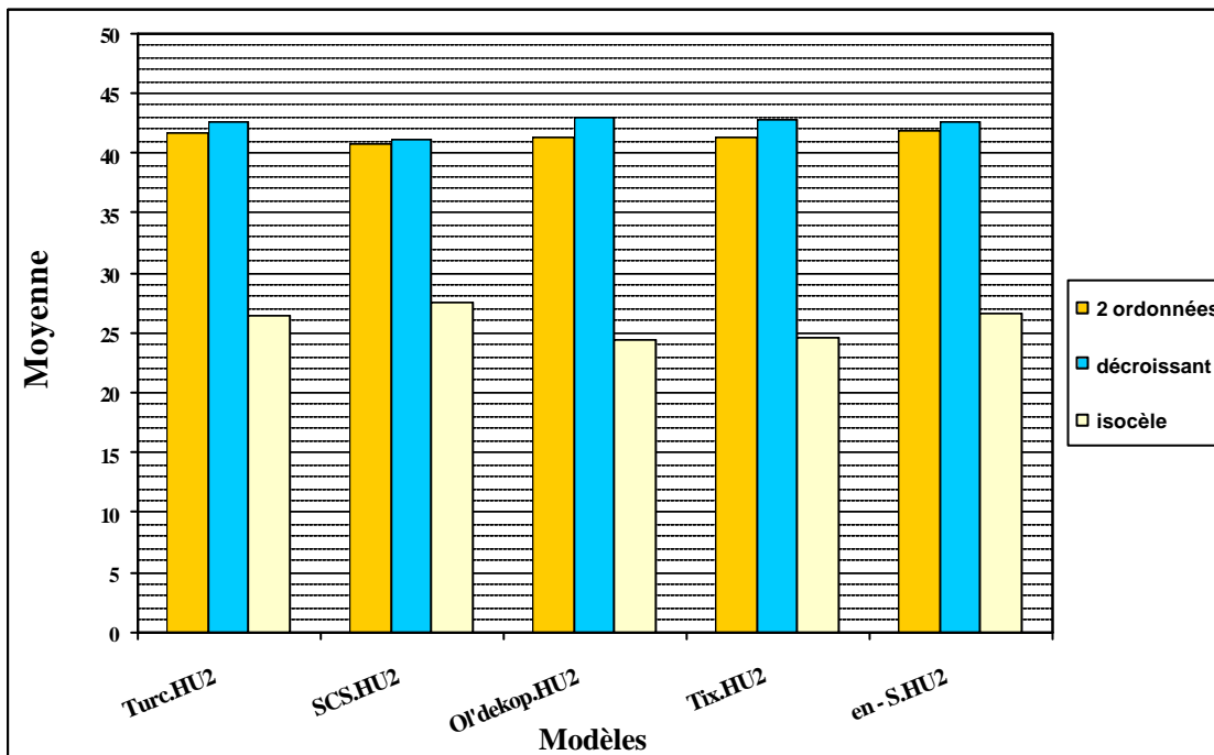
Figure 65 : Test de l'architecture III (Hydrogramme Unitaire) : a) selon le critère Cr3 ; b) selon le critère 'moyenne' des Nash
