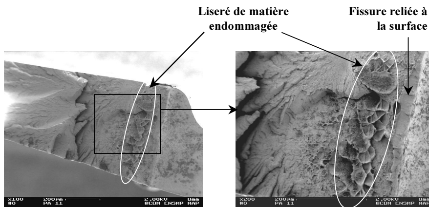
Figure III.28 : Observation après cryofractographie de l'endommagement du PA 11 vieilli en service. On observe le liseré de matière endommagé ainsi qu'une fissure débouchant à la surface.
