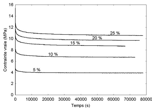
Figure V.3 : Courbes de relaxation du PA 11 neuf sous 4 valeurs de déformations nominales imposées : 5%, 10%, 15%, 20% et 25%. Si le PA 11 avait un comportement viscoélastique, la contrainte asymptotique de l'essai soumis à 20% de déformation devrait être le double de celle correspondant à l'essai sous 10% de déformation.
