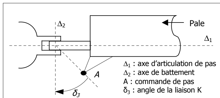
Figure I.7 : Liaison K
