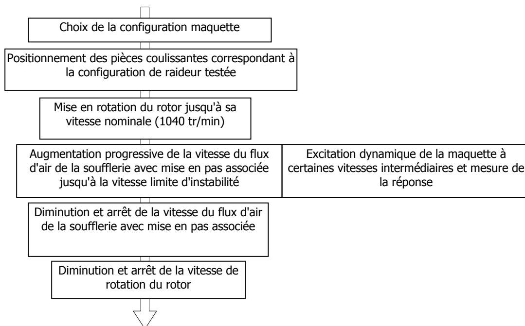
Figure IV.1 : Procédure d'essais
