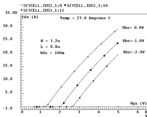
a : caractéristiques I_{\text{DS}} = F(V_{\text{cgs}}) La courbe neutre à V_{\text{BS}} = 0\text{V}
