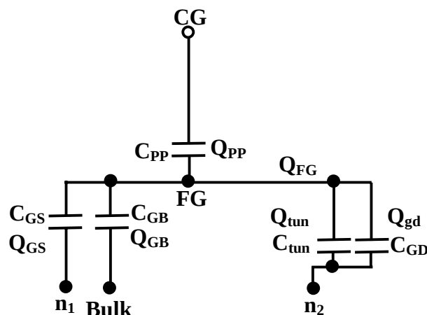
Figure 3-9 : Modèle capacitif du transistor MOS à grille flottante.
