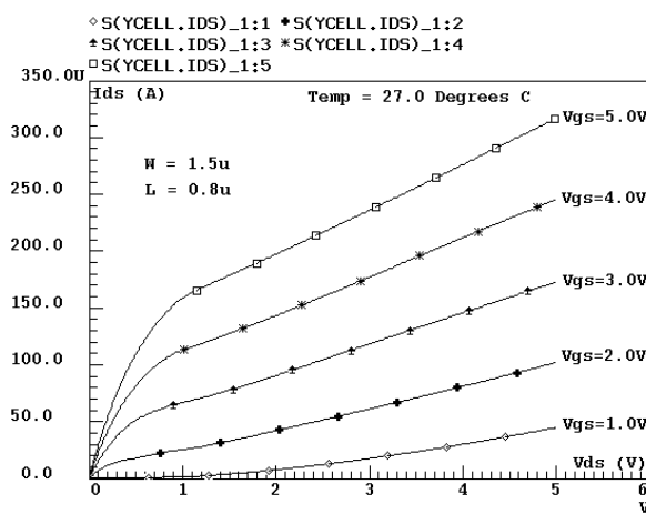
b : caractéristiques I_{\text{DS}} = F(V_{\text{ds}})
