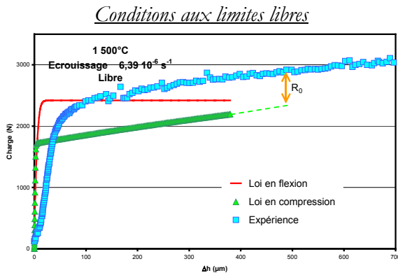
Figure 7.37 - Simulation d'essai de compression à vitesse de déformation imposée à 1500°C.
