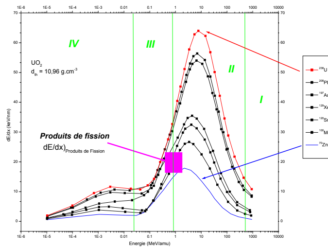
Figure 9.1 - Pertes d'énergie de différents ions dans \text{UO}_2 .
