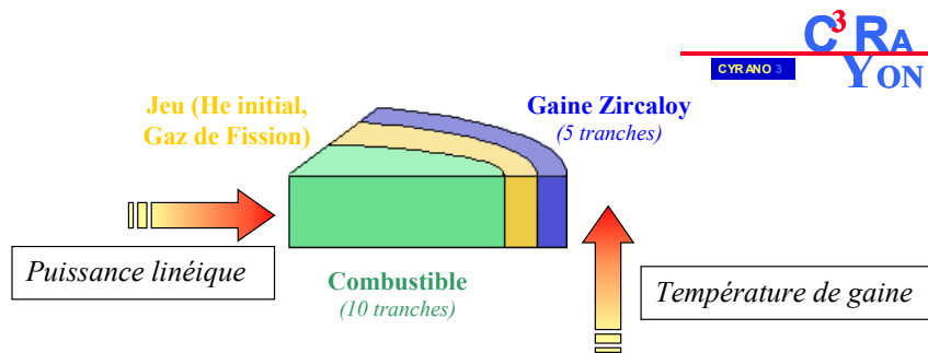
Figure 4.1 - Principe de fonctionnement du logiciel CYRANO3 avec les conditions aux limites en températures et en puissance.
