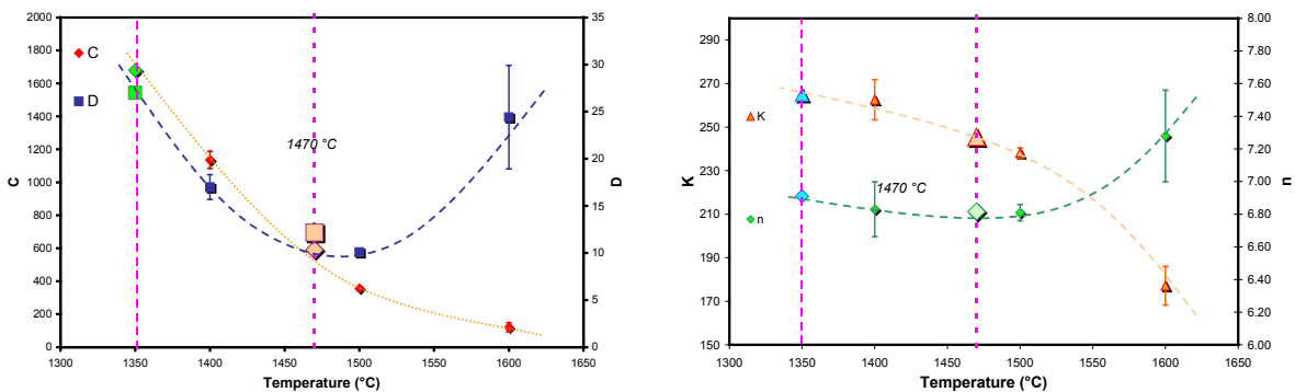
Figure 7.38 – Extrapolation à 1350°C des coefficients de la loi identifiée en compression.
