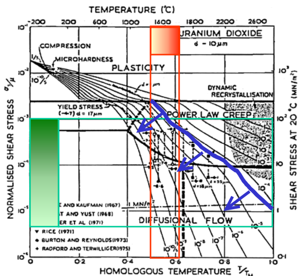
Figure 6.37 - Superposition de nos essais avec la carte de fluage d'Ashby.
