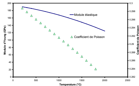
Figure 8.14 - Module d'élasticité et coefficient de Poisson de UO_2 .
