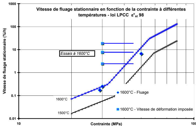
Figure 7.8 - Base d'essais à 1600^{\circ}\text{C} en compression, superposition avec la loi LPCC.
