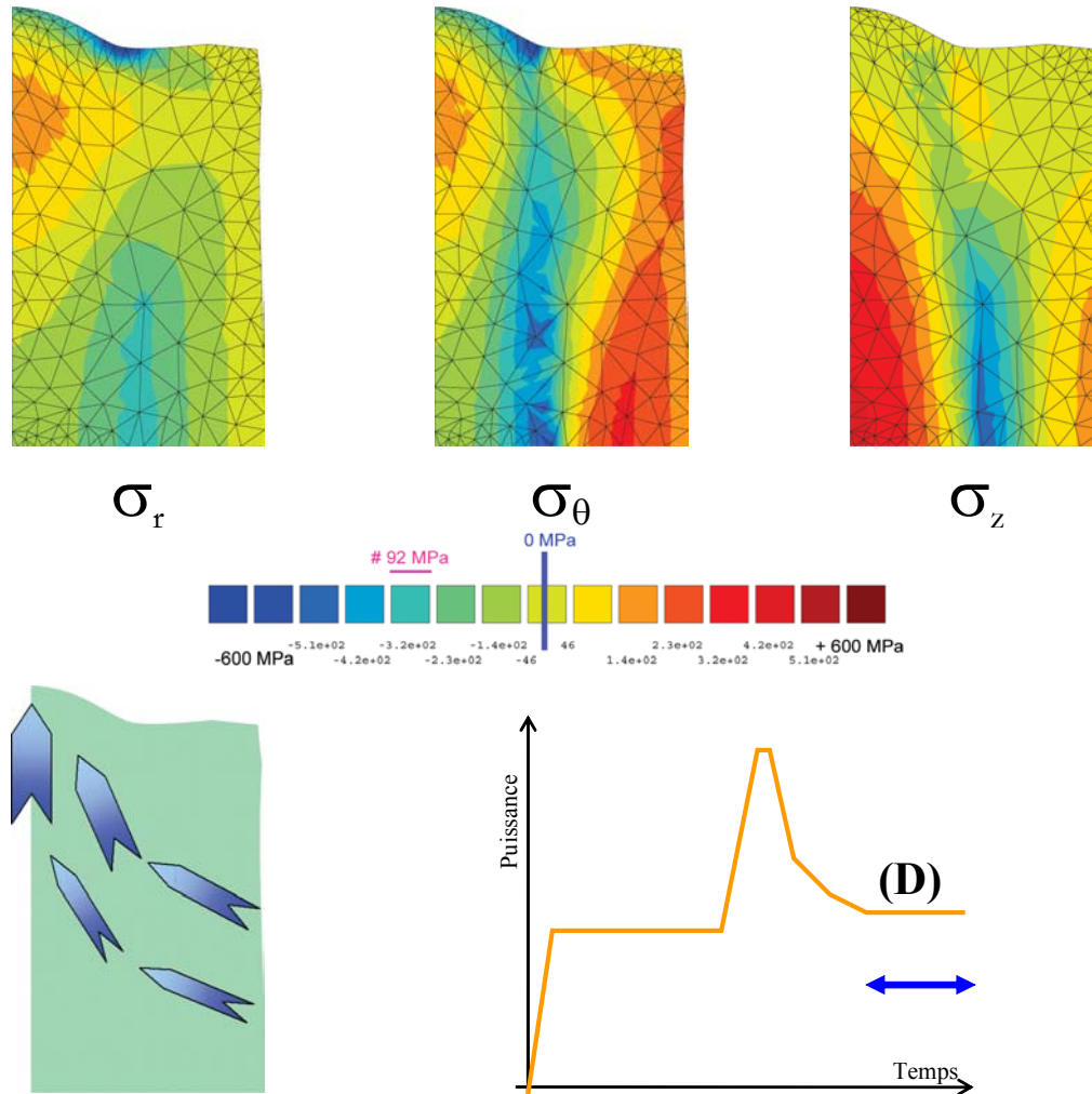
Figure 8.21 - Association des contraintes et des déformations subies par le combustible après un transitoire de puissance : retour au régime de base.
