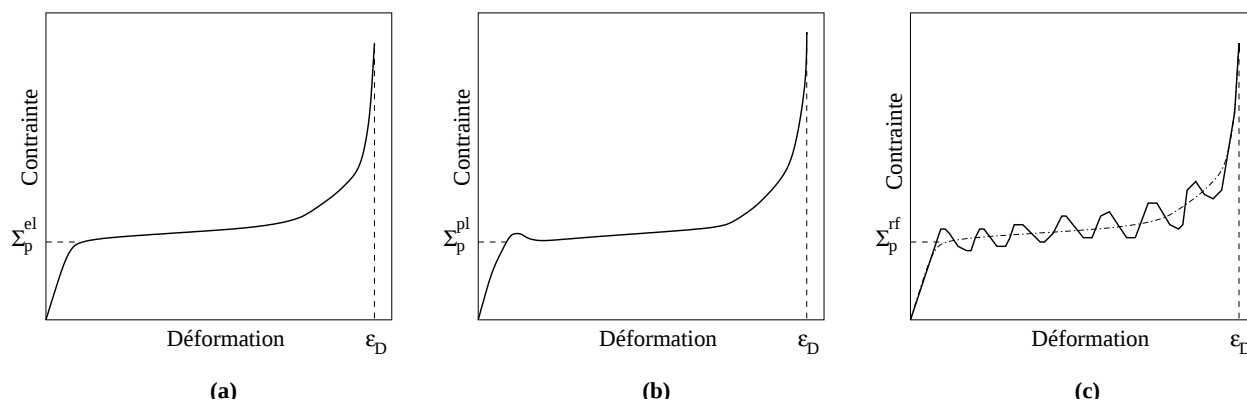
FIG. 1.7 – Courbes contrainte-déformation schématiques de mousses en compression uniaxiale : (a) mousse élastomérique ; (b) mousse élasto-plastique ; (c) mousse élastique fragile
