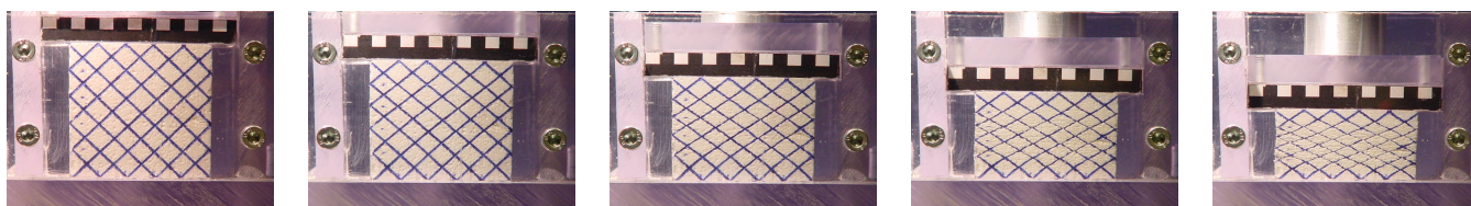
FIG. 10.9 – Essai de compression biaxiale sur une mousse de caril
