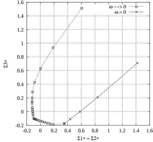
FIG. 9.5 – Surfaces de charge des modes périodiques ou à grandes longueurs d'onde dans le plan \Sigma_1 = \Sigma_2
