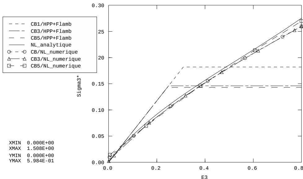
FIG. 7.1 – Courbes contrainte adimensionnelle-déformation des CB, CB3 et CB5 en compression uniaxiale
