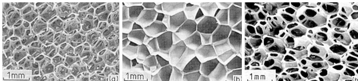
FIG. 1.2 – Trois types de matériaux cellulaires tridimensionnels [Gibson et Ashby, 1988] : (a) polyuréthane à porosité ouverte; (b) polyéthylène à porosité fermée; (c) polyéther à cellules ouvertes et fermées
