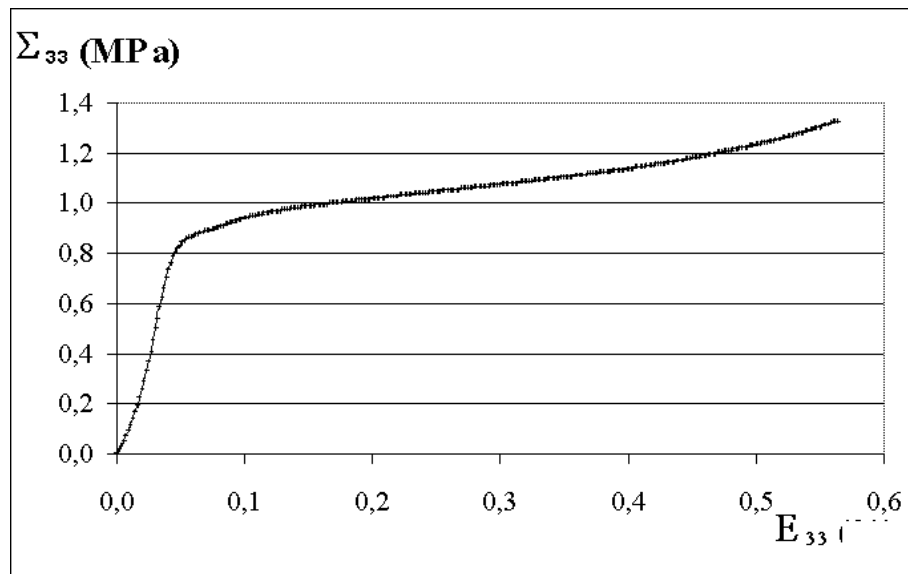
FIG. 10.6 – Exemple de courbe contrainte-déformation nominales
