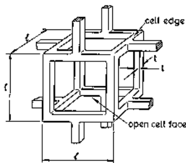
FIG. 3.3 – Première cellule de base adoptée par Gibson et ses collaborateurs
