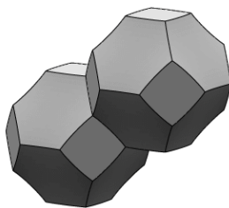
FIG. 2.3 – Partition de Kelvin : les tétrakaidécaèdres [Thomson, 1887]
