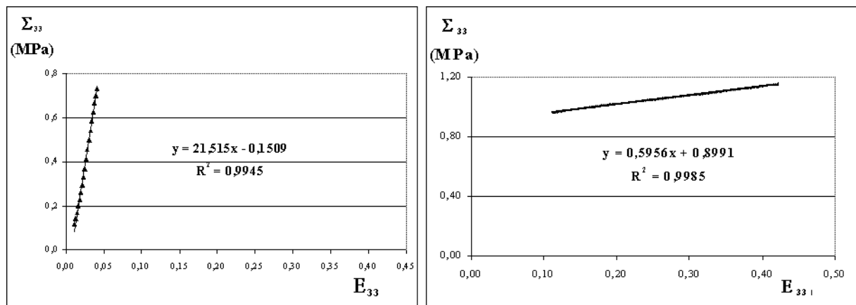
FIG. 10.7 – Linéarisation des deux premières phases de l'exemple de courbe contrainte-déformation nominales
