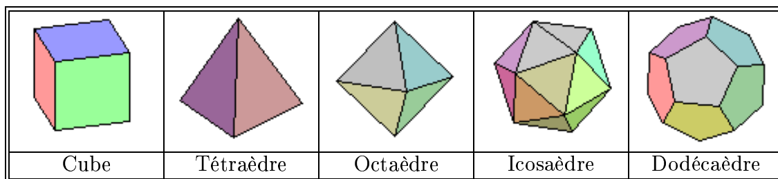
FIG. 2.1 – Les cinq solides platoniciens
