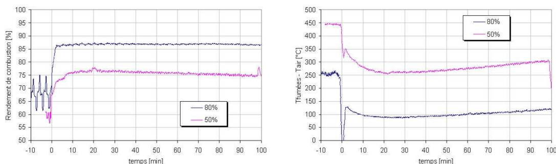
Figure 3.38 – Influence du taux d'aspiration sur (a) le rendement de combustion du four et (b) sur la différence de température entre l'air préchauffé et les fumées.
