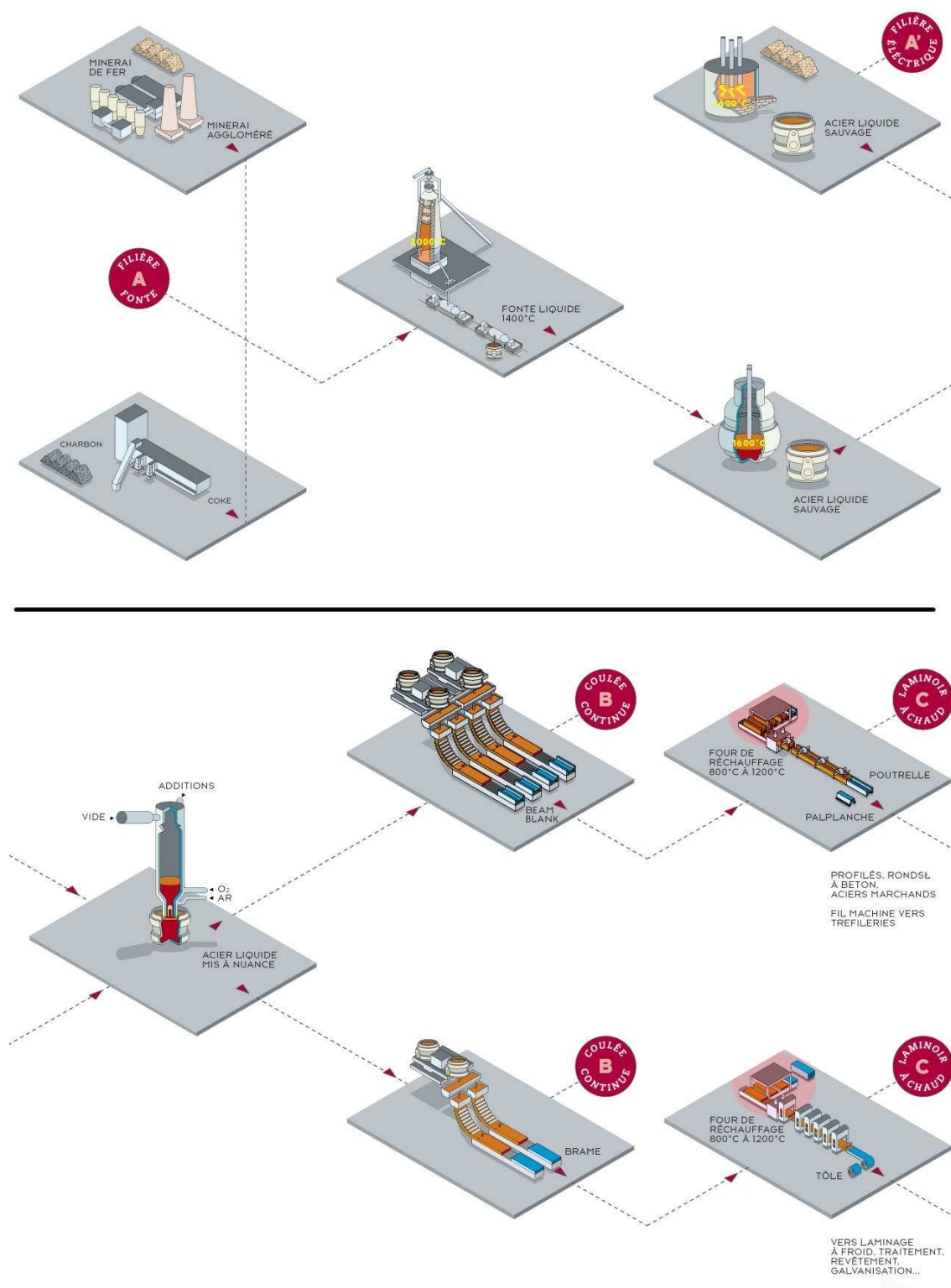
Figure 1.1 – Process de fabrication de l'acier (document Arcelor).
