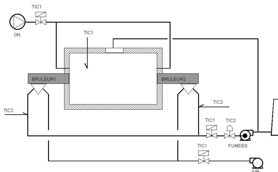
Figure 3.33 – Schéma fluidique incluant la régulation en température des fumées.
