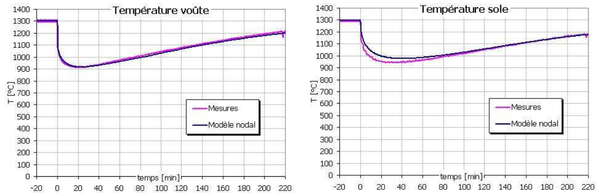
Figure 3.65 – Essai n°1 : comparaison du calcul des températures de parois avec les mesures.
