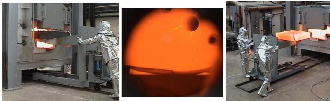
Figure 3.29 – (a) Enfournement de la brame. (b) Réchauffage de la brame par les brûleurs. (c) Défournement de la brame.
