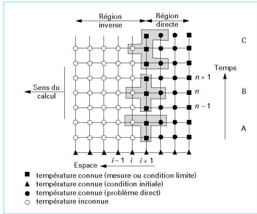
Figure I.3 – Molécule de calcul des températures dans la zone inverse.
