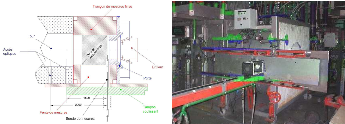
Figure 2.11 – Cellule d’essais de Gaz de France.
