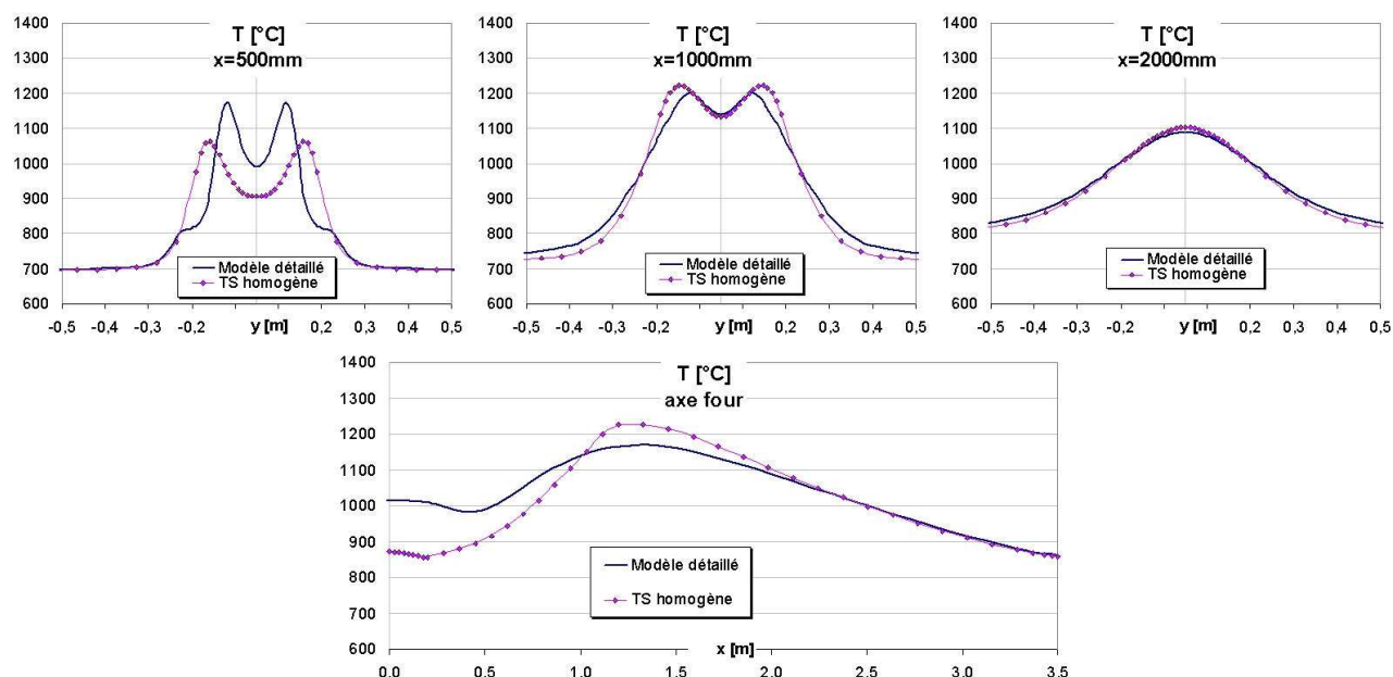
Figure 2.34 – Comparaison du modèle détaillé et du modèle simplifié avec terme source homogène sur le champ de température.
