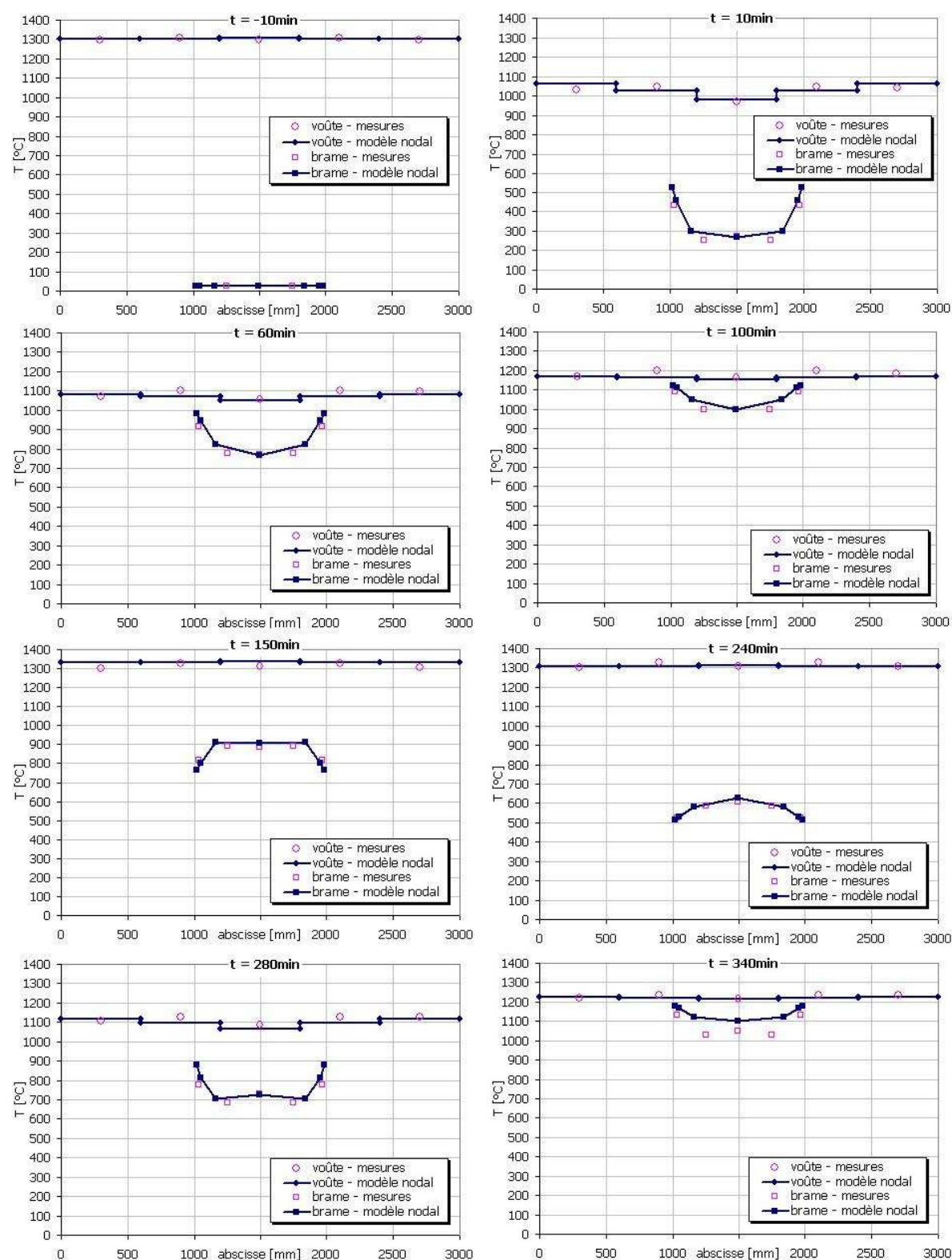
Figure 3.78 – Essai n°2 : comparaison du calcul de l'hétérogénéité thermique avec les mesures.
