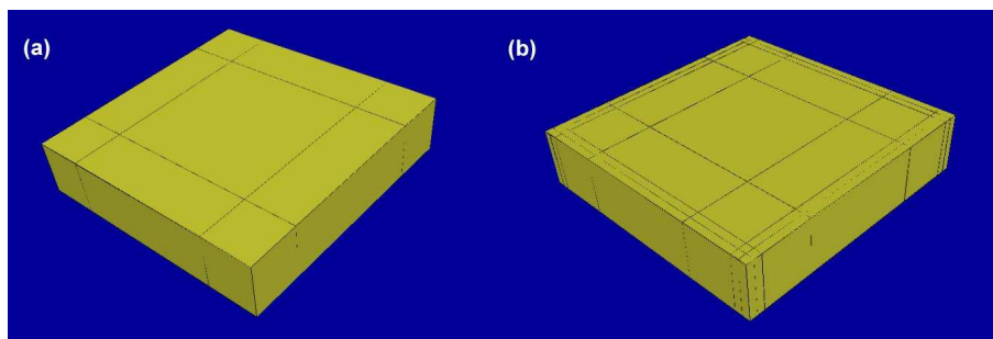
Figure 3.49 – Discrétisation de la charge : (a) 3 \times 3 branches. (b) 7 \times 7 branches.
