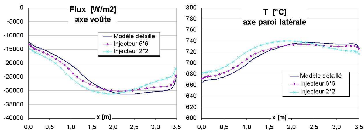
Figure 2.41 – Comparaison des maillages sur les échanges thermiques en paroi.
