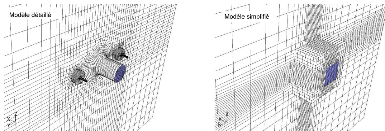
Figure 2.29 – Maillages utilisés pour les modèles détaillés et simplifiés.
