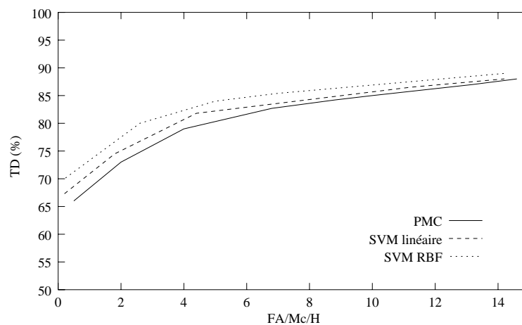
FIG. 7.9 – Courbes ROC obtenues par une représentation vectorielle mixte.
