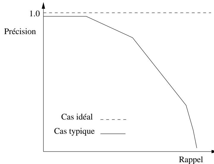
FIG. 4.6 – Courbes rappel/précision
