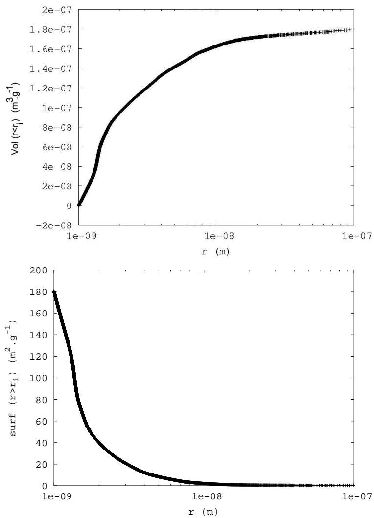
FIG. 5.15 – Volume cumulé V(r) (en haut) et surface S(r) (en bas) pour la désorption
