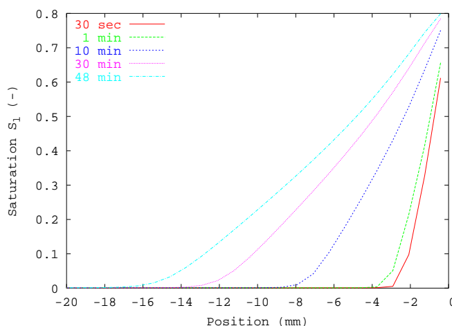
FIG. 9.1 – Evolution de la saturation dans le milieu poreux au cours du temps
