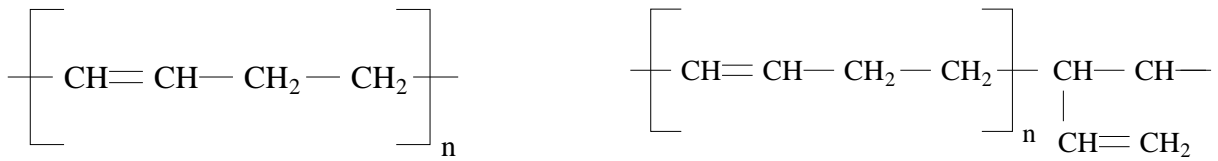
FIG. 1.7 – La molécule de polybutadiène et le cas d'une configuration vinyl
