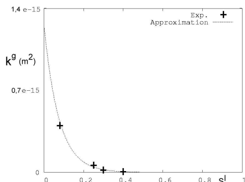
FIG. 7.7 – K^g(S^l) expérimental et approximation par la relation (7.43)
