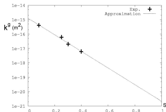
FIG. 7.8 – K^g(S^l) expérimental et approximation par la relation (7.43) (échelle logarithmique)
