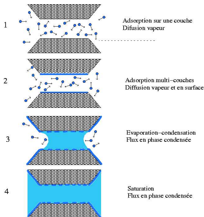
FIG. 5.4 – Mécanisme de la sorption
