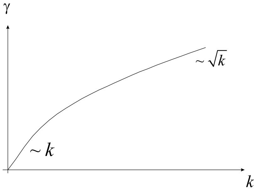
Fig.2. Taux de croissance de l'instabilité.
