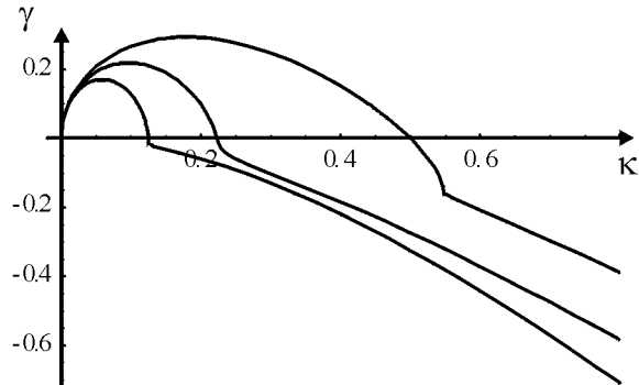
Fig. 4. Courbes de taux de croissance \gamma(\kappa) pour quelques valeurs du paramètre \xi_0 \Omega \rho^{1/3} / (\eta^{1/3} g^{1/3}) , obtenues à partir de l'équation (35) (en variables adimensionnelles).
