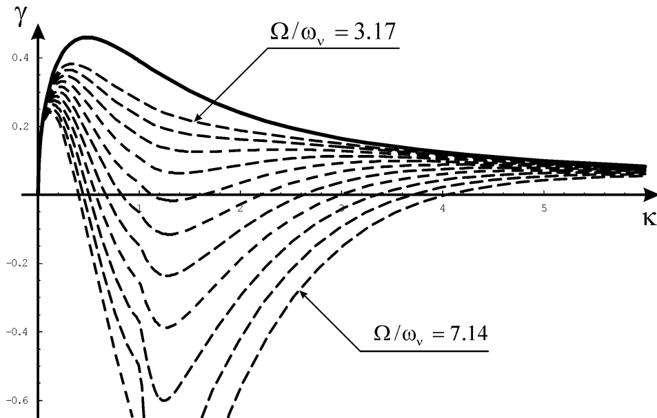
Fig.6. Courbes de dispersion de l'instabilité Rayleigh-Taylor pour différentes valeurs de \Omega/\omega_v variants de 3.17 à 7.14, le pas étant de 0.4. \xi_0 k_v = const = 0.4
