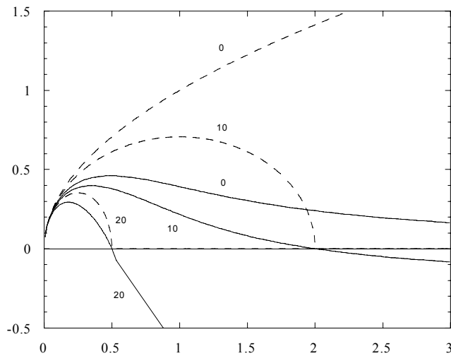
Fig. 4a. Un exemple de la fonction \gamma(\kappa) pour une limite de petite amplitude et grande fréquence, le nombre d'onde est petit. Ici \xi_0 k_v = 0.1 ( (\xi_0 k)_{\max} = 0.3 ). Les lignes solides représentent les solutions de l'équation (36), lignes en pointillées sont les solution de l'équation (37). Les nombres correspondent aux différentes valeurs de \Omega / \omega_v .
