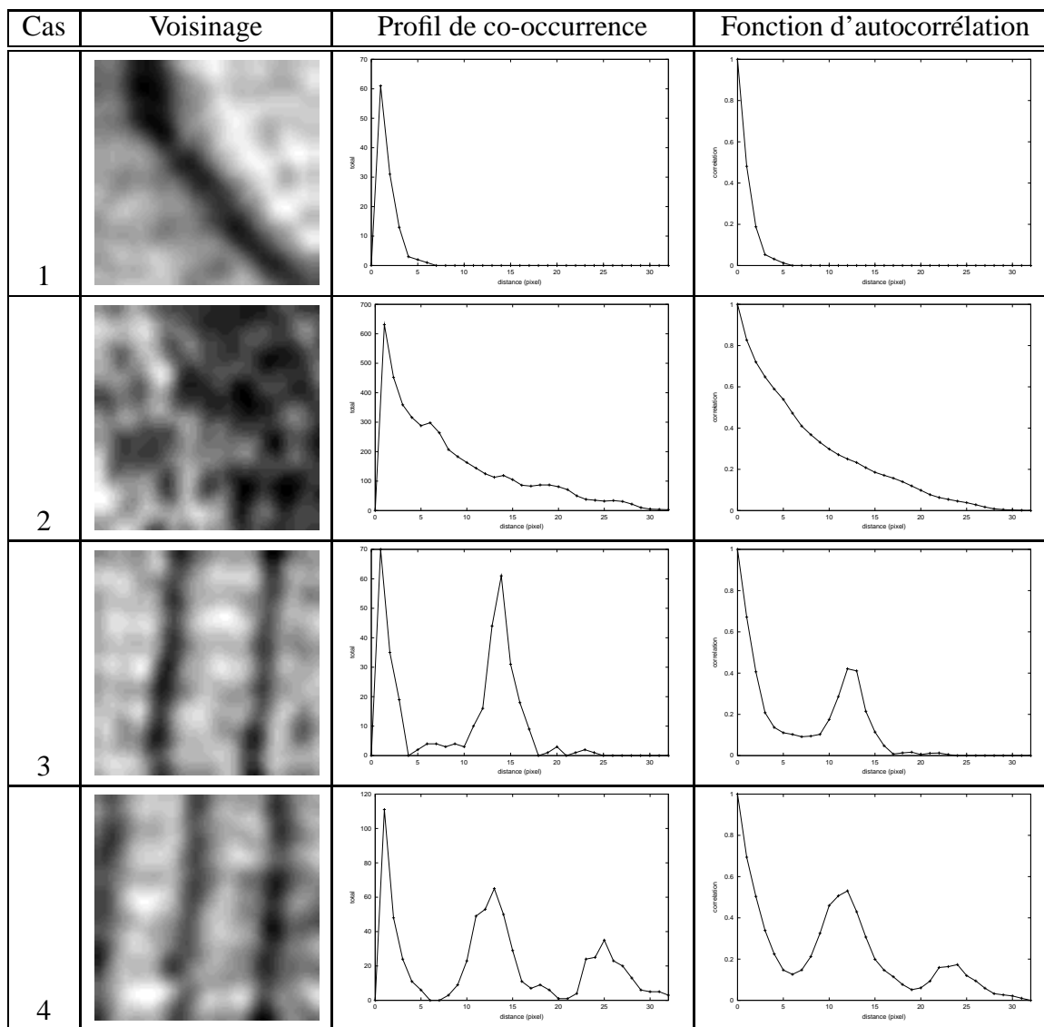
FIG. 9.7. – Les quatre cas de classement des profils de co-occurrence. Pour chaque cas y figure : le voisinage de l'image, le profil de co-occurrence et la fonction d'autocorrélation.
