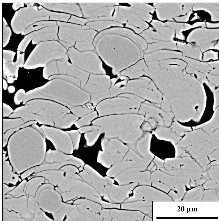
Figure III.1 : Micrographie MEB d'une coupe transversale d'un dépôt obtenue par la projection de la poudre \text{Al}_2\text{O}_3[-25 +10 \mu\text{m}] avec le plasma HPPS-12,5 kW et une distance de projection de 130 mm.
