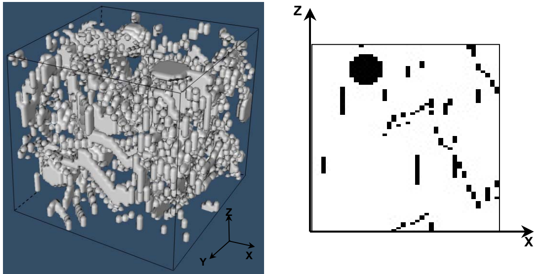
Figure V.43 : Simulation de la porosité totale dans un cube de 20 \times 20 \times 20 \mu\text{m}^3 (somme des images a, b et c de la Figure V.42). Visualisation de l'image 3D (à gauche) et d'une coupe particulière ( Y = 3 \mu\text{m} ) (à droite).
