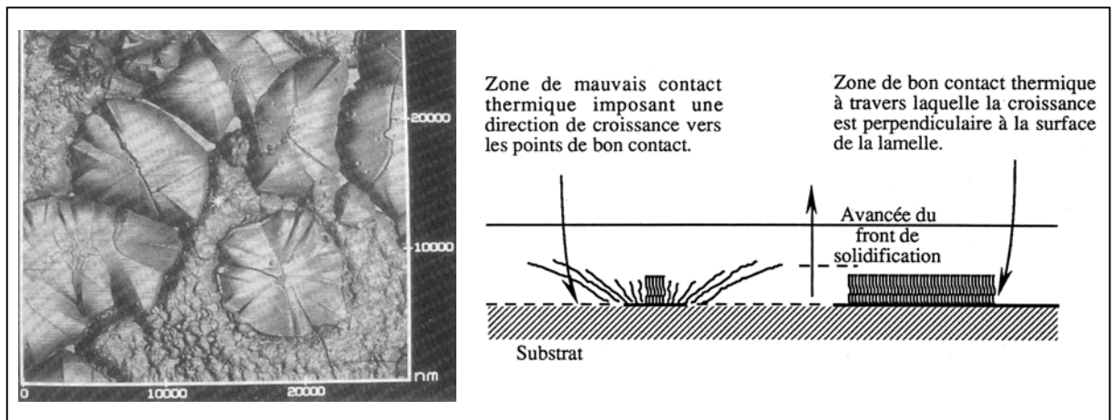
Figure I.12 : Vue AFM de la microstructure générale d'une lamelle d'alumine déposée sur un substrat en acier (à gauche) et représentation schématisée des directions de croissance cristalline dans une lamelle en fonction de la qualité du contact thermique à l'interface (à droite) [BIA 95].
