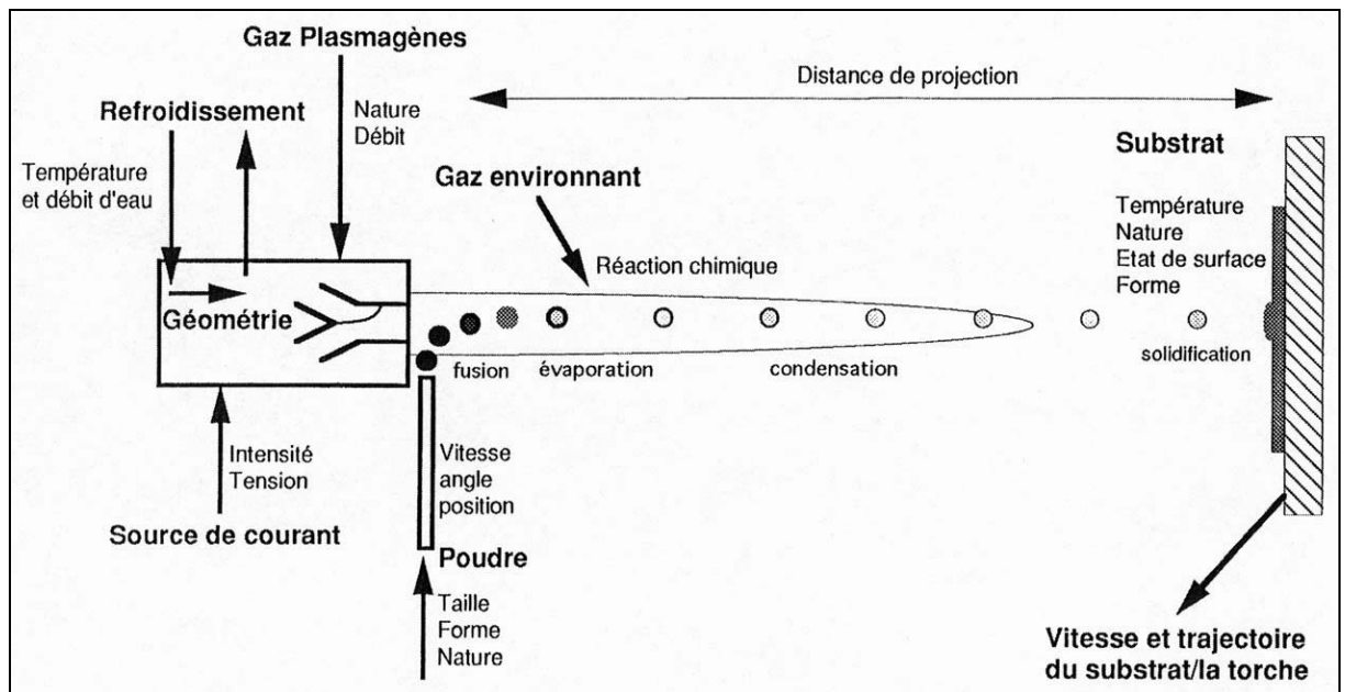
Figure I.4 : Représentation schématis des paramètres influents en projection thermique : exemple de la projection plasma [GAR 95].
