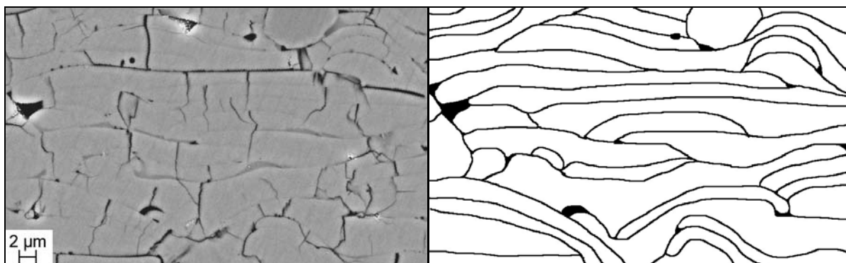
Figure III.4 : Micrographie MEB (à gauche) et schéma des frontières inter-lamellaires (à droite) de la coupe d'un dépôt (poudre \text{Al}_2\text{O}_3 [-25 +10 μm], plasma HPPS-22 kW, distance de projection de 130 mm).
