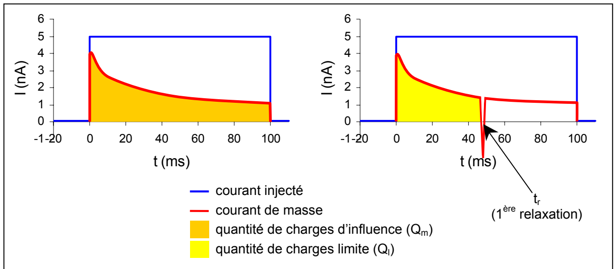
Figure II.22 : Mesures de Q_m , t_r et Q_l à partir des courbes I = f(t) .
