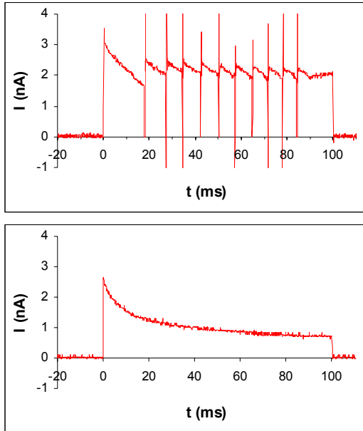
Figure IV.25 : Evolutions du courant de masse lors d'injections de 500 pC sur la surface du dépôt obtenu avec le plasma HPPS de 12,5 kW.
