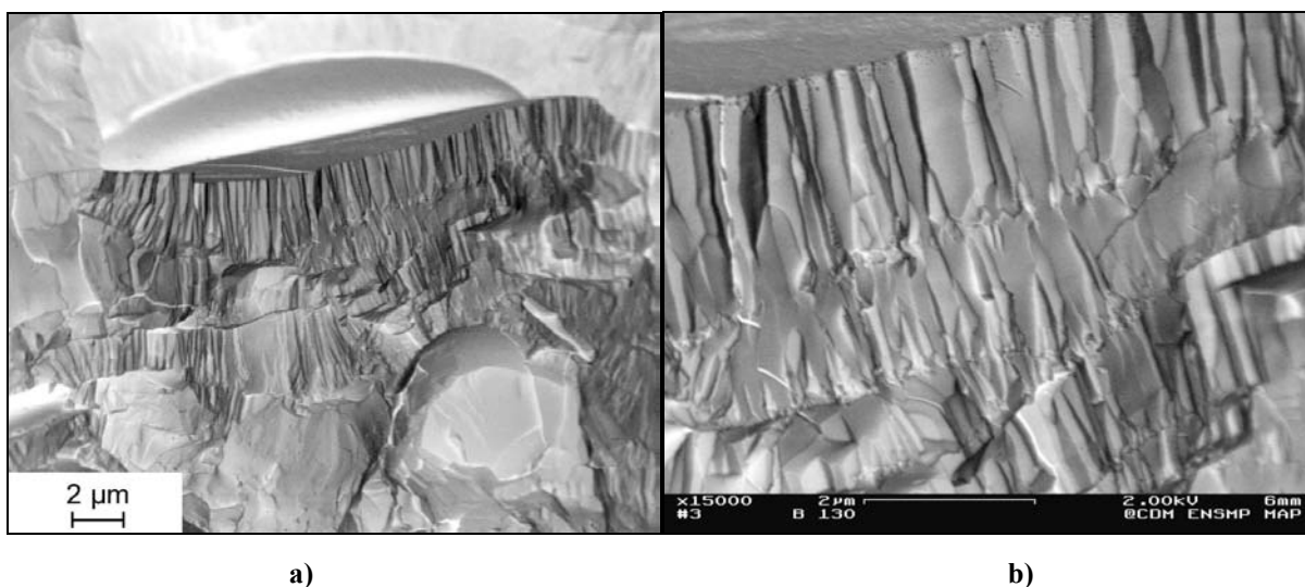
Figure III.7 : Fractographie MEB d'un dépôt (poudre \text{Al}_2\text{O}_3 [-25 +10 \mu\text{m} ], plasma HPPS-22 kW, distance de projection de 130 mm) ; (en b) : vue plus détaillée de a))
