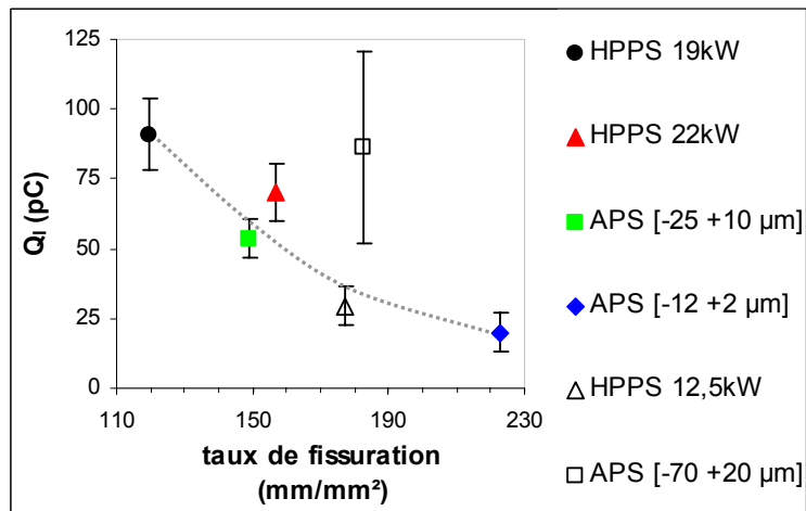
Figure IV.29 : Evolution de Q_i en fonction du taux de fissuration
