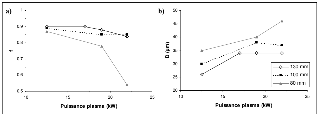
Figure V.18 : Evolution du facteur de forme f et du diamètre moyen des lamelles D en fonction de la puissance du plasma HPPS utilisé et de la distance de projection.
