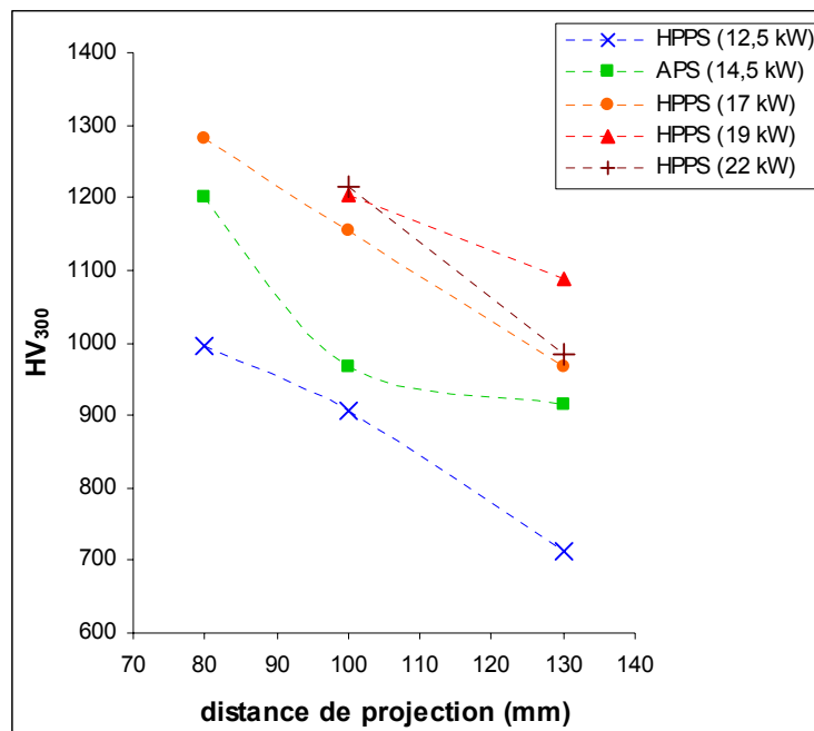
Figure III.20 : Evolution de la dureté Vickers de dépôts plasma de la poudre \text{Al}_2\text{O}_3 [-25+10 \mu\text{m} ], indents avec une masse de 300 g, en fonction du plasma et de la distance de projection utilisés.
