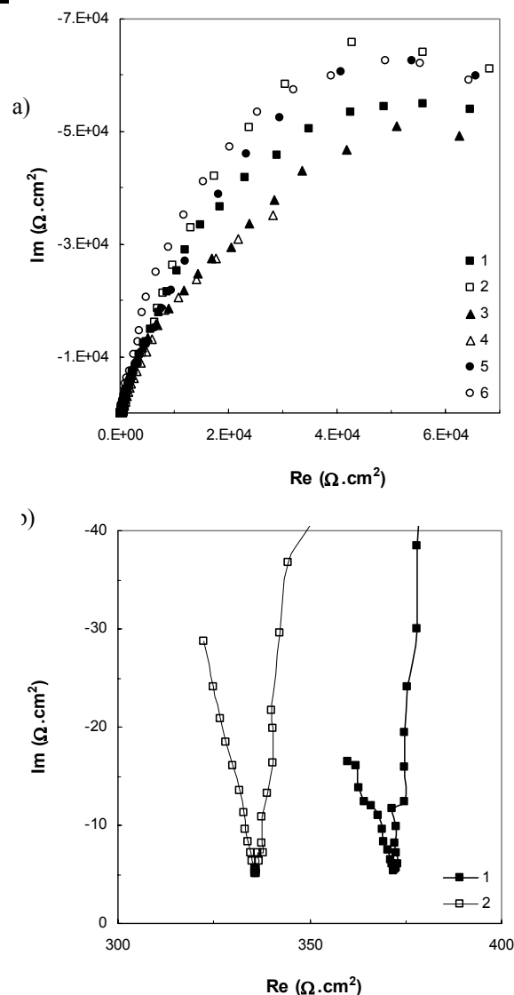
Figure IV.12 : Diagrammes de Nyquist des dépôts étudiés après immersion dans une solution de NaCl (3%) : a) courbes de 65 kHz à 10 mHz, b) exemples de début de courbes (cas 1 et 2) : de 65 kHz à environ 100 Hz.
