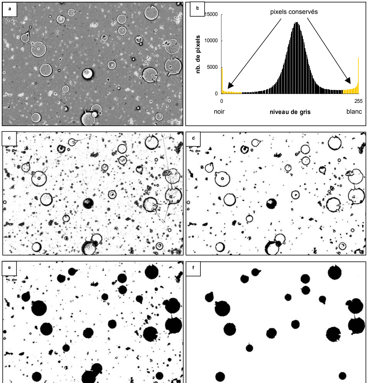
Figure II.8 : Processus d'analyse d'images des lamelles étalées (a : image MEB ; b : histogramme des niveaux de gris ; c : image seuillée ; d : image débruitée ; e : image avec les surfaces fermées remplies ; f : image finale) (poudre \text{Al}_2\text{O}_3 [-25 +10 \mu\text{m} ], plasma APS-14,5 kW, 130 mm).
