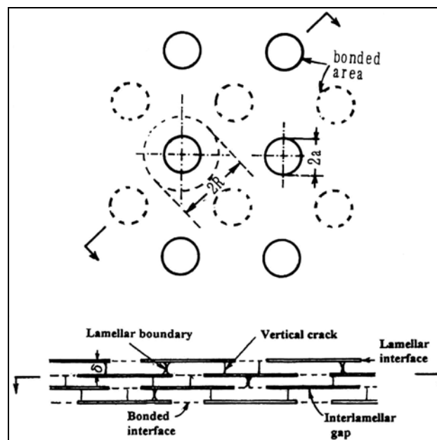
Figure I.23 : Modélisation de la microstructure d'un dépôt plasma où les lamelles sont des cylindres de rayon R et hauteur \delta en contact les uns avec les autres au travers d'une zone centrale de contact (« bonded area ») de rayon a [(vue du dessus (en haut) et vue en coupe (en bas))] ([LI 02]).
