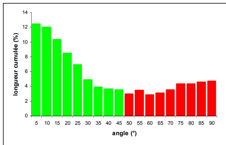
Figure II.15 : Répartition angulaire des fissures du dépôt plasma correspondant à l'image de la Figure II.12a (poudre \text{Al}_2\text{O}_3 [-25 +10 \mu\text{m} ], plasma HPPS-17 kW, 130 mm).
