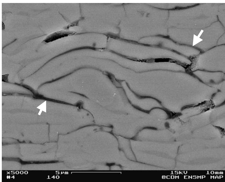
Figure III.16 : Micrographie MEB de la coupe d'un dépôt (poudre \text{Al}_2\text{O}_3 [-12 +2 μm] projeté à 130 mm et en mode APS) révélant notamment le décollement inter-lamellaire.
