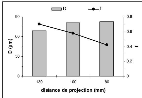
Figure V.17 : Evolution du diamètre moyen D et facteur de forme moyen f des lamelles de la poudre \text{Al}_2\text{O}_3[-70 +20 \mu\text{m}] projetée en mode APS.
