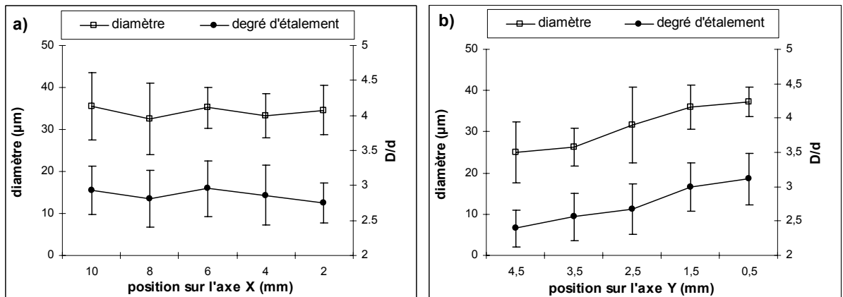
Figure V.3 : Evolution du diamètre et du degré d'étalement D/d des lamelles de la périphérie vers le centre de la tâche de poudre, le long des axes X et Y définis dans la Figure V.1.
