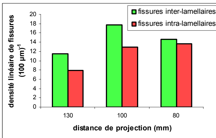
Figure III.17 : Evolution des taux de fissurations des dépôts de poudre intermédiaire \text{Al}_2\text{O}_3[-25 +10 \mu\text{m}] en mode APS en fonction des distances de projections.
