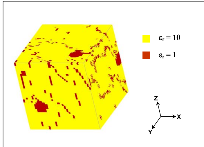
Figure V.45 : Répartition des permittivités relatives dans le cube maillé.
