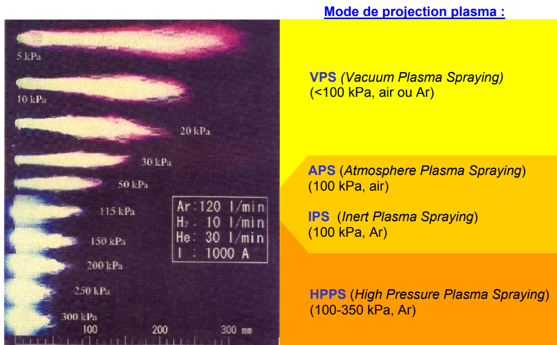
Figure I.8 : Evolution du plasma en fonction de la pression dans l'enceinte de projection ([SOD 96])
