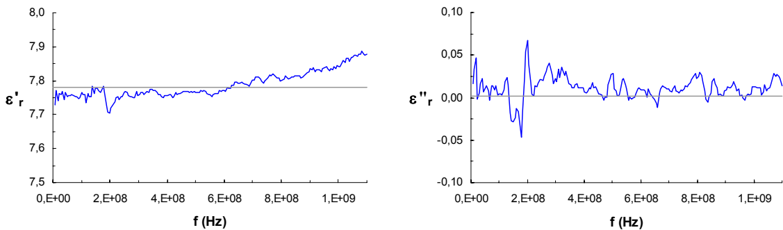
Figure IV.6 : Evolution des parties réelle et imaginaire de la permittivité complexe d'un dépôt d'alumine \text{Al}_2\text{O}_3 [-25 +10 µm] projetée en mode APS.
