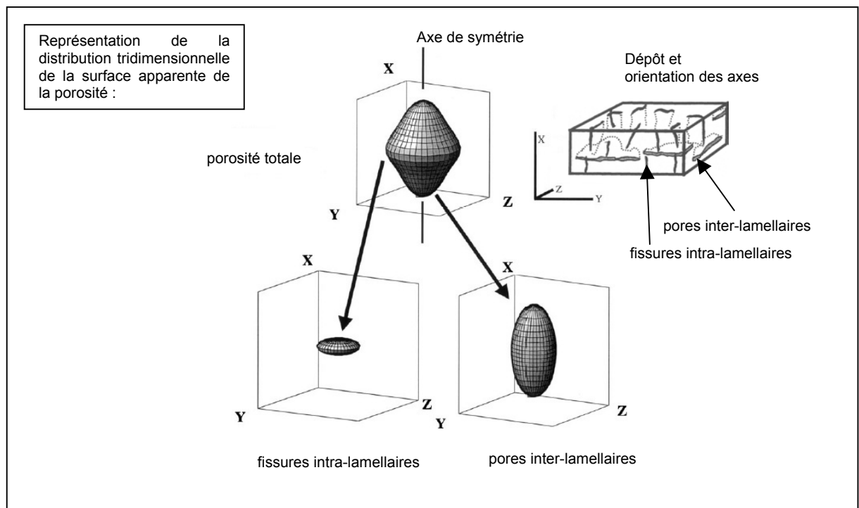
Figure I.22 : Représentation tridimensionnelle de la surface apparente de la porosité (au centre) qui peut être divisée en deux parties : celle provenant des fissures intra-lamellaires (à gauche) et celle provenant des pores inter-lamellaires (à droite) (Rq. : dépôt de ZrO_2-Y_2O_3 par projection plasma APS ; la graduation 0 se trouve au centre de chaque axe ; ces axes n'ont pas tous la même échelle) (d'après [ILA 99] et [HER 00]).
