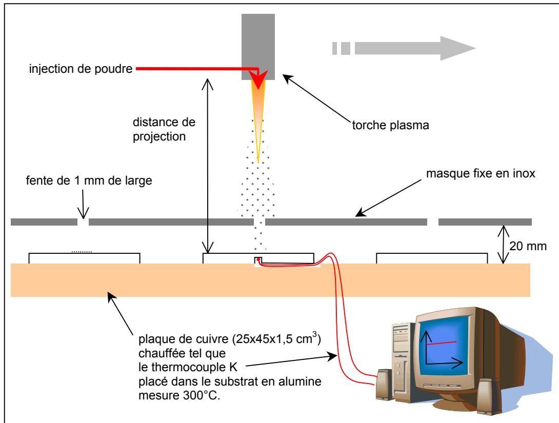
Figure II.5 : Schéma du montage utilisé pour l'obtention de lamelles individuelles d'alumine étalées sur des substrats en alumine polis et chauffés à 300°C (les échelles ne sont respectées).
