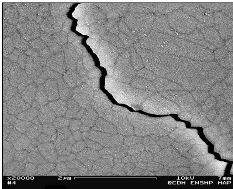
Figure III.6 : Micrographie MEB d'une fissure visible à la surface d'une lamelle (poudre d'alumine \text{Al}_2\text{O}_3 [-25 +10 \mu\text{m} ], plasma HPPS-22 kW, distance de projection de 130 mm).
