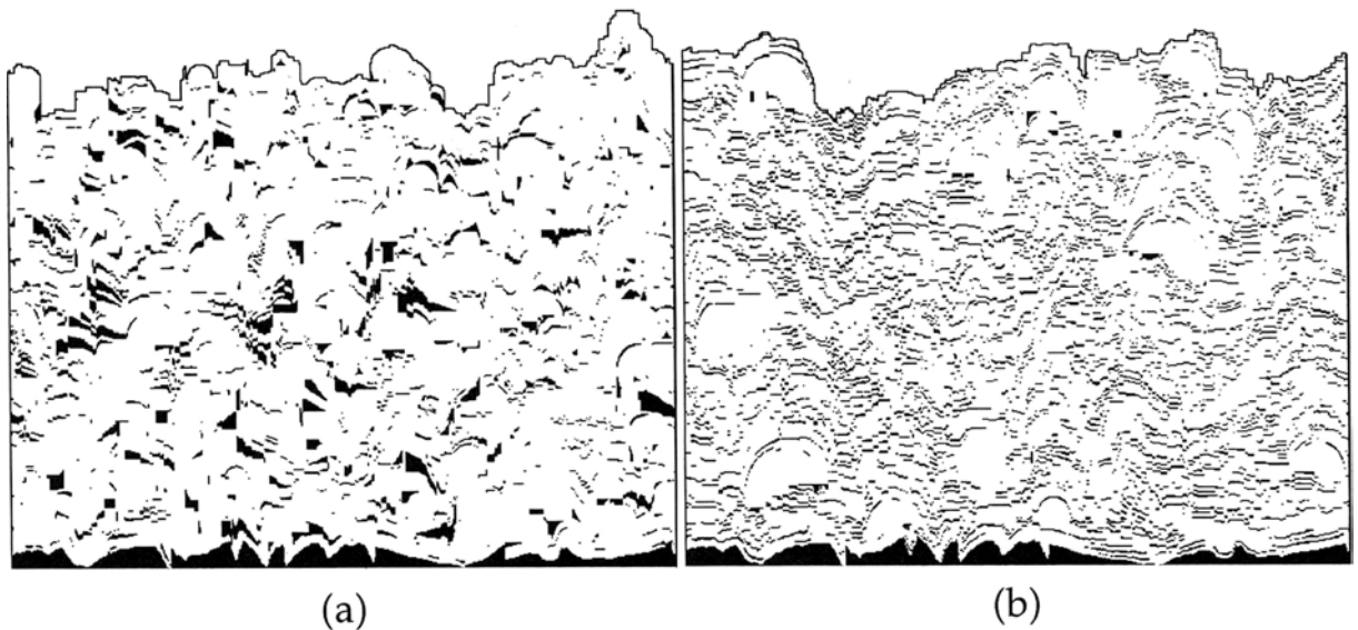
Figure I.25 : Simulation bidimensionnelle d'un dépôt plasma par empilement de lamelles ayant un paramètre de contact f (a) aléatoire (b) égal à 0,2 ( f = diamètre de la zone de contact / diamètre de la lamelle) [HAR 95]
