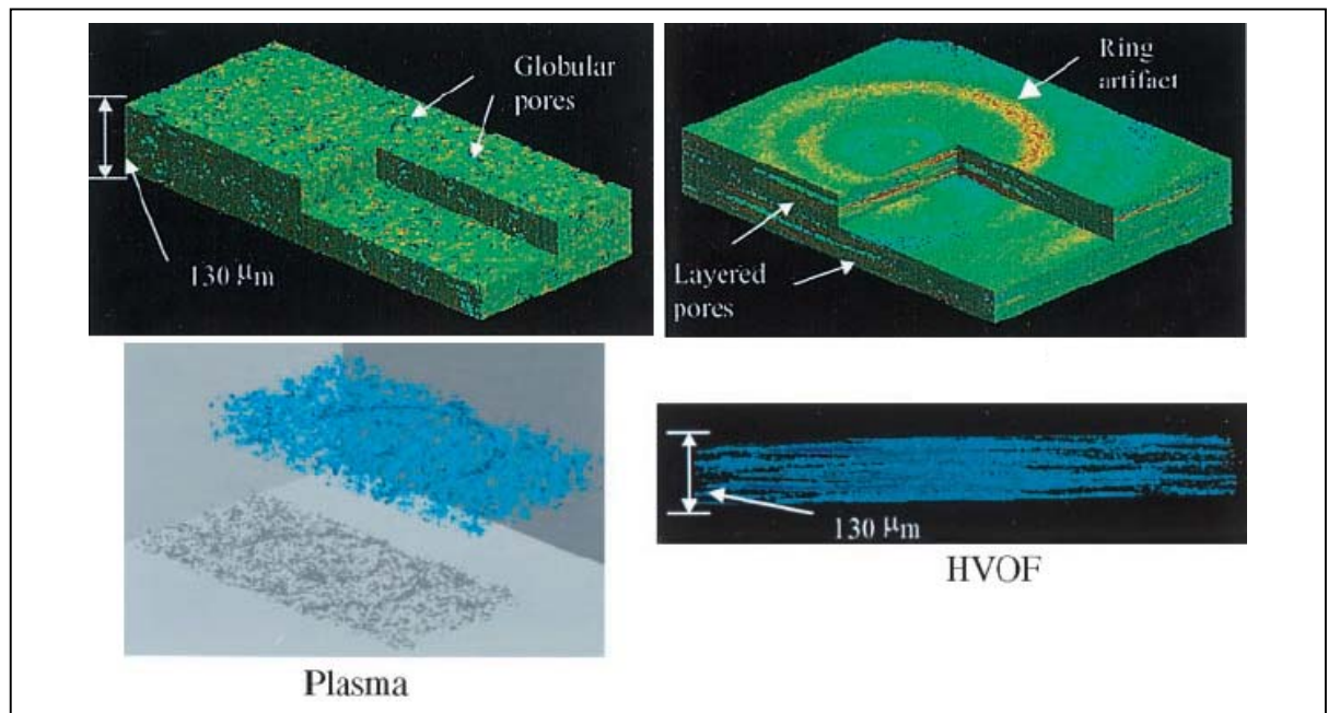
Figure I.21 : Utilisation de la microtomographie pour observer un dépôt APS d'alumine [-50 +15 μm] (images de gauche) et un dépôt HVOF d'alumine [-22 +5 μm] (images de droite) ; visualisations tridimensionnelles des dépôts (images du haut) et de leur porosité (images du bas) [KUL 00].
