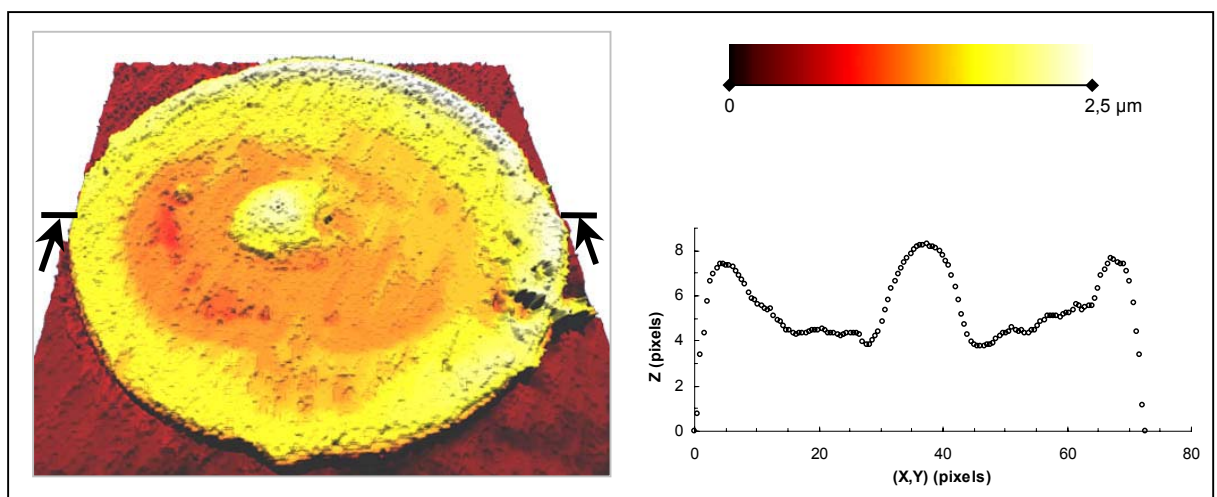
Figure V.25 : Image et profil utilisé pour la simulation, de la lamelle de la Figure V.9, obtenue par microscopie confocale, (poudre \text{Al}_2\text{O}_3 [-25 +10 μm] projetée en mode APS).
