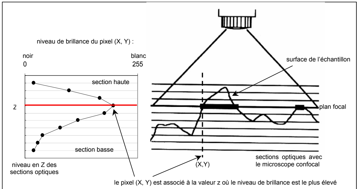
Figure II.10 : Principe de la construction d'une image topographique à l'aide d'un microscope confocal, d'après [LAN 93].
