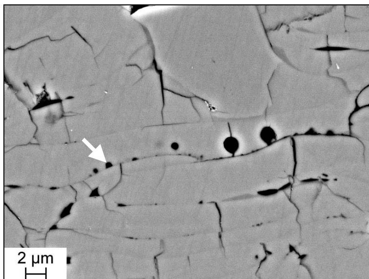
Figure III.3 : Micrographie MEB de la coupe d'un dépôt (poudre \text{Al}_2\text{O}_3 [-25 +10 \mu\text{m} ], plasma HPPS-22kW, distance de projection de 130 mm) révélant des bulles submicroniques aux interfaces inter-lamellaires.
