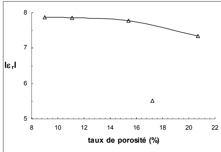
Figure IV.7 : Evolution de la permittivité \epsilon_r des dépôts en fonction du taux de porosité.
