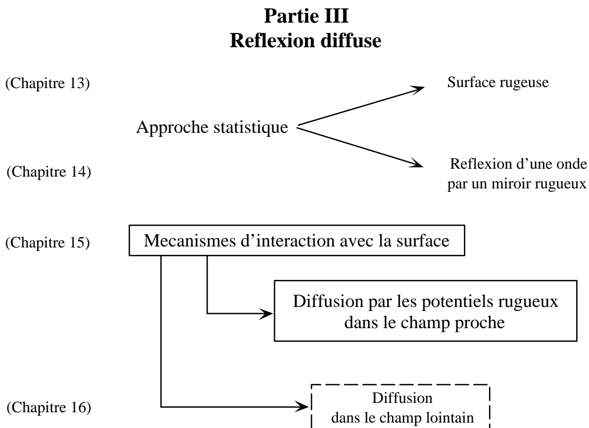
Figure 3: Organigramme de la partie III : réflexion diffuse.
