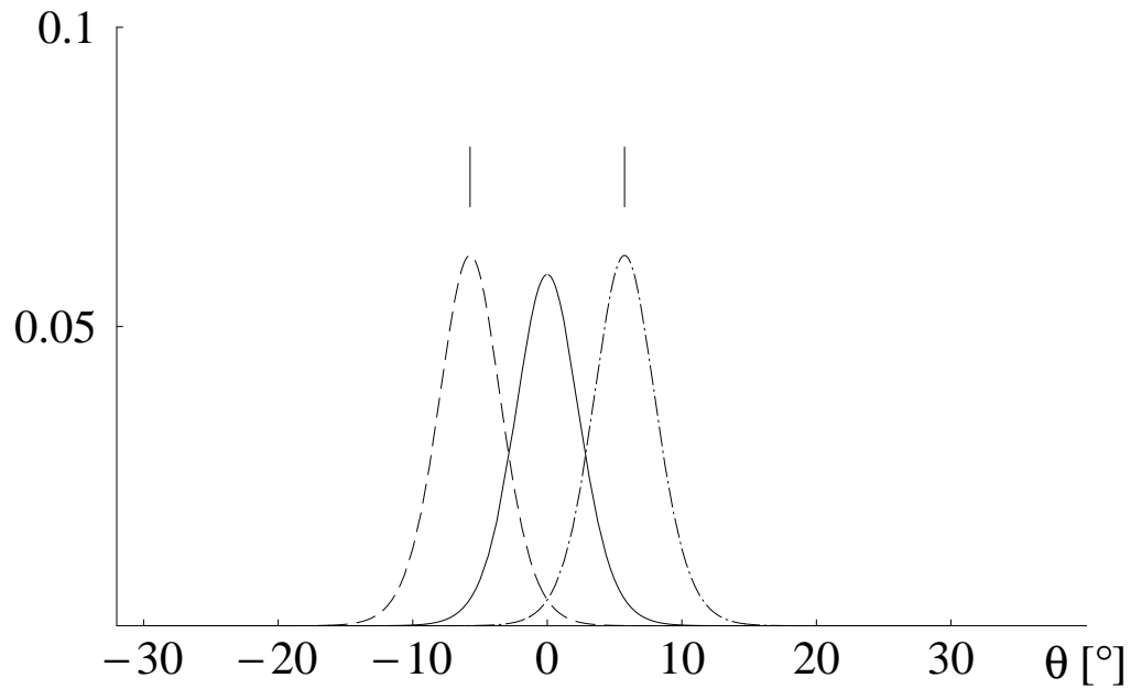
Figure 8.12: Populations w_{\pm 1} en fonction de l'angle d'incidence, dans le régime de BRAGG. Les traits verticaux marquent les angles de résonance \theta_B \approx \pm 5.^\circ 7 .
