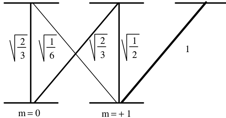
Figure 15.10: Coefficients de CLEBSCH-GORDON pour une transition J = 1 \rightarrow J_e = 2 . A cause de la symétrie des coefficients par rapport à m = 0 , seuls ceux avec m \geq 0 sont représentés.
