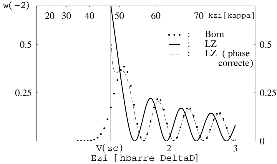
Figure 11.23: Résultat (11.32) pour la population de l'ordre de diffraction \nu = -2 dans l'approximation de BORN, en fonction de l'énergie incidente E_{zi} (en unités de l'énergie DOPPLER \hbar\Delta_D ). A comparer à la figure 11.21.
