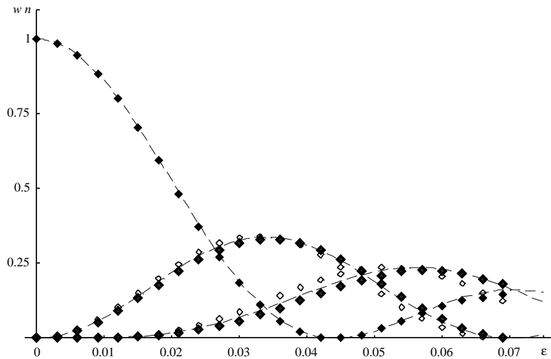
Figure 8.22: Identique à la figure 8.21, mais en incidence oblique \theta_i = 45^\circ . Les losanges pleins (creux) représentent les résultats de l'approche BKW pour les ordres positifs (négatifs). Les courbes en tirets donnent les résultats de l'approximation du réseau de phase mince (8.62) (identiques pour les ordres n et -n ). La composante normale du vecteur d'onde incident vaut encore k_{zi} = 200 \kappa .
