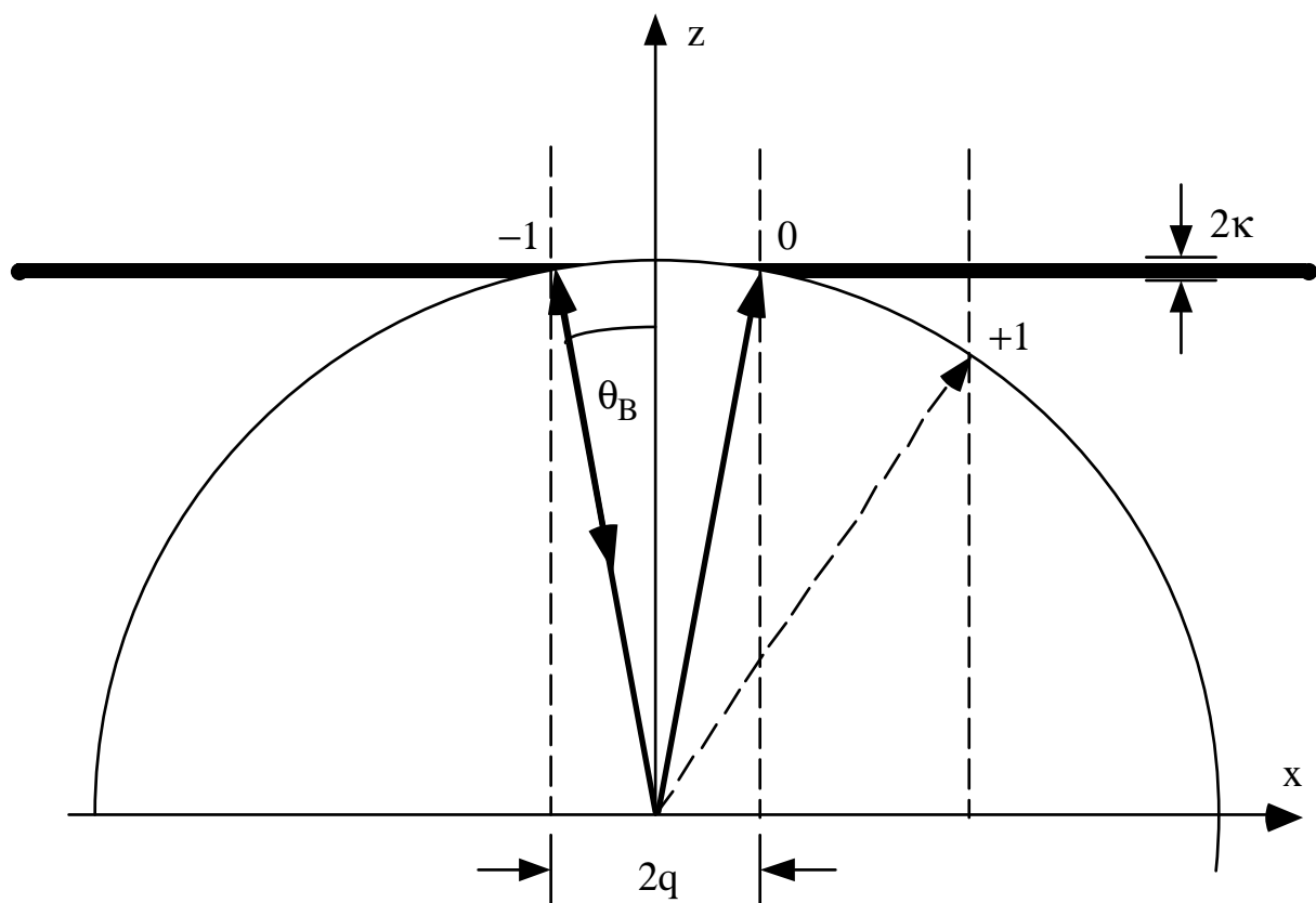
Figure 7.15: Diffraction d'atomes dans le régime de BRAGG. Géométrie de LITROW pour l'ordre n = -1 .
