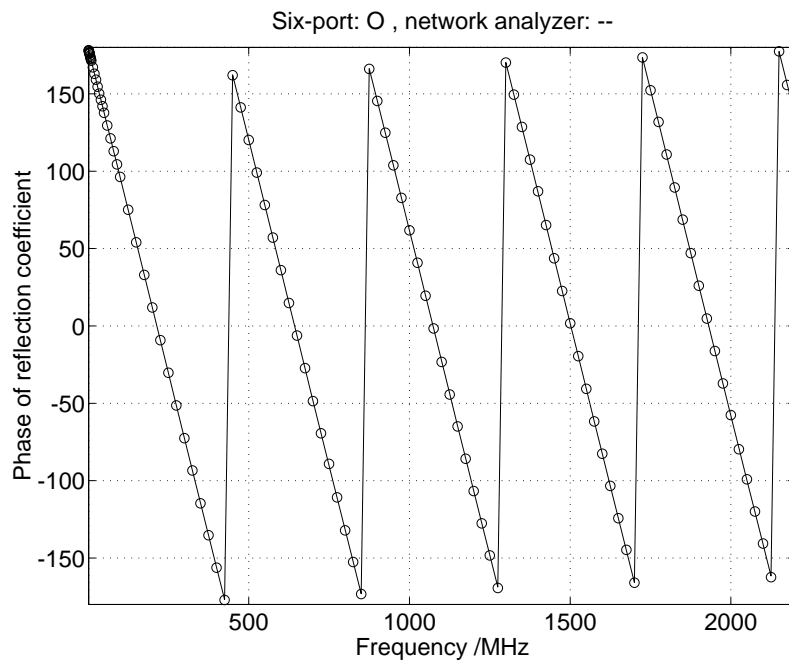
FIG. 6.27 – La phase du facteur de réflexion d'une charge (ligne \approx 20 cm et court-circuit) mesurée avec le réflectomètre 3 et le HP 8753C
