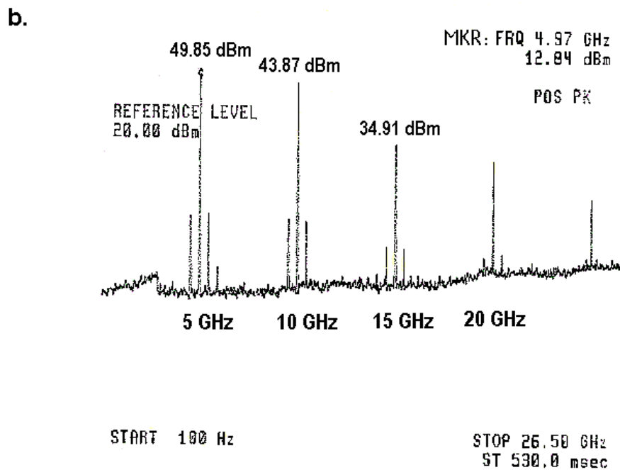
FIG. 5.5 – Spectres en sortie du tube pour la saturation à 5 GHz seule (a) et pour la configuration la plus favorable d'injection de 10 GHz en plus de 5 GHz (b). Les valeurs portées à côté de chaque raie sont celles lues sur les bolomètres.
