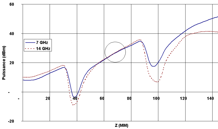
FIG. 4.12 – Puissances de sortie sur fondamentale et sur harmonique en fonction de la distance pour le tube TH2 : P_{e1} = 12 dBm, P_{e2} = 10 dBm, \Phi_1 = 0 et \Phi_2 = 5.28 rad.
