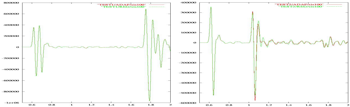
FIG. 8.10: Solution pour le maillage adapté (en rouge) et le maillage non-adapté (en vert), dans le cas où c_1 = c_2 (à gauche) et c_1 \neq c_2 (à droite).
