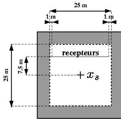
FIG. 10.1: Domaine d'étude pour la validation
