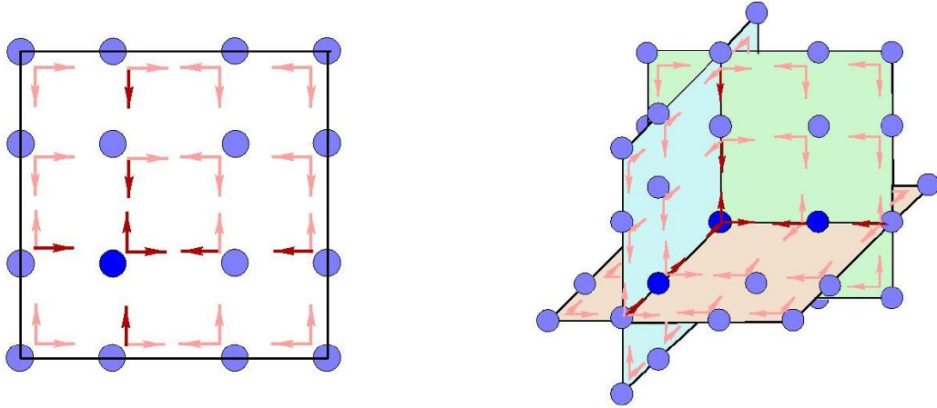
FIG. 1.7: Interactions non-nulles de la matrice de rigidité pour r = 3 en 2D (à gauche) et 3D (à droite).
