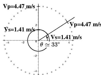
FIG. 10.6: Vitesses de groupe associées au milieu isotrope.
