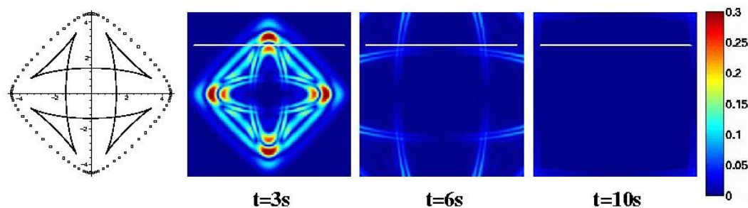
FIG. 10.4: Fronts d'ondes théoriques (à gauche) et module du champ de déplacement, à différents instants, obtenus par EFMS (à droite) pour le troisième matériau.
